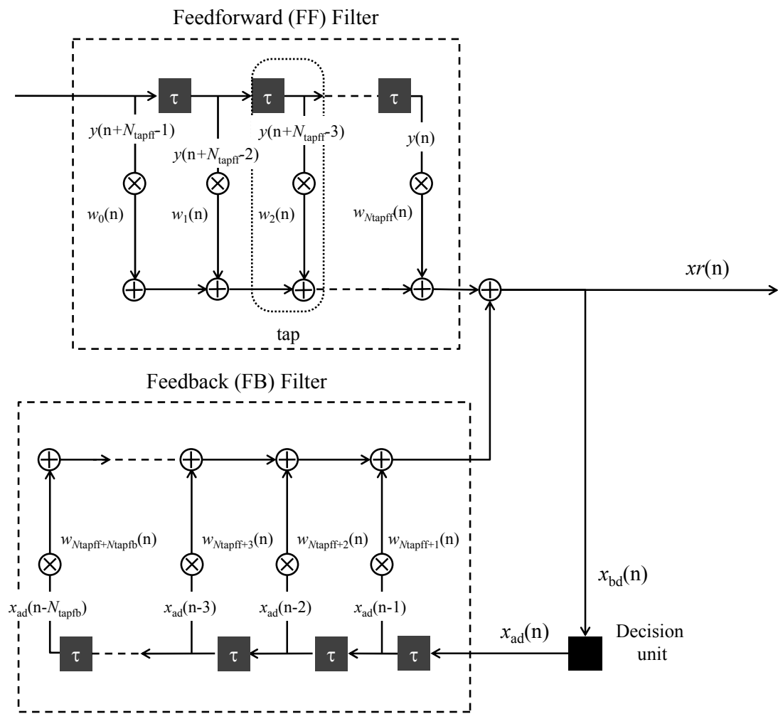
図 2.4 DFE の構成
