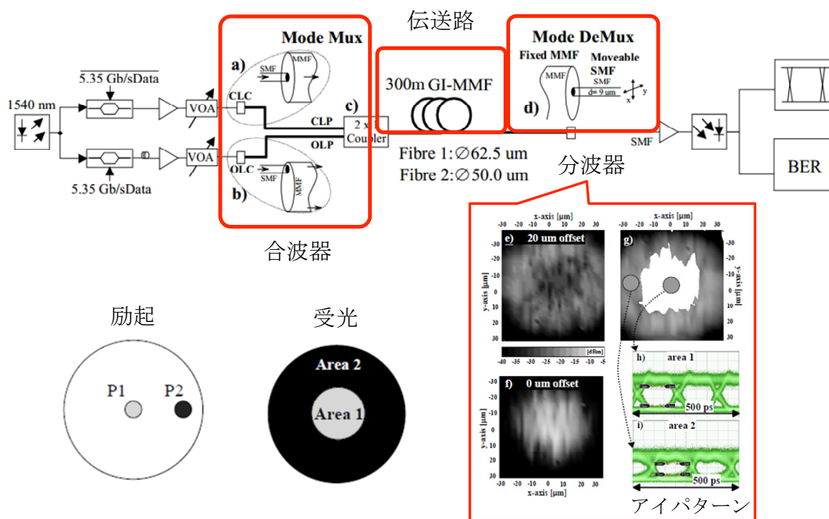
図 1.4 励起・受光位置の調整によるモード合分波 ([1.21]を参考に編集)
