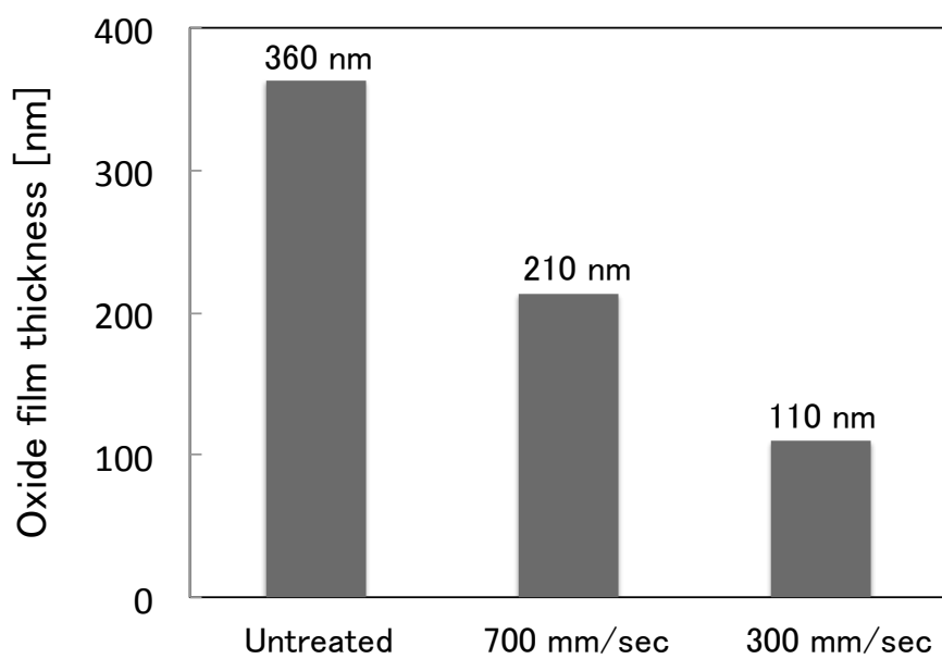
図 4-26 プラズマ処理前後での酸化膜厚変化
