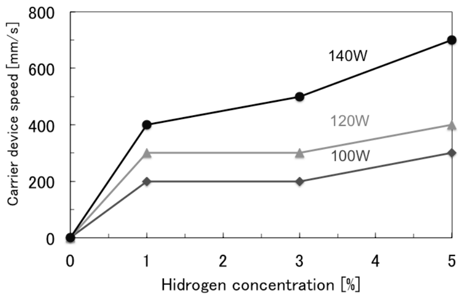
図 4-23 各プラズマ生成条件における酸化膜除去速度
