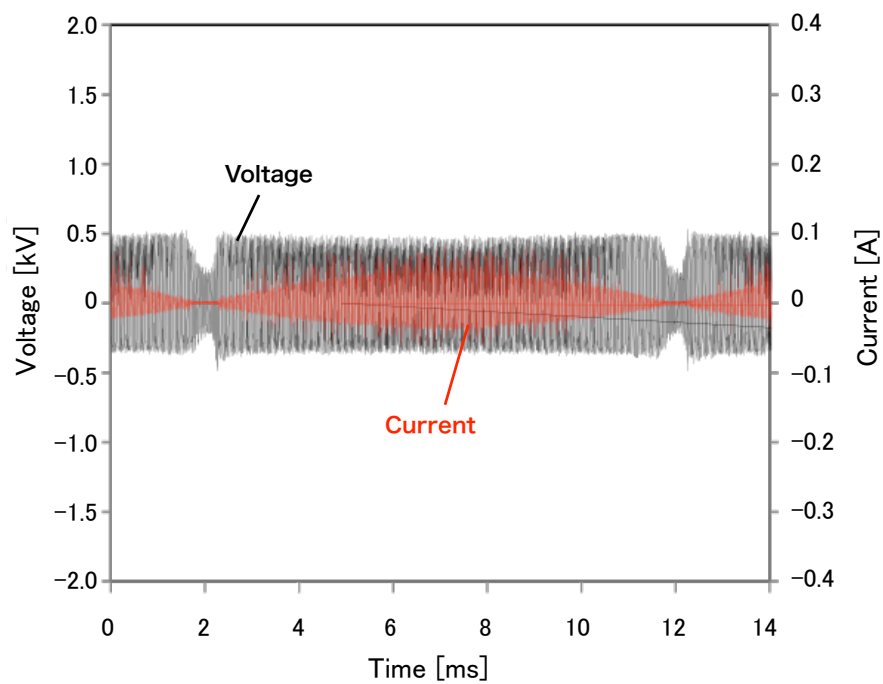
図 3-10 ヘリウムプラズマ生成時の電圧及び電流波形
