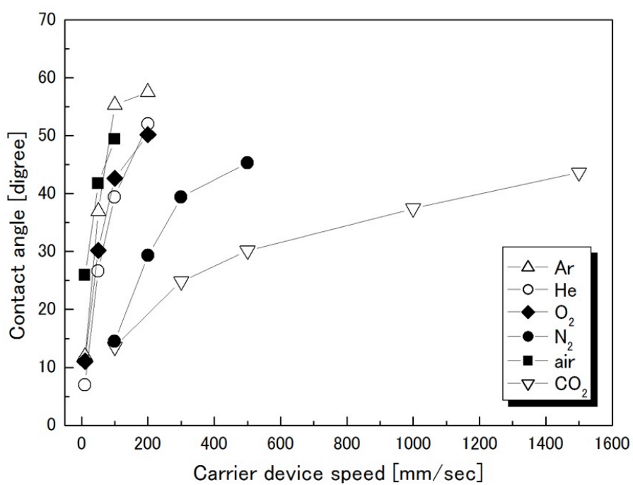
図 4-3 各ガス種のプラズマによる親水化効果
