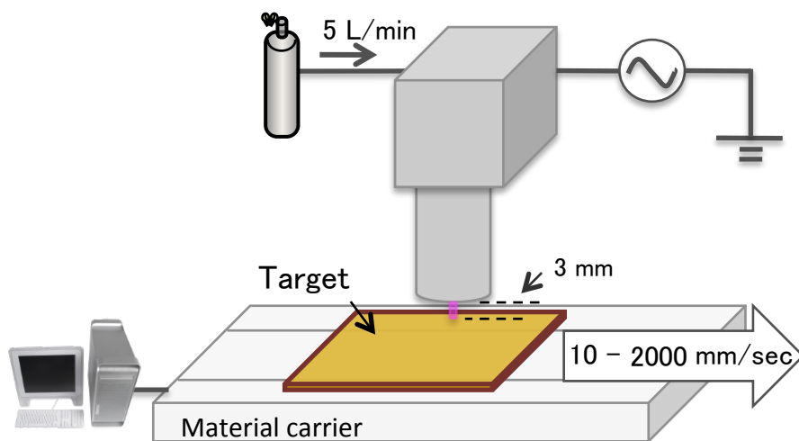
図 4-2 実験装置構成
