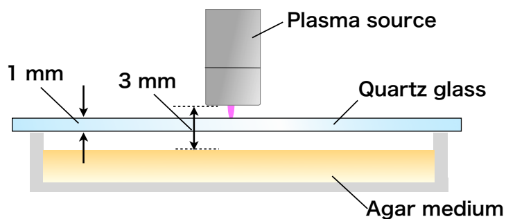
図 5-3 プラズマから発せられる紫外線による影響調査のセットアップ
