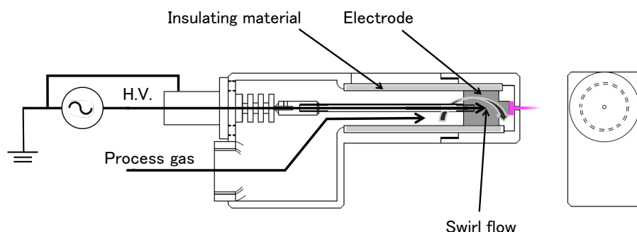
図 3-2 マルチガスプラズマジェットの内部構造
