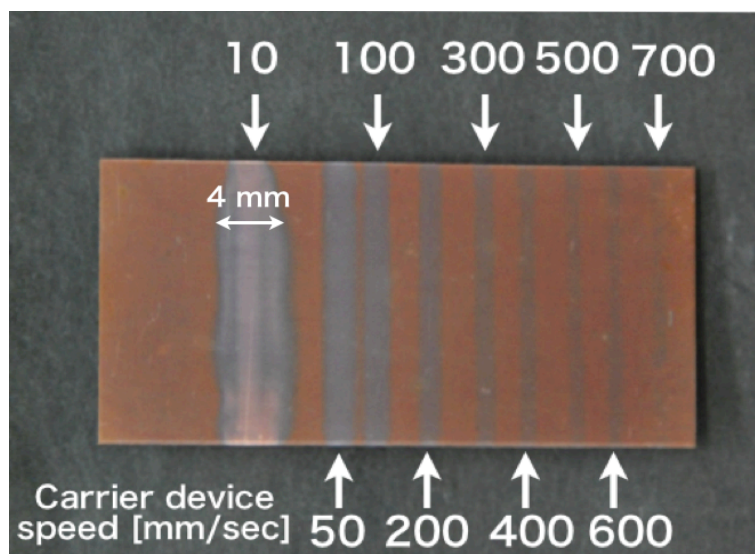
図 4-24.最適条件での酸化膜除去(照射距離 1 mm, アルゴンガス 10 L/min, 水素添加濃度 5%, 入力電力 140 W)
