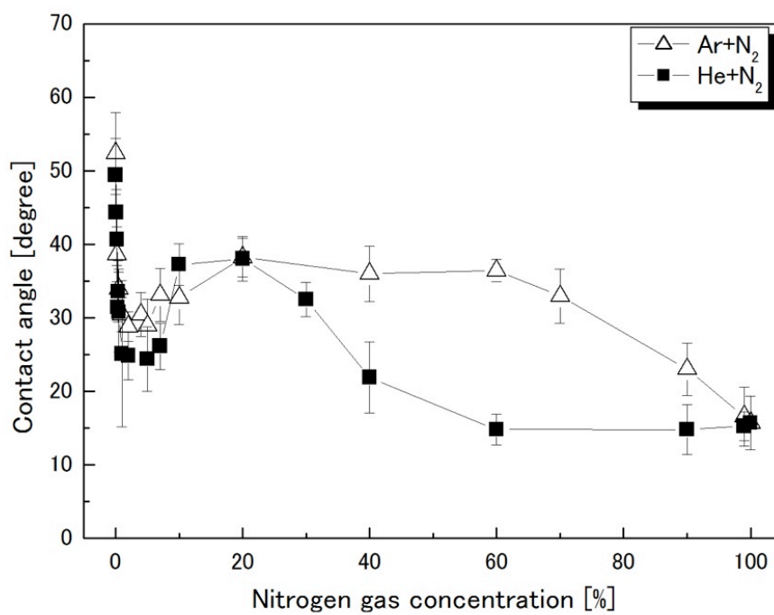
図 4-6 アルゴン窒素及びヘリウム窒素プラズマの親水化効果の混合率依存性
