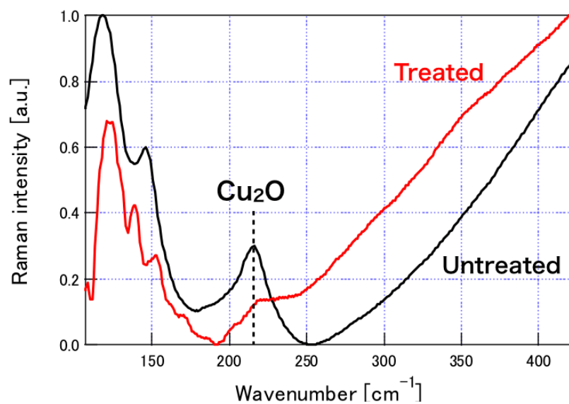
図 4-22 プラズマ処理前後での Cu 2 O ラマンスペクトル変化(照射距離 1 mm, アルゴンガス 10 slm, 水素添加濃度 3%, 入力電力 100 W, 搬送速度 10 mm/s)
