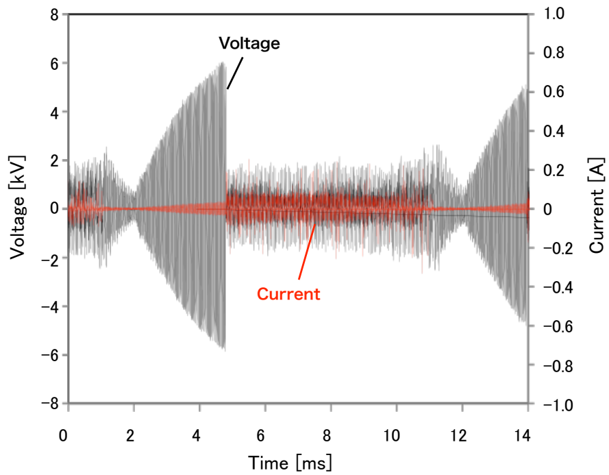
図 3-12 空気プラズマ生成時の電圧及び電流波形
