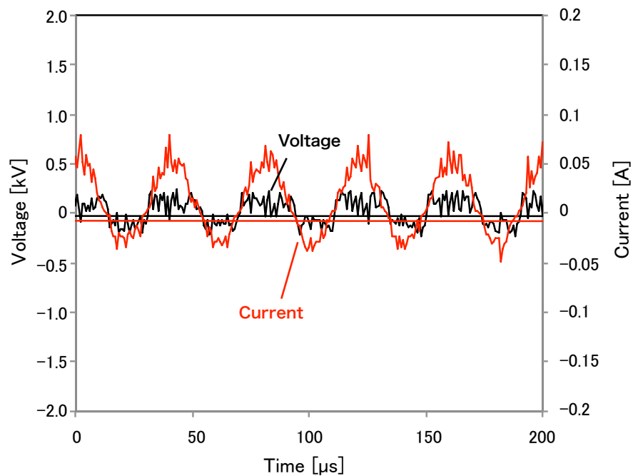
図 3-9 アルゴンプラズマの放電部の電圧及び電流波形
