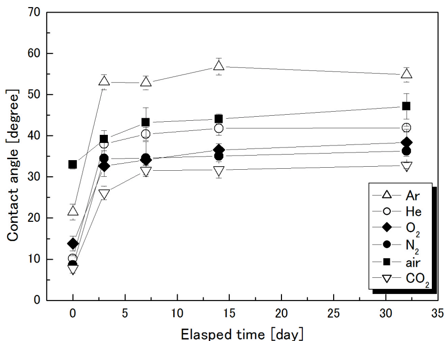
図 4-8 各ガス種のプラズマ処理後の親水化効果の経時変化
