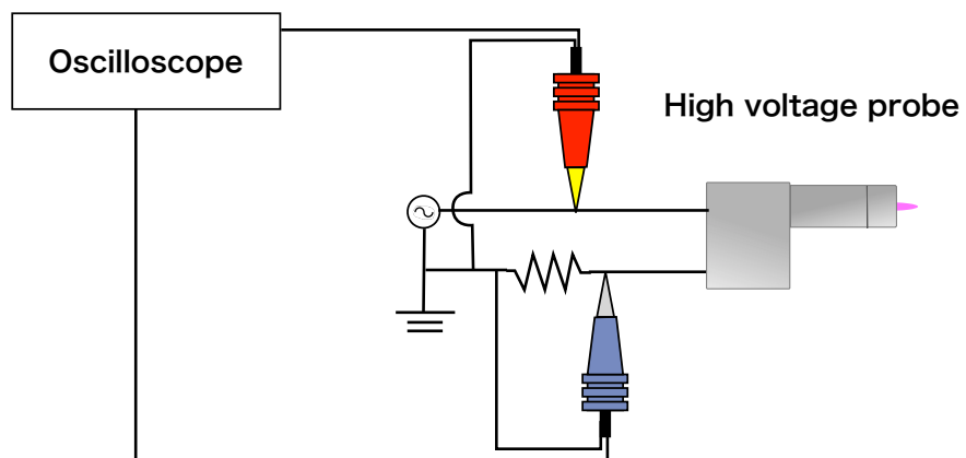
図 3-6 プラズマ生成時の電圧および電流測定
