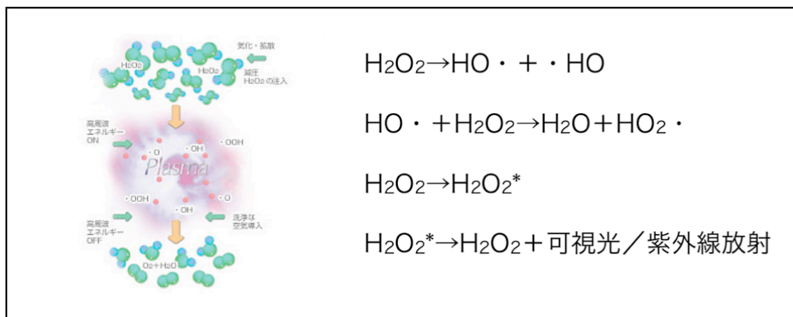
図 2-3 ステラッド®の動作原理
