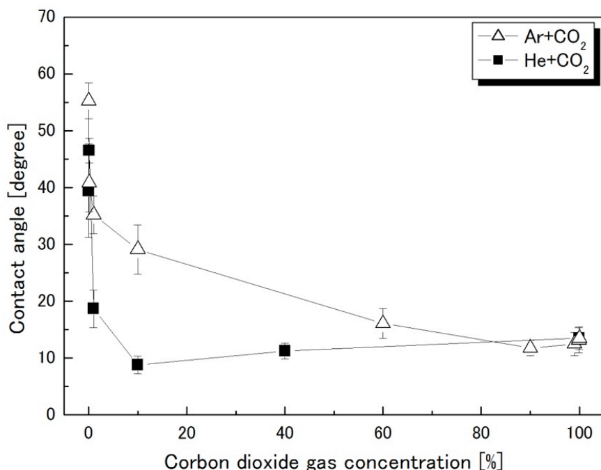
図 4-7 アルゴン二酸化炭素及びヘリウム二酸化炭素プラズマの親水化効果の混合率依存性
