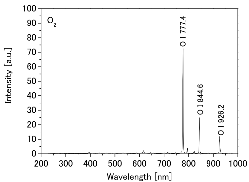
図 7-7 酸素プラズマの発光スペクトル
