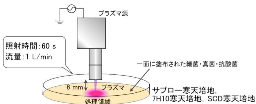
図 5-7 寒天培地上の細菌・真菌に対するプラズマの照射
