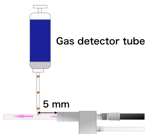
図 7-10 ガス濃度測定の設定アップ
