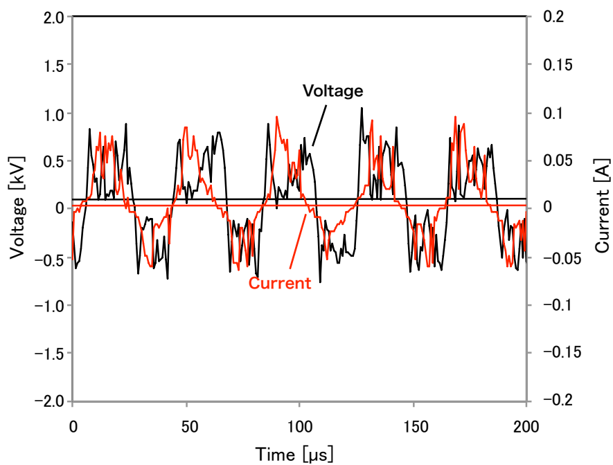
図 3-15 窒素プラズマの放電部の電圧及び電流波形
