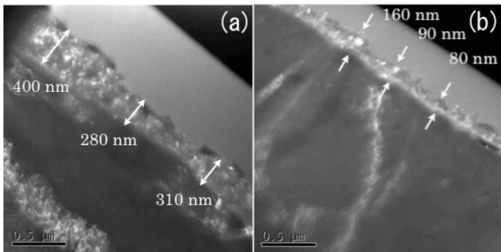
図 4-25. (a)プラズマ処理前の銅酸化膜層(b)搬送速度 300 mm/sec でプラズマ処理した後の銅酸化膜層
