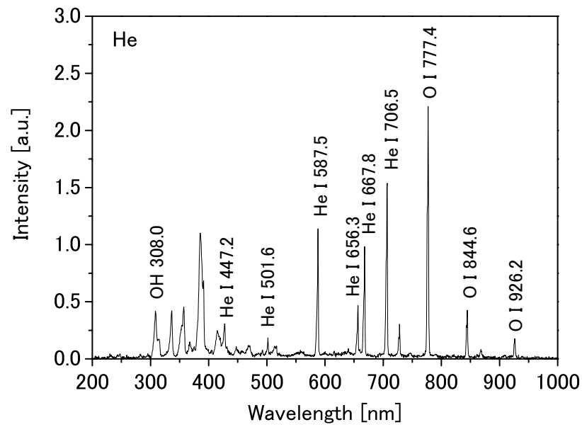
図 7-4 ヘリウムプラズマの発光スペクトル
