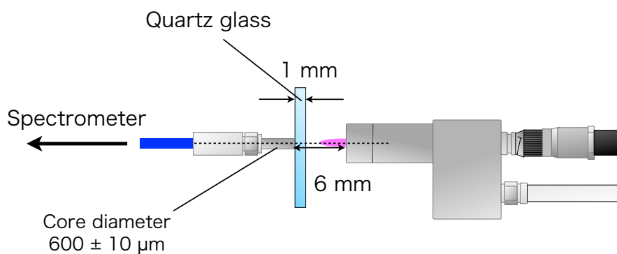
図 7-2 発光分光のセットアップ
