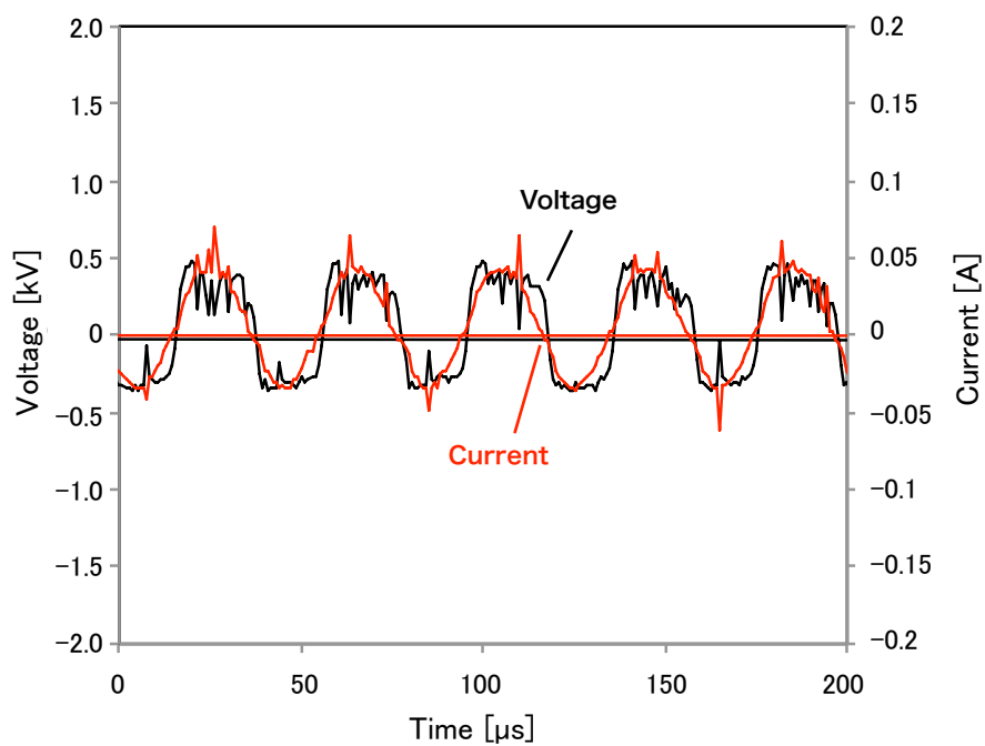
図 3-11 ヘリウムプラズマ放電部の電圧及び電流波形
