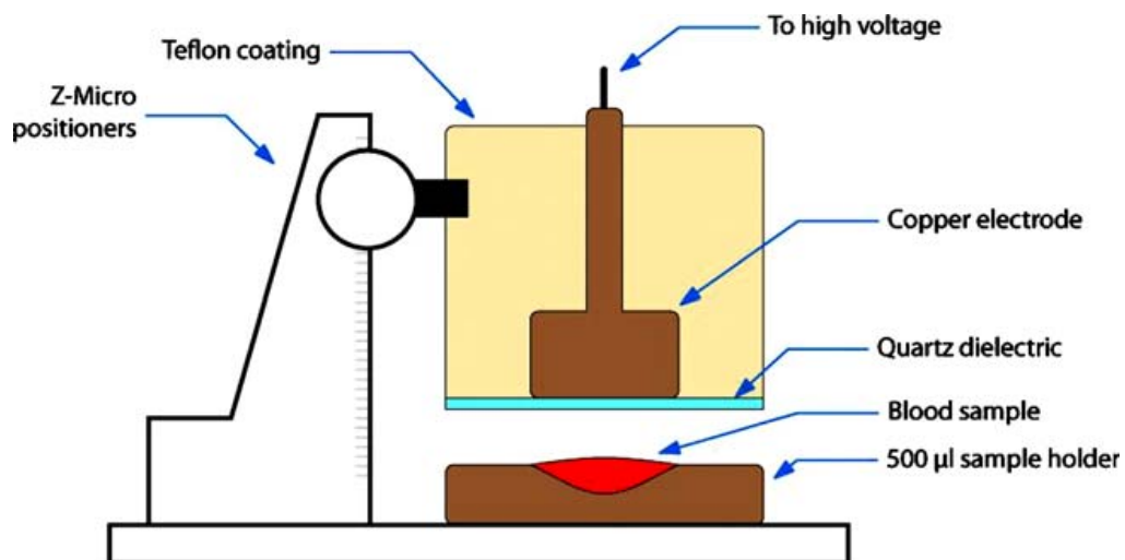
図 2-6 浮遊電極型誘電体バリア放電装置
