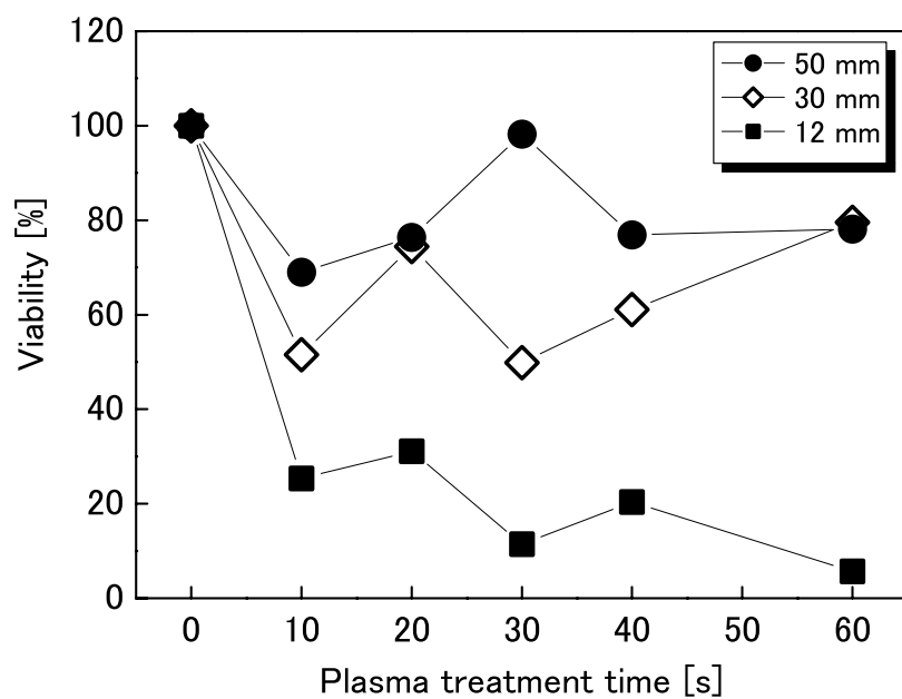
図 6-12 照射距離と CO 2 プラズマによる生存率の関係
