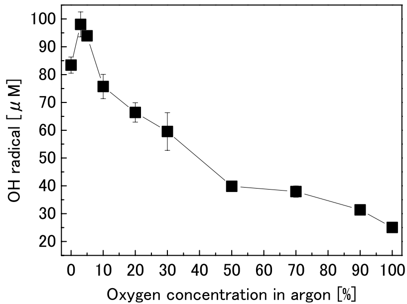
図 7-32 各 Ar/O 2 混合プラズマの OH ラジカル量
