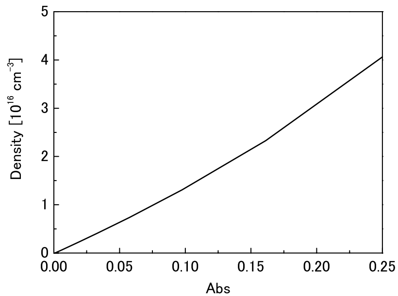
図 7-16 酸素原子の吸光度と密度の関係
