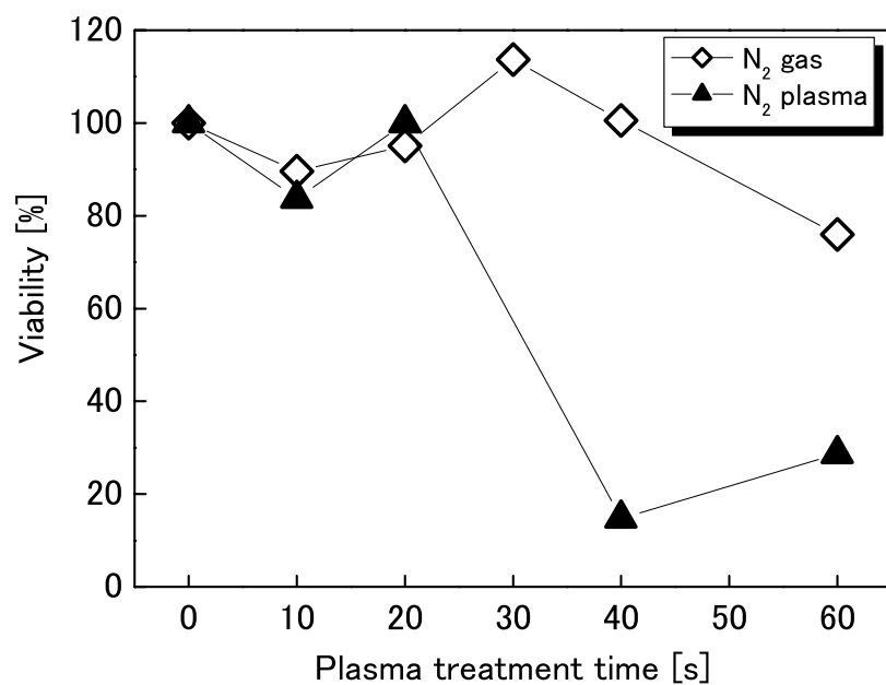
図 6-8 窒素ガス及びプラズマによる HeLa 細胞の生存率の変化
