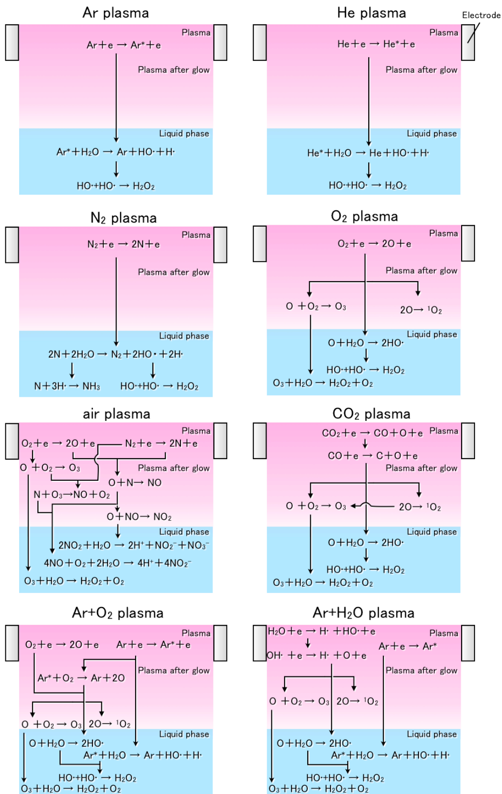
図 7-45 各活性種の生成過程
