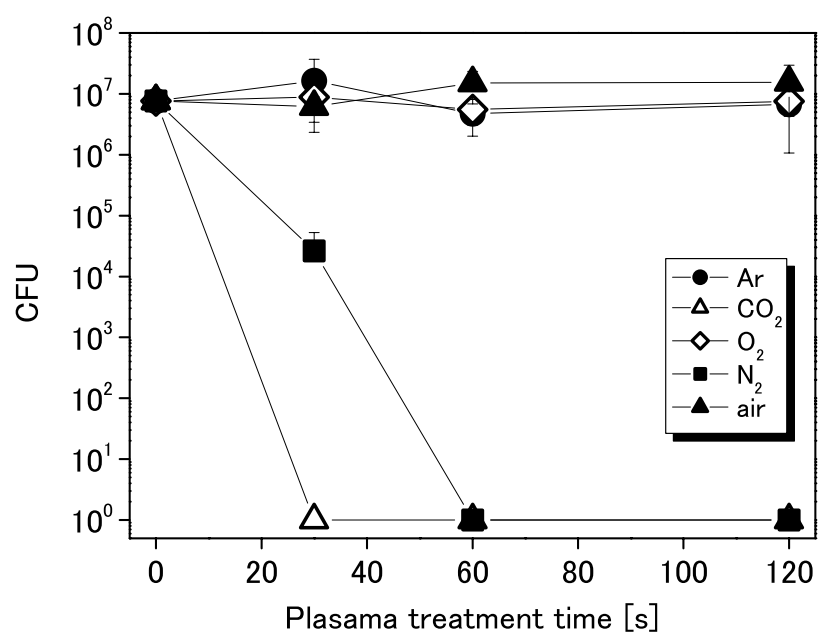
図 5-10 黄色ブドウ球菌に対する殺菌効果
