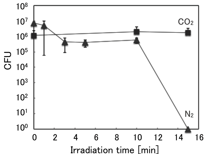
図 5-23 芽胞形成菌(セレウス菌)に対する殺菌効果
