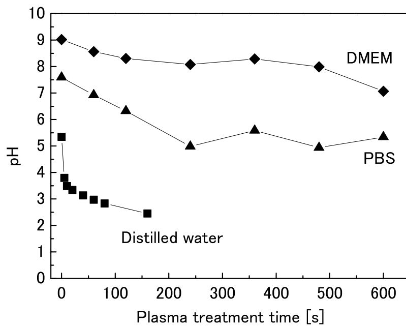
図 3-25 空気プラズマによる各種溶液の pH 変化
