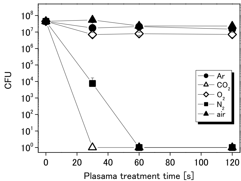
図 5-12 大腸菌に対する殺菌効果
