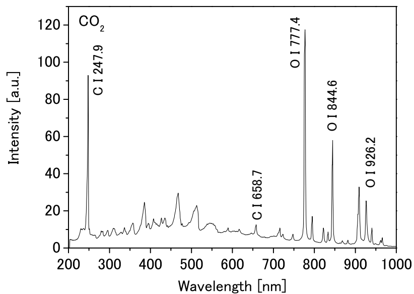
図 7-8 二酸化炭素プラズマの発光スペクトル
