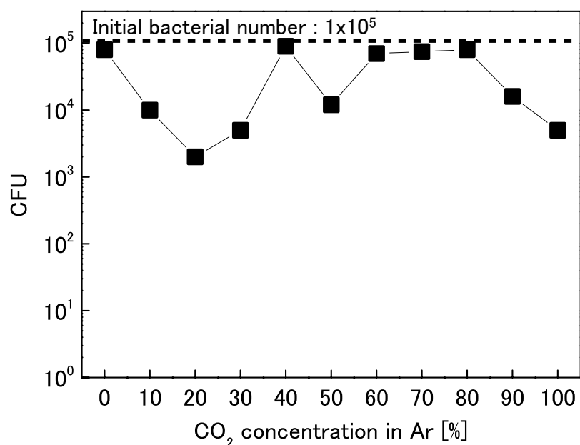
図 5-38 B. subtilis の殺菌に対するアルゴン二酸化炭素プラズマの混合比依存性
