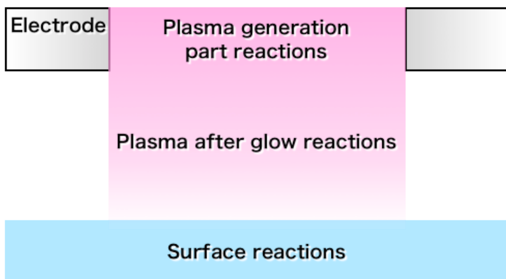
図 7-1 各活性種が生成されるエリア
