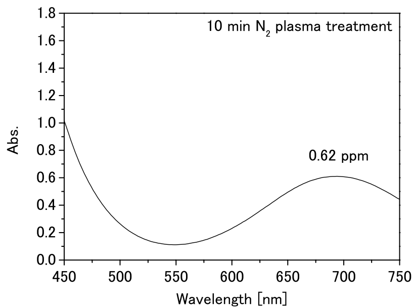
図 7-44 10 分間の窒素プラズマ処理によるアンモニアの生成
