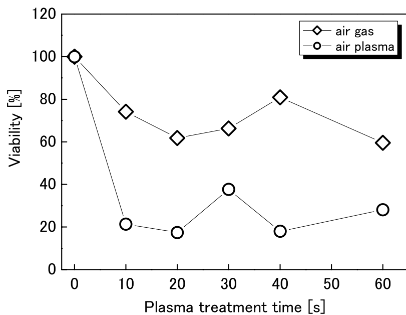
図 6-7 空気ガス及びプラズマによる HeLa 細胞の活性力の変化
