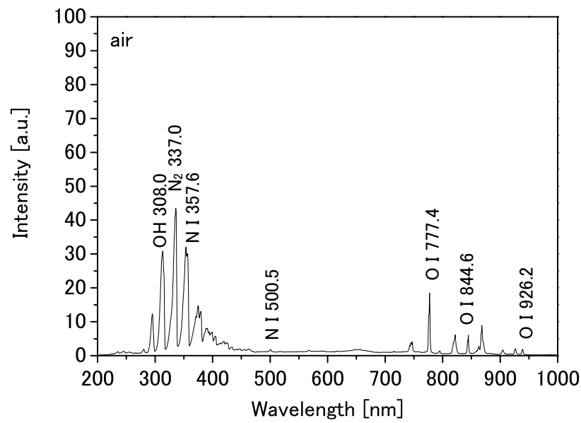
図 7-5 空気プラズマの発光スペクトル
