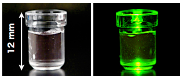
図 7-38 未処理の過酸化水素のプロープ(左図：蛍光灯下, 右図：535 nm の LED 下)
