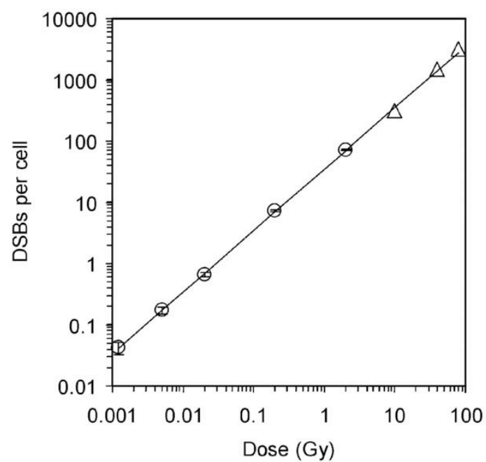
図 6-29 X 線照射による MRC-5 細胞の DNA の二本鎖切断 [69]
