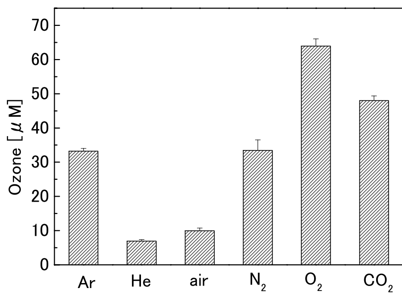
図 7-35 各種プラズマガスにおける液中のオゾン濃度
