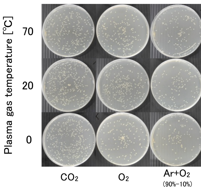
図 5-6 各ガス種のプラズマのガス温度による殺菌効果への影響
