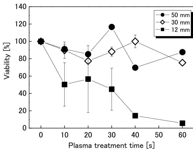
図 6-14 照射距離と Ar+O 2 プラズマによる生存率の関係
