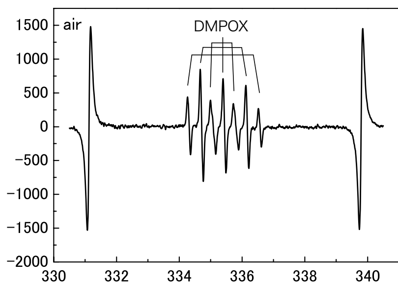
図 7-29 空気プラズマ照射時の DMPO の ESR
