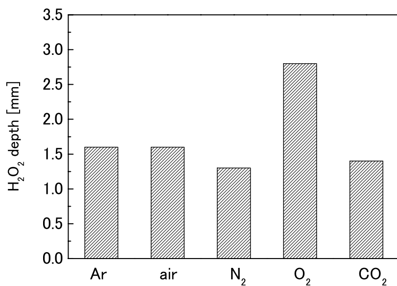
図 7-41 各ガス種のプラズマによって過酸化水素が反応する深度
