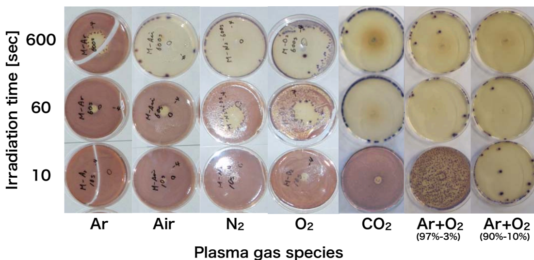
図 5-2 E.coli に対する各ガス種の効果
