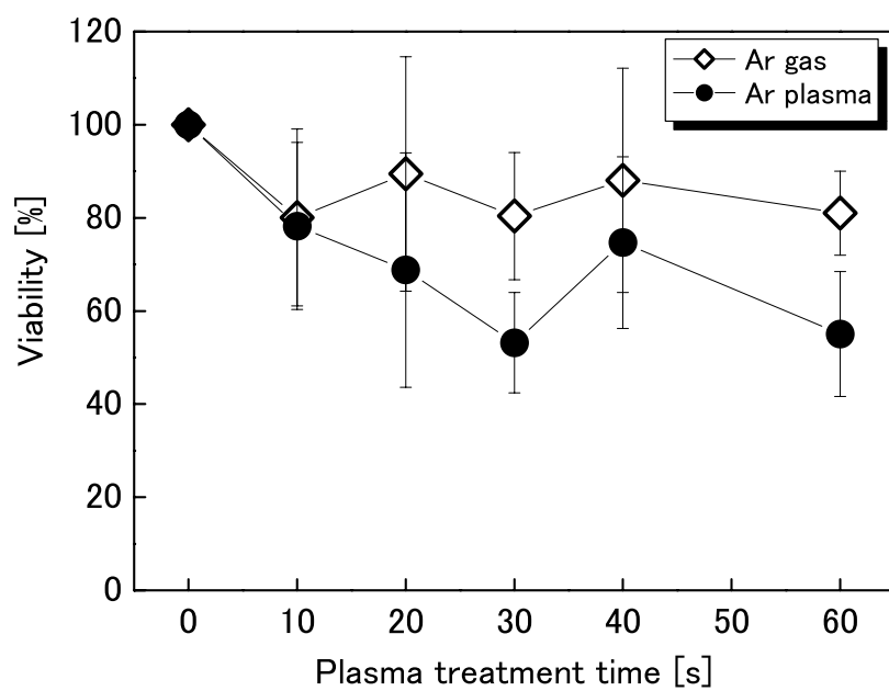
図 6-6 アルゴンガス及びプラズマによる HeLa 細胞の生存率の変化
