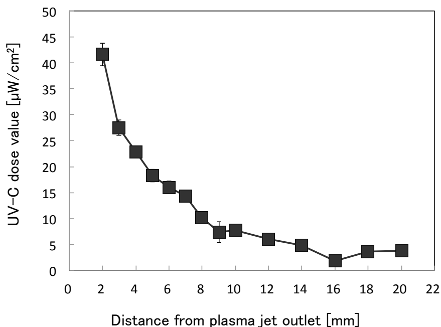
図 3-22 窒素プラズマから発せられる UV-C の紫外線量の距離依存性
