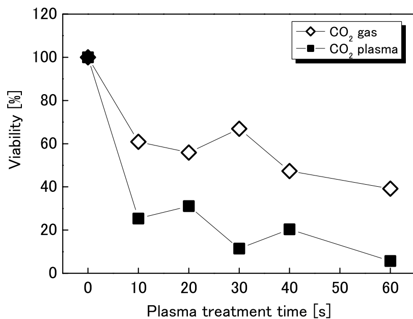
図 6-10 二酸化炭素ガス及びプラズマによる HeLa 細胞の生存率の変化
