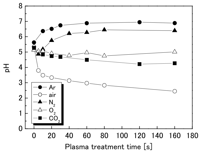
図 3-24 各ガス種のプラズマ照射による蒸留水の pH 変化
