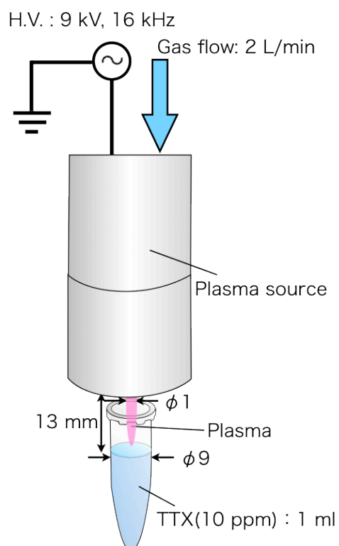
図 5-44 TTX 溶液に対するプラズマ照射
