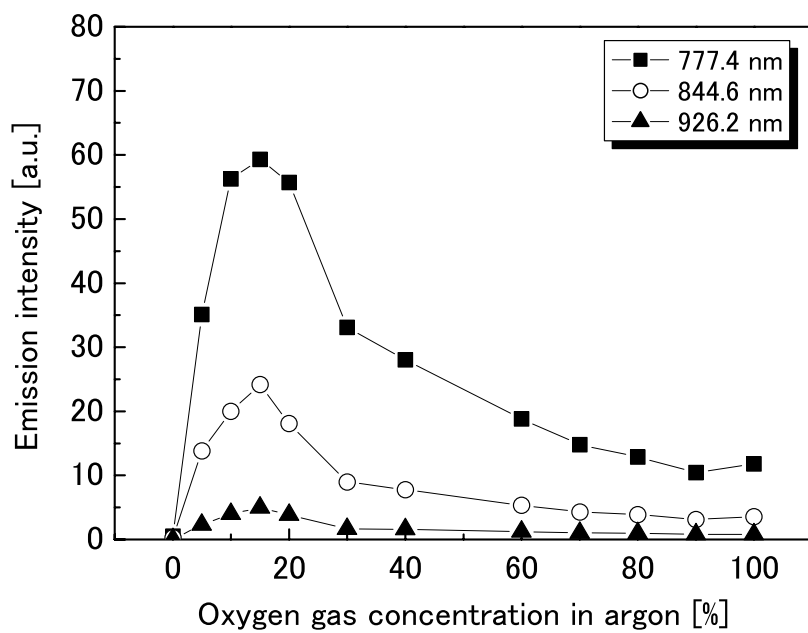
図 7-9 酸素原子線強度に関する酸素混合アルゴンプラズマの混合比依存性
