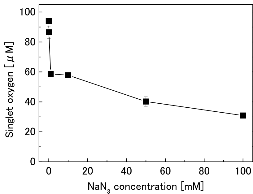
図 7-21 \text{NaN}_3 による酸素プラズマの一重項酸素量の減少
