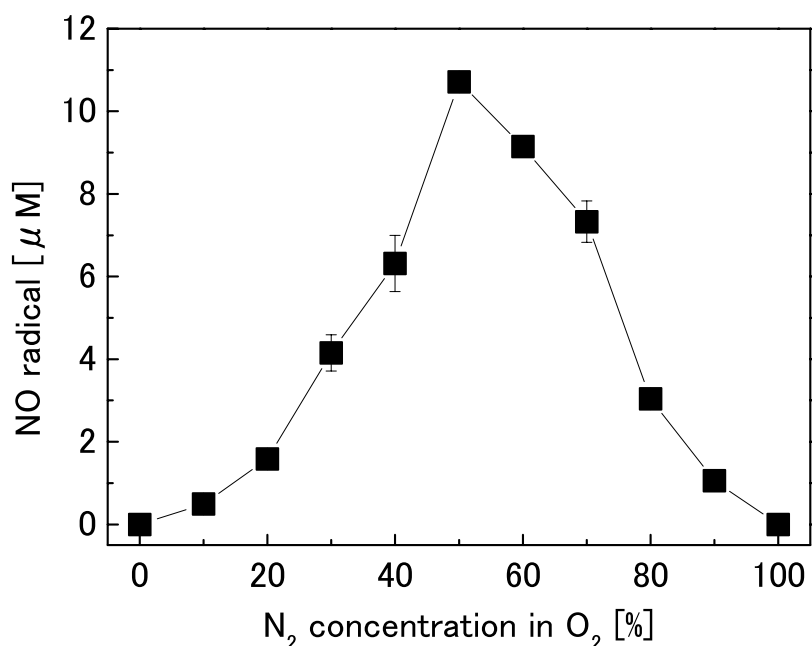
図 7-33 各 N 2 /O 2 混合プラズマの NO ラジカル量
