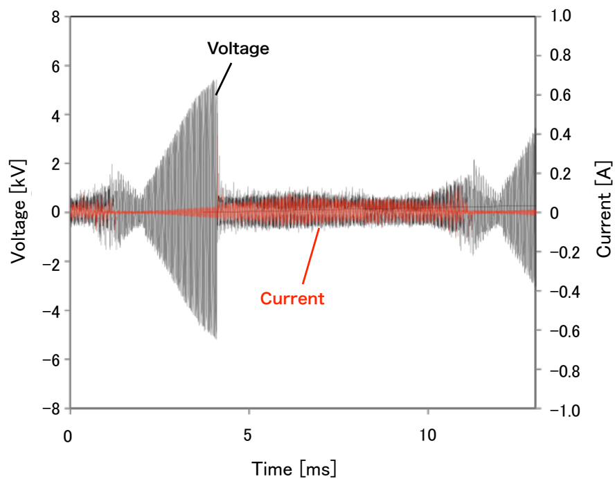
図 3-14 窒素プラズマ生成時の電圧及び電流波形
