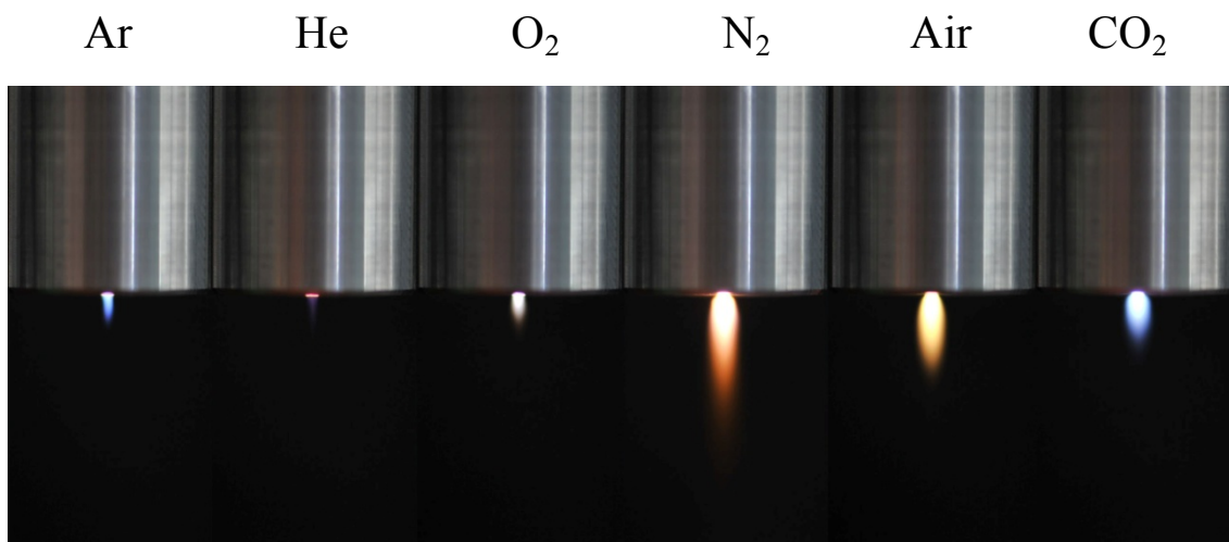
図 3-3 各種ガスで生成したプラズマ
