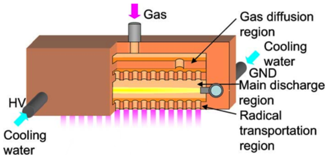
図 2-7 大気圧非平衡アルゴンプラズマ
