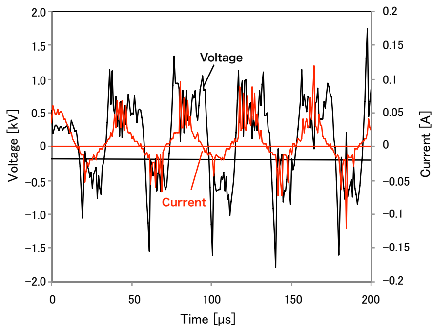
図 3-17 酸素プラズマの放電部の電圧及び電流波形
