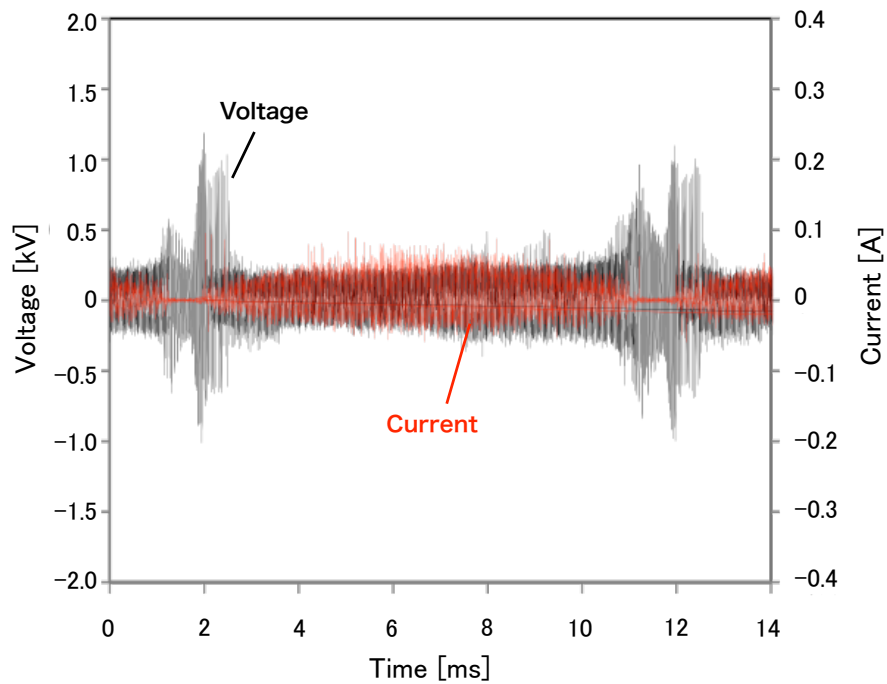
図 3-8 アルゴンプラズマ生成時の電圧及び電流波形
