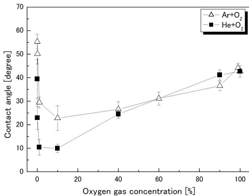
図 4-5 アルゴン酸素及びヘリウム酸素プラズマの親水化効果の混合率依存性
