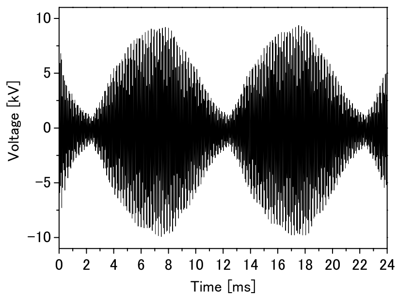
図 3-7 無負荷時の電圧波形
