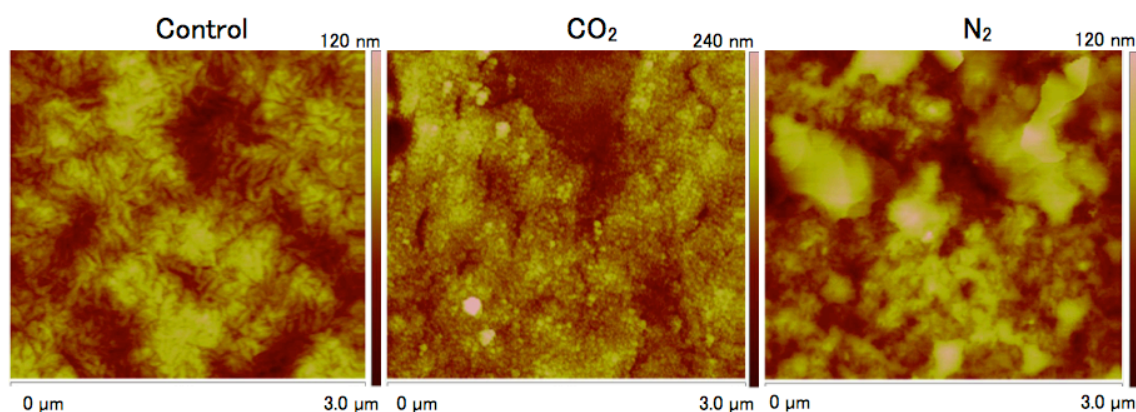
図 4-11 AFM による Non-coat のセルデスク表面の観察 (左図：未処理，中央：二酸化炭素プラズマ処理，右図：窒素プラズマ処理)
