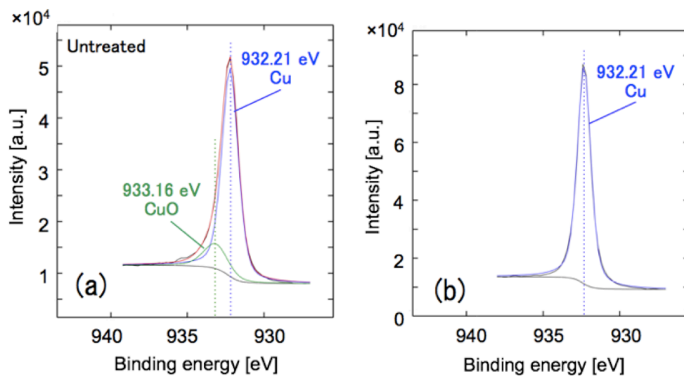
図 4-21 (a)プラズマ処理前の銅板表面の XPS のスペクトル.(b)プラズマ処理後の銅板表面の XPS のスペクトル(照射距離 1 mm, アルゴンガス 10 L/min, 水素添加濃度 3%, 入力電力 100 W, 搬送速度 10 mm/s)
