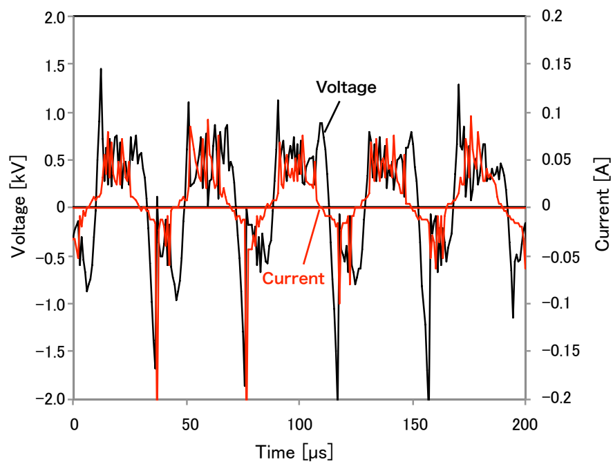
図 3-19 二酸化炭素プラズマの放電部の電圧及び電流波形
