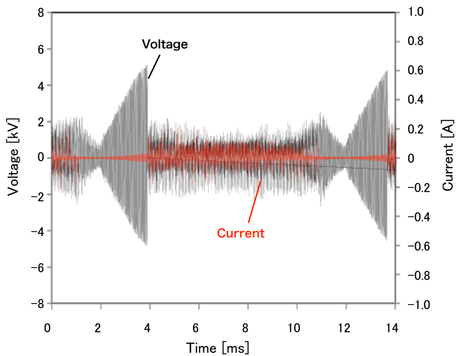
図 3-16 酸素プラズマ生成時の電圧及び電流波形
