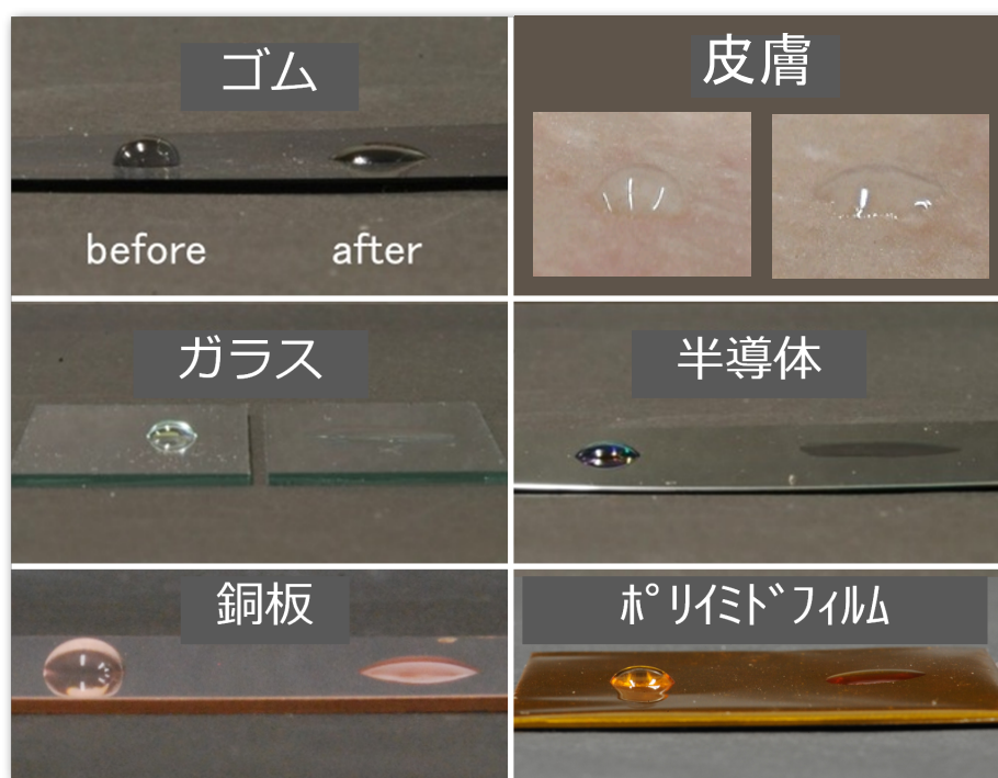
図 4-1 各材質に対するプラズマ処理のぬれ性変化
