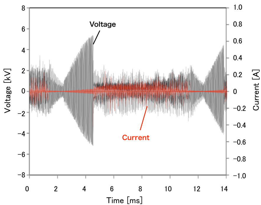
図 3-18 二酸化炭素プラズマ生成時の電圧及び電流波形
