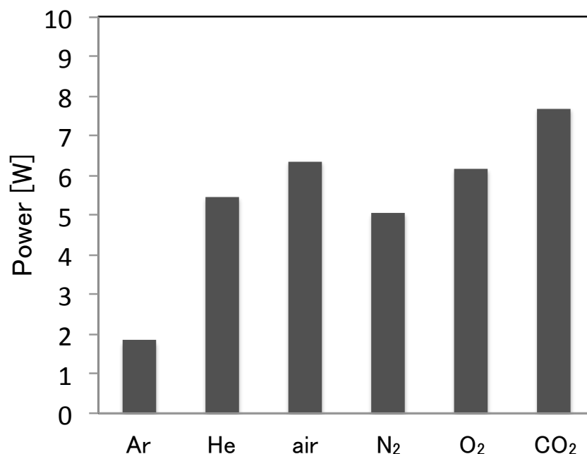
図 3-20 各ガス種のプラズマ生成時における電力
