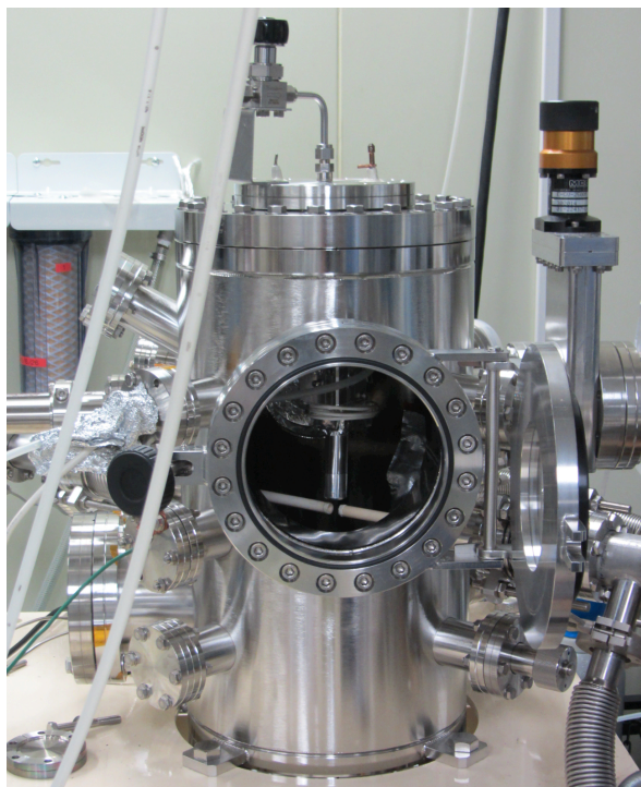
図 7-14 真空紫外吸光分光装置
