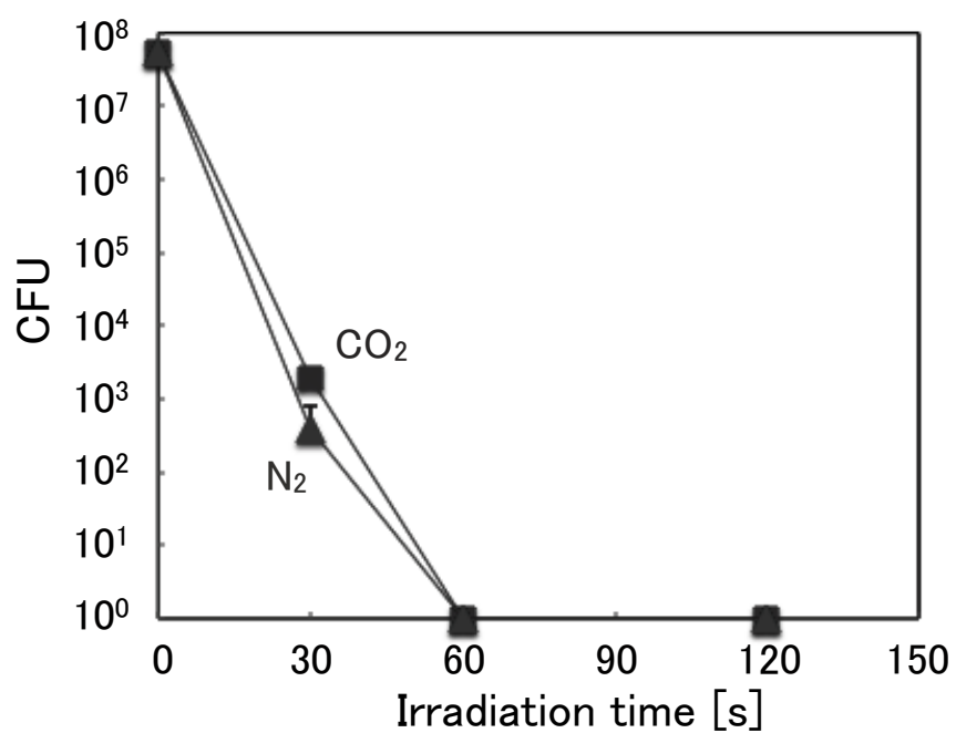
図 5-13 一般細菌(腸球菌)に対する殺菌効果
