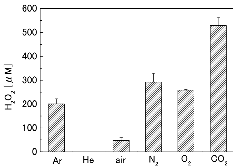
図 7-34 各種プラズマガスにおける液中の過酸化水素濃度
