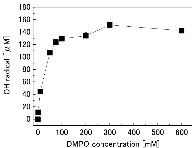
図 7-23 窒素プラズマにおける ESR スペクトルの DMPO 濃度依存性
