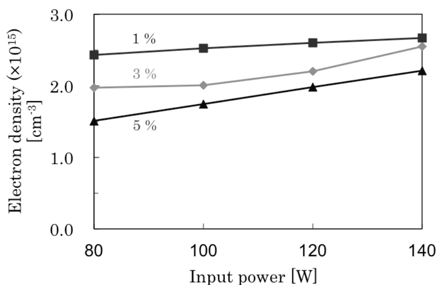
図 4-19 電子密度の水素混合濃度および入力電力依存性
