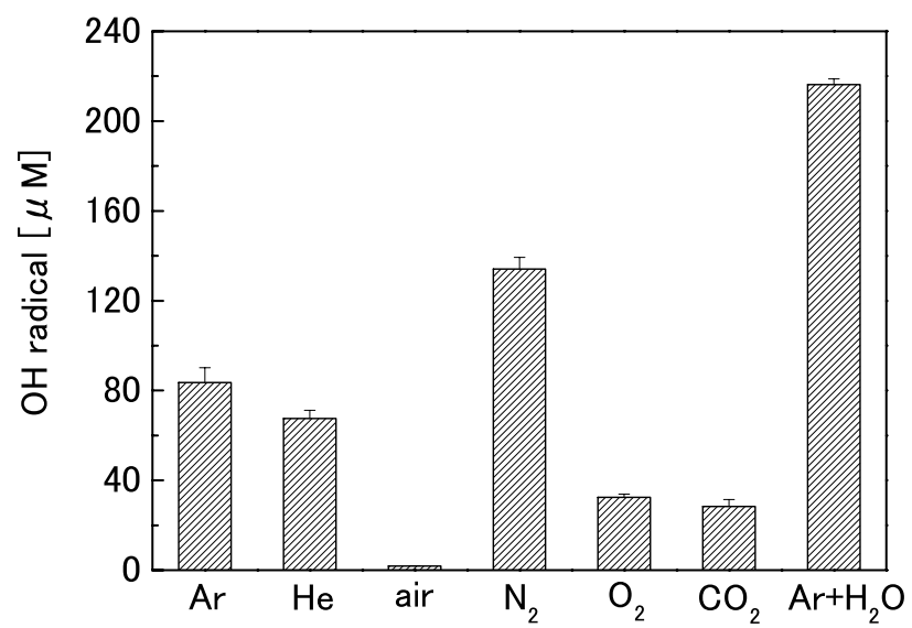
図 7-27 各ガス種による OH ラジカルの生成量
