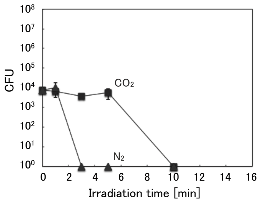
図 5-17 糸状真菌(水虫菌 T. rubrum )に対する殺菌効果
