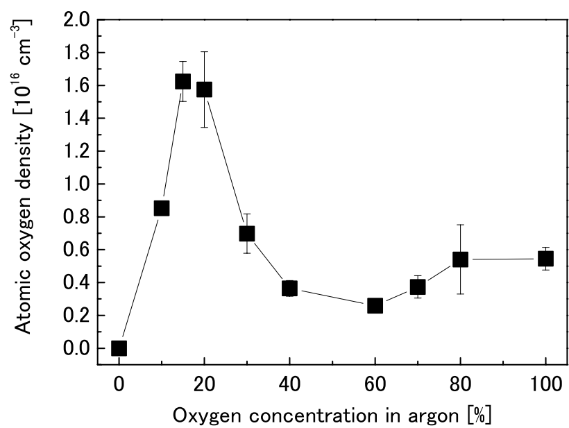
図 7-17 酸素原子生成の酸素濃度依存性
