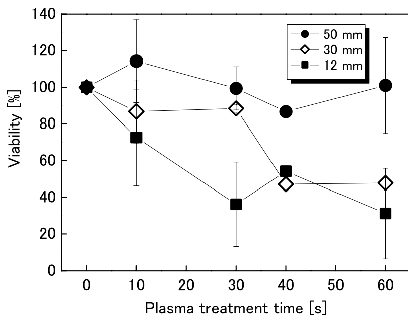
図 6-15 照射距離と Ar+CO 2 プラズマによる生存率の関係
