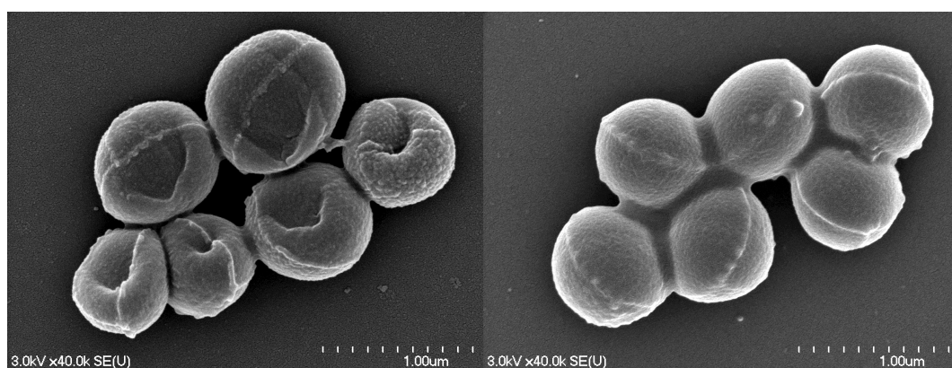
図 5-32 窒素プラズマ照射した黄色ブドウ球菌(左:10 秒, 右:120 秒)
