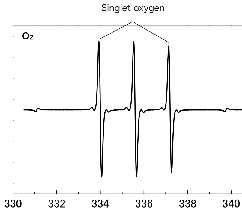
図 7-19 一重項酸素生成時の ESR スペクトル
