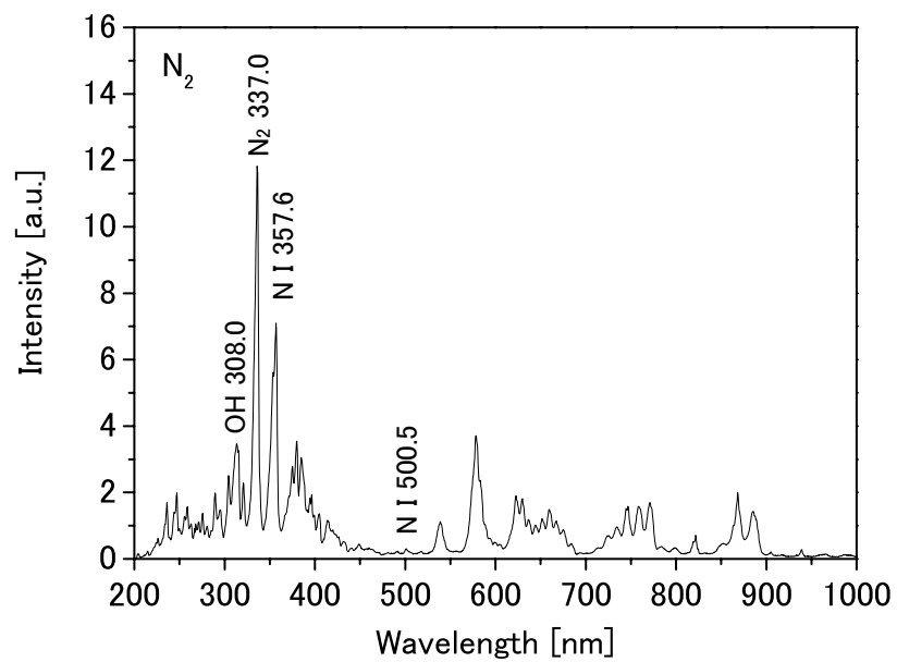
図 7-6 窒素プラズマの発光スペクトル
