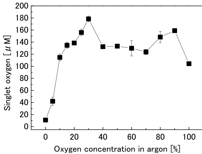
図 7-31 各 Ar/O 2 混合プラズマの一重項酸素量
