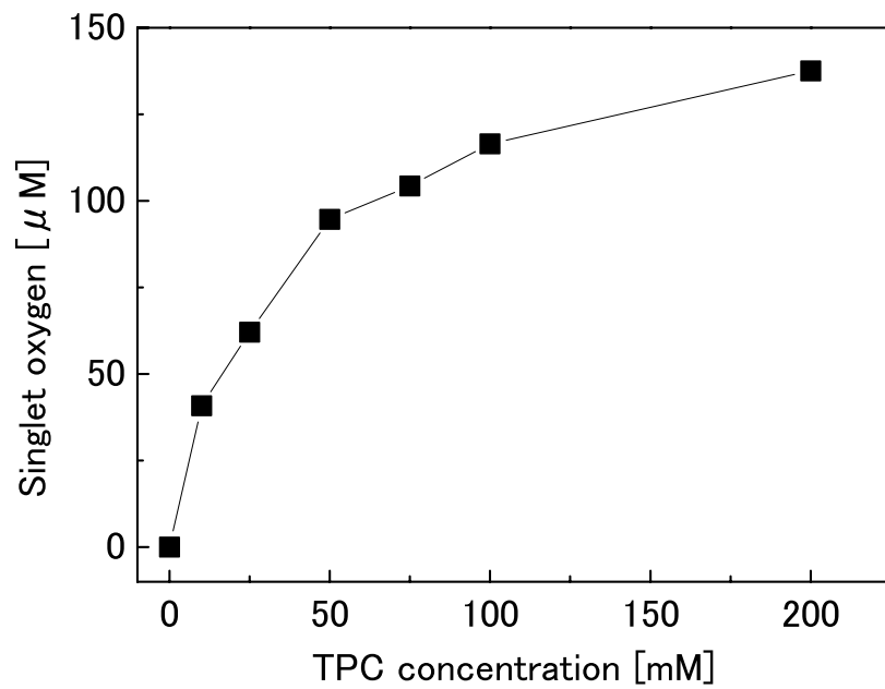
図 7-20 酸素プラズマにおける ESR スペクトルの TPC 濃度依存性
