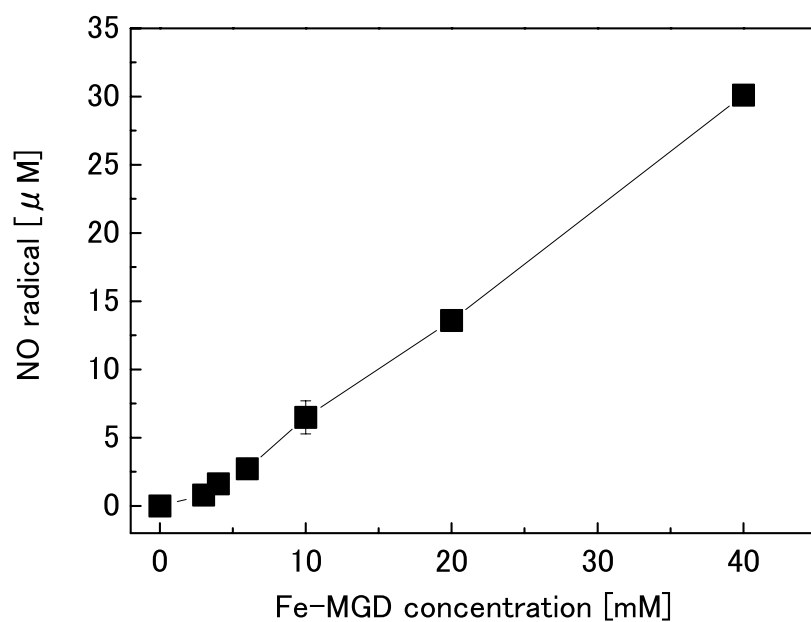
図 7-25 空気プラズマにおける ESR スペクトルの Fe-MGD 濃度依存性
