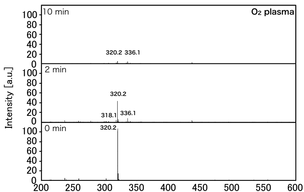
図 5-48 酸素プラズマ照射前後の質量スペクトル
