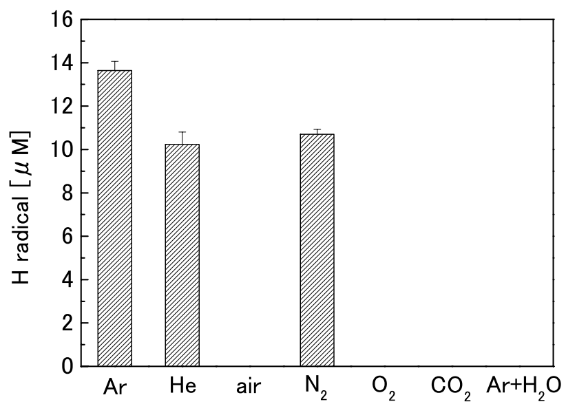
図 7-28 各ガス種による H ラジカルの生成量
