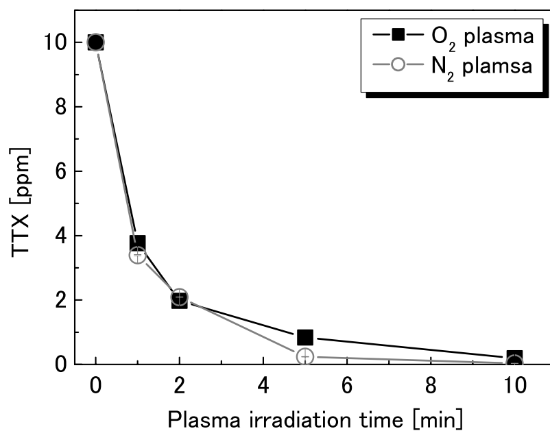
図 5-47 酸素及び窒素プラズマ照射による TTX の濃度
