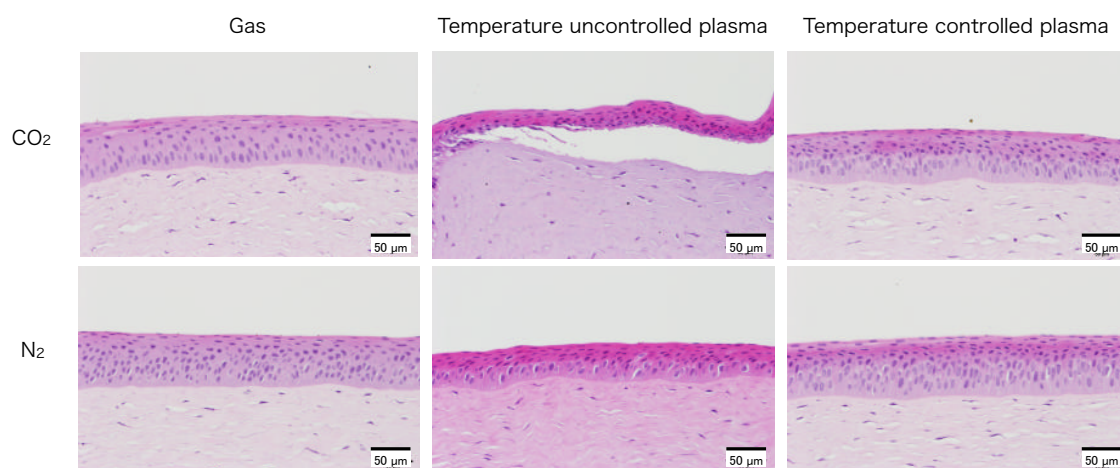
図 6-32 角膜に対する二酸化炭素及び窒素の各条件 1 min 照射の病理像(左：ガス照射，中：温度制御無しのパラズマ照射，右：温度制御パラズマ照射)
