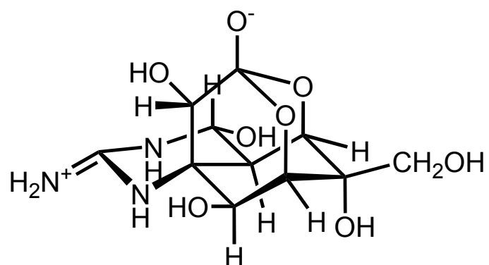
図 5-43 Tetrodotoxin (TTX)
