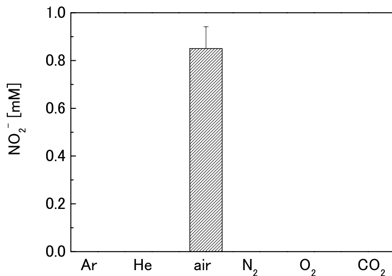
図 7-37 各種プラズマガスにおける液中の亜硝酸イオン濃度
