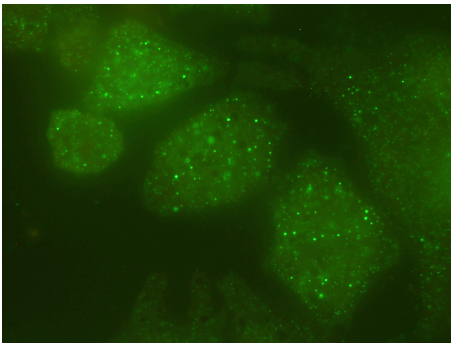
図 6-28 窒素プラズマ処理した HeLa 細胞における \gamma -H2AX 免疫蛍光染色像 (図 6-27 と同じ視野を観察した。)
