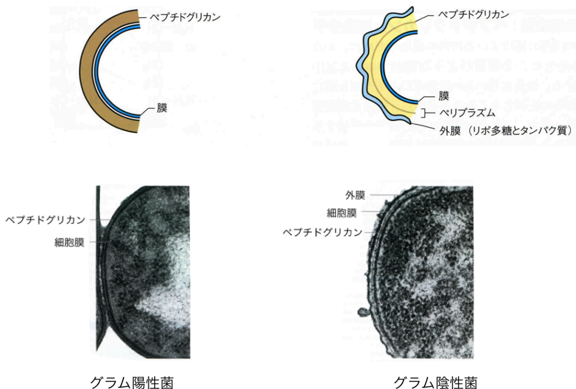
図 2-10 グラム陽性菌とグラム陰性菌の構造 [25]
