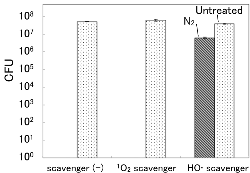
図 5-29 活性種消去剤を混合した場合の抗酸菌( M. abscessus )に対する殺菌効果
