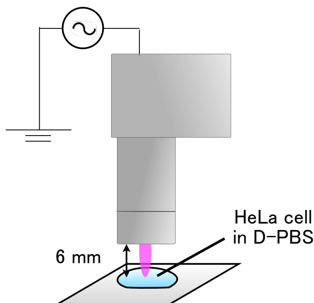
図 6-24 HeLa 細胞への照射
