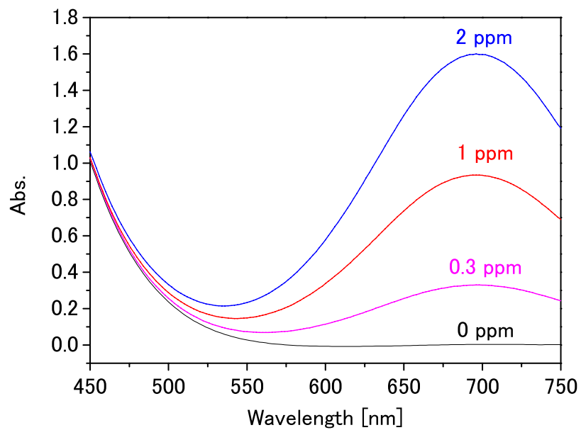
図 7-43 アンモニア測定キットによる吸光度測定
