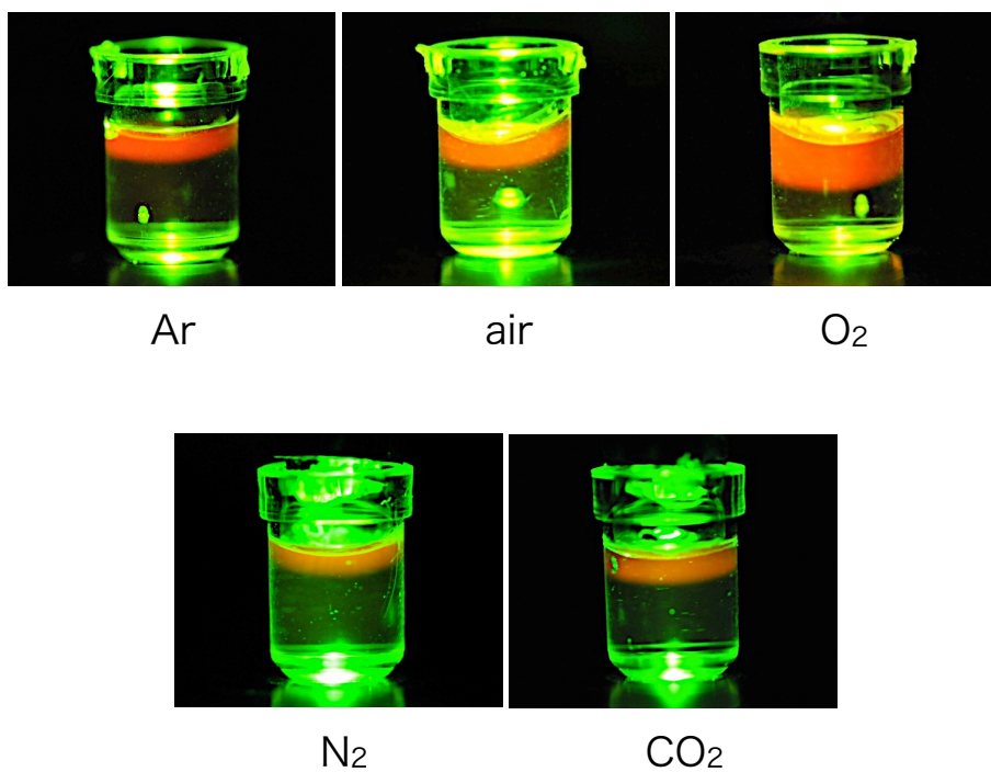
図 7-40 各ガス種のプラズマによる過酸化水素のプロープの蛍光
