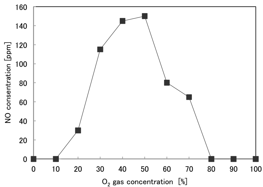
図 7-11 プラズマ生成時における N 2 と O 2 の比と NO の濃度の関係
