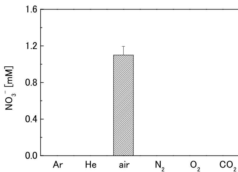
図 7-36 各種プラズマガスにおける液中の硝酸イオン濃度
