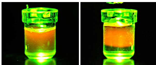
図 7-39 各条件における過酸化水素のプロープの蛍光(左図：紫外線 15 分照射, 右図：3%過酸化水素 30 \mu\text{l} 滴下)
