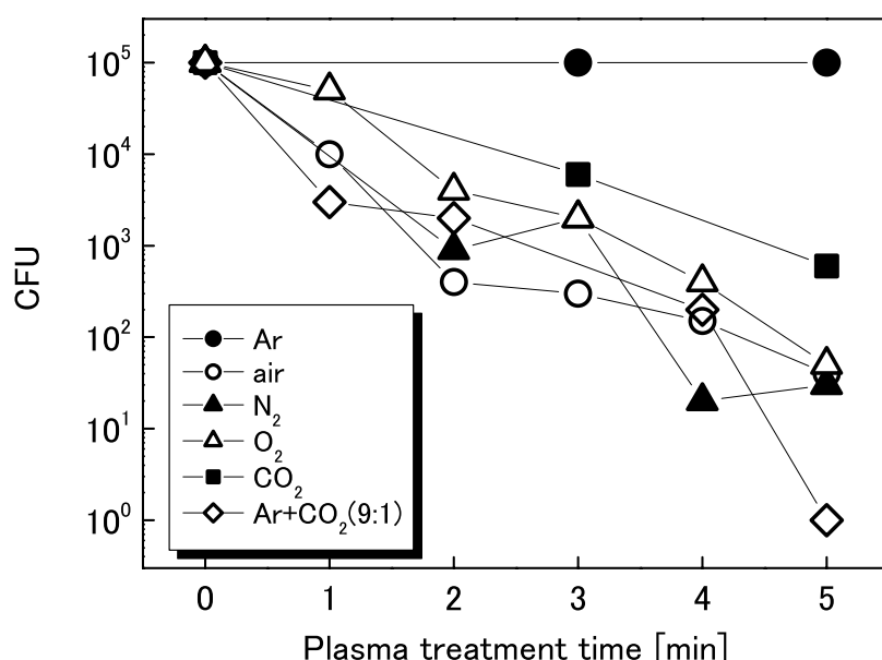
図 5-37 B.subtilis に対する各ガス種のプラズマ殺菌効果
