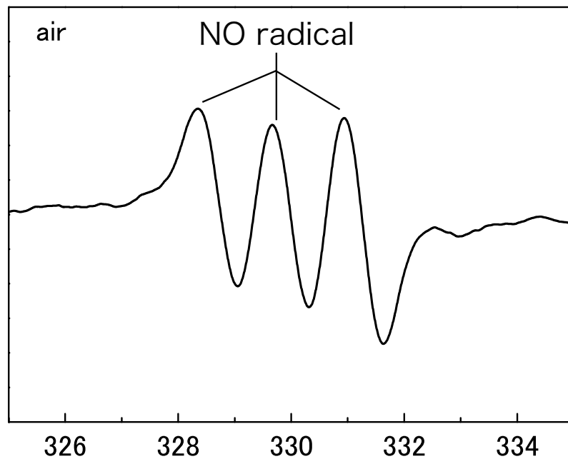
図 7-24 空気プラズマ照射時の MGD-Fe 錯体の ESR
