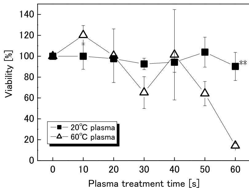
図 6-16 アルゴン酸素混合(9:1)プラズマ照射による生存率の温度依存性 (**は温度による有意性 P < 0.01 )
