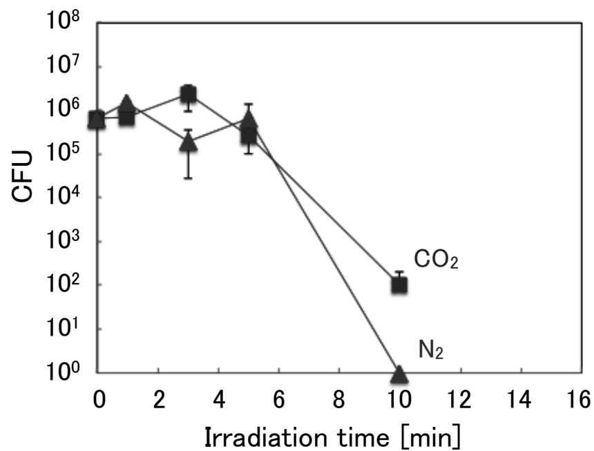
図 5-18 糸状真菌(水虫菌 T. mentagrophytes )に対する殺菌効果
