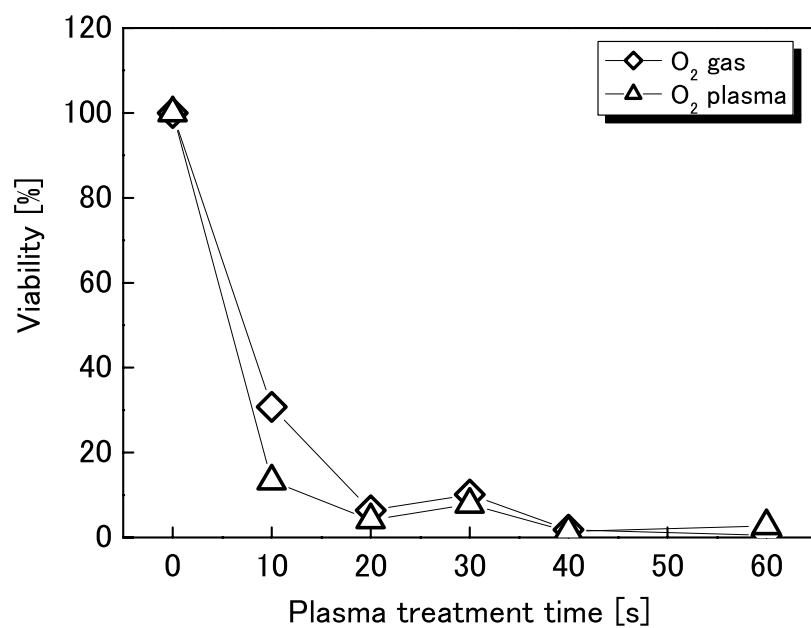
図 6-9 酸素ガス及びプラズマによる HeLa 細胞の生存率の変化
