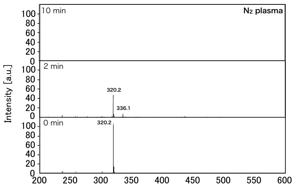
図 5-49 窒素プラズマ照射前後の質量スペクトル
