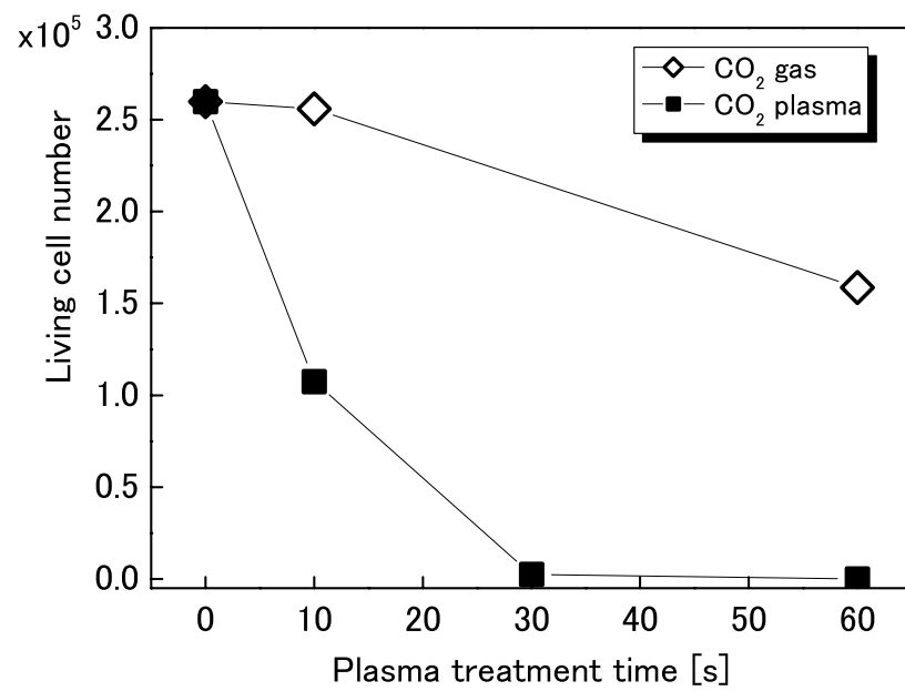
図 6-4 二酸化炭素ガス及びプラズマ照射後の生細胞数
