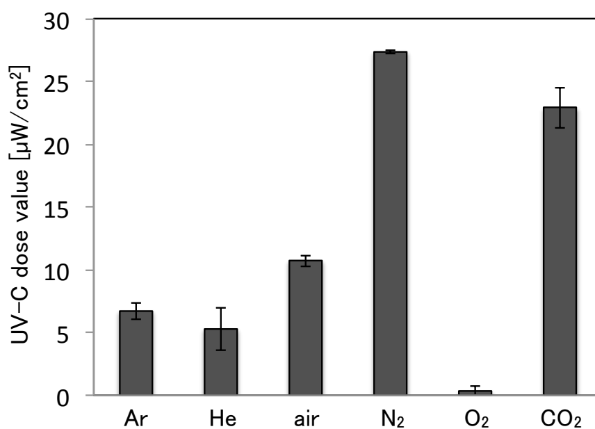
図 3-21 各ガス種のプラズマから発せられる UV-C の紫外線量
