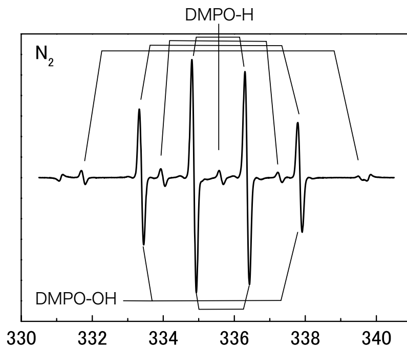
図 7-22 窒素プラズマ照射時の DMPO の ESR
