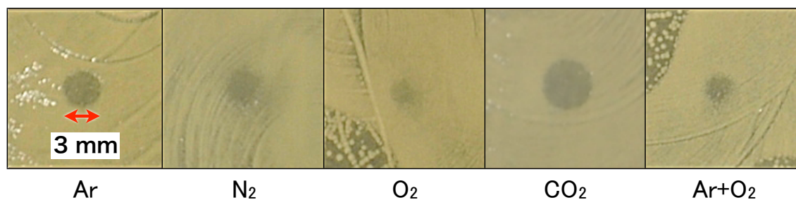
図 5-5 各ガス種のプラズマから発せられる紫外線による殺菌効果
