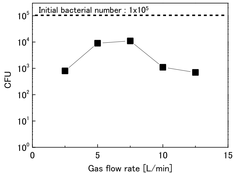
図 5-39 殺菌のガス流量依存性
