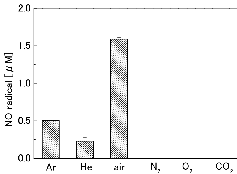
図 7-30 各ガス種による NO ラジカルの生成量
