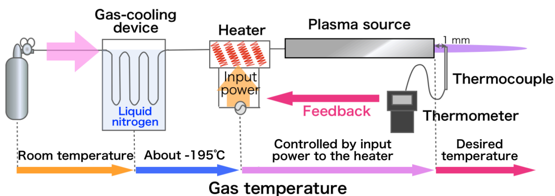
図 3-4 温度制御プラズマの機構
