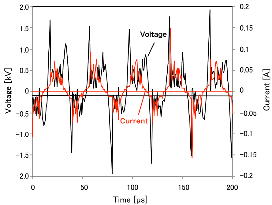
図 3-13 空気プラズマ放電部の電圧及び電流波形
