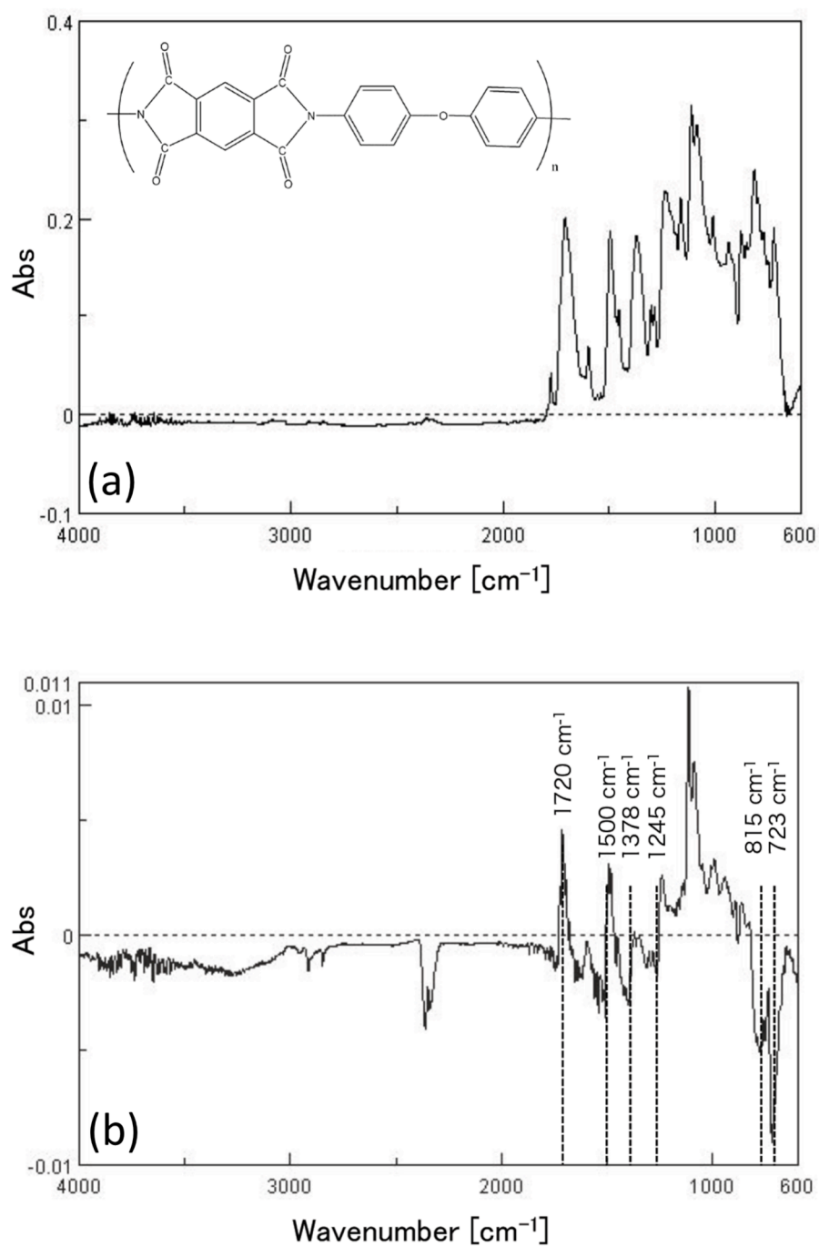
図 4-4 二酸化炭素プラズマの処理前後の ATR FT-IR スペクトル, (a) 未処理のポリイミドフィルム, (b)二酸化炭素プラズマ処理前後のスペクトルの差
