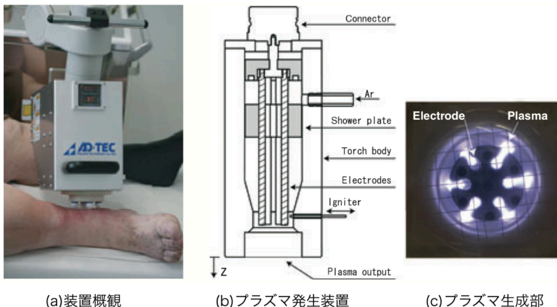
図 2-5 マイクロ波アルゴンプラズマ発生装置
