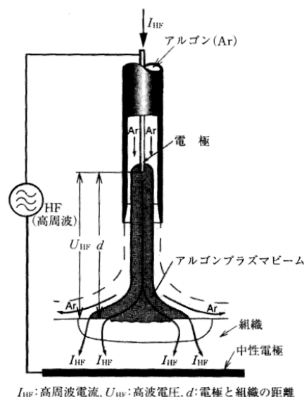
図 2-2 アルゴンプラズマ凝固装置の原理
