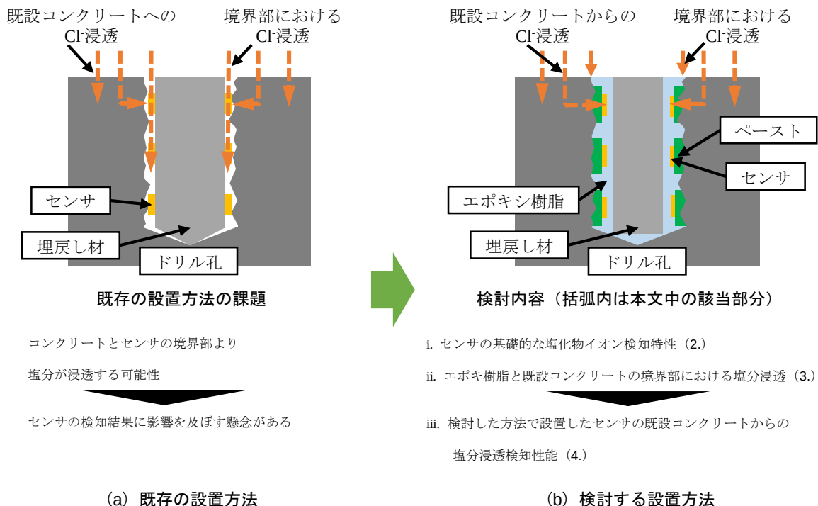
図-1 モニタリングセンサの既存の設置方法と本論で検討する設置方法の比較
