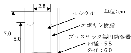
図-5 塩水圧入試験供試体寸法
