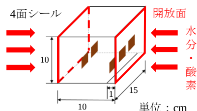
図-3 センサ検知特性試験供試体寸法
