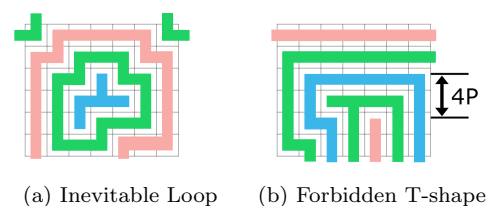
図2 SAQPの3次パターン(緑)
