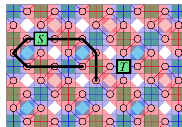
図 8 パス探索の干渉
