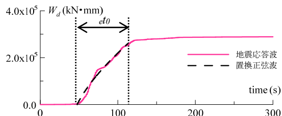
図18 吸収エネルギー時刻歴の比較
