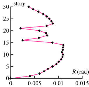
図10 層間変形角
