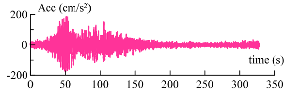
図3 三の丸波の時刻歴波形
