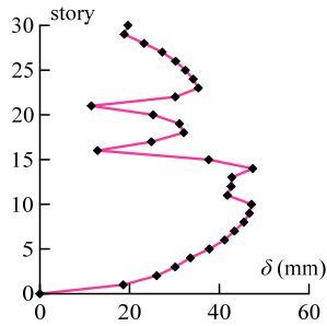
図9 層間変形
