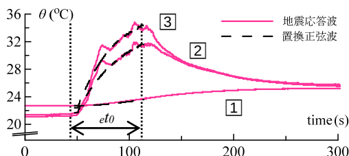
図17 B-B断面左側上段 地震応答波と置換正弦波の温度時刻歴
