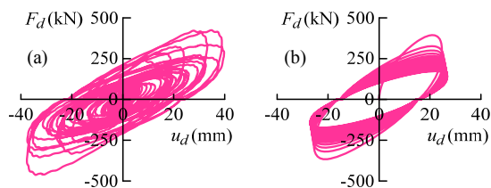
(a) 地震応答波, (b) 置換正弦波 図16 ダンパー履歴
