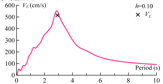
図5 三の丸波のエネルギースペクトル
