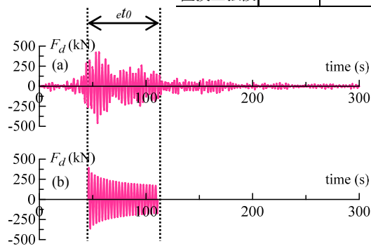
(a) 地震応答波, (b) 置換正弦波 図15 ダンパー力時刻歴波形
