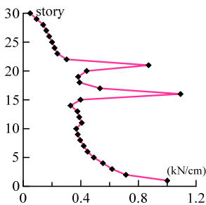
図7 剛性分布
