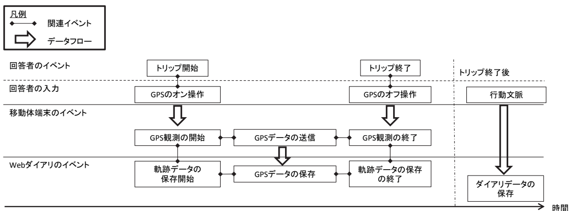
(a)従来のプローブパーソン調査システム
