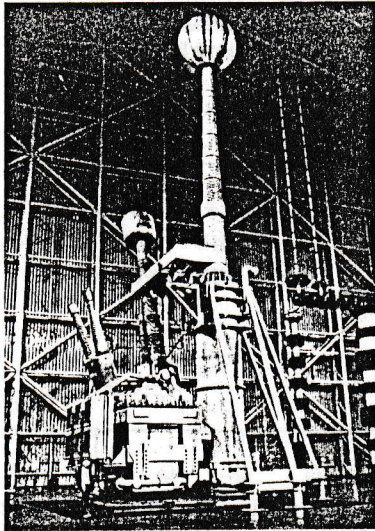
(a) UHVプロトタイプ変圧器
