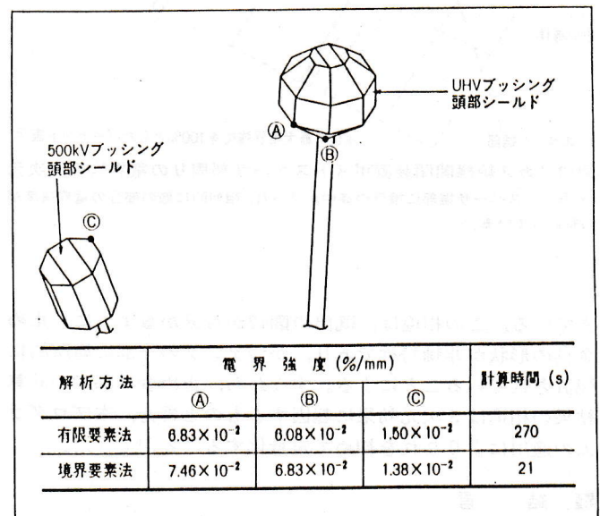
図11 BEMと有限要素法の解析精度、計算時間の比較 有限要素法モデルとBEMモデルの節点数は、各々4,500、115個である。BEMの計算時間は、有限要素法に比べて1/10以下に短縮できている。
