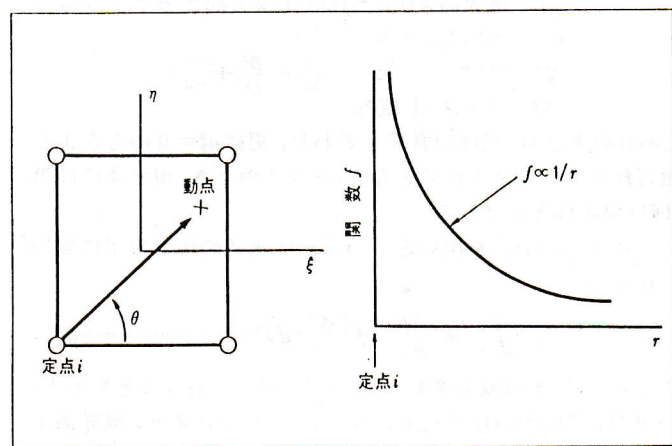
図2 定点近傍での被積分関数の挙動 直交系 (\xi, \eta) →極座標系 (r, \theta) 変換により特異積分を除去できる。
