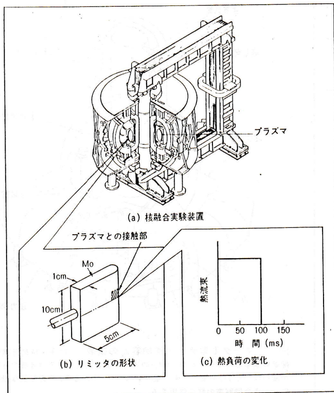
図7 核融合実験装置とリミッタ形状 プラズマとの接触によるリミッタの疲労と寿命の予測には、過渡温度解析が必要である。
