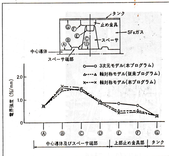
図14 軸対称モデルと3次元モデルによる計算結果の比較 止め金具、スペーサが導体周りに軸対称性を保って広がっているとして差分法で計算した結果と、BEMによる結果の比較でE、Fの位置の電界に3次元効果が現われていることが分かる。
