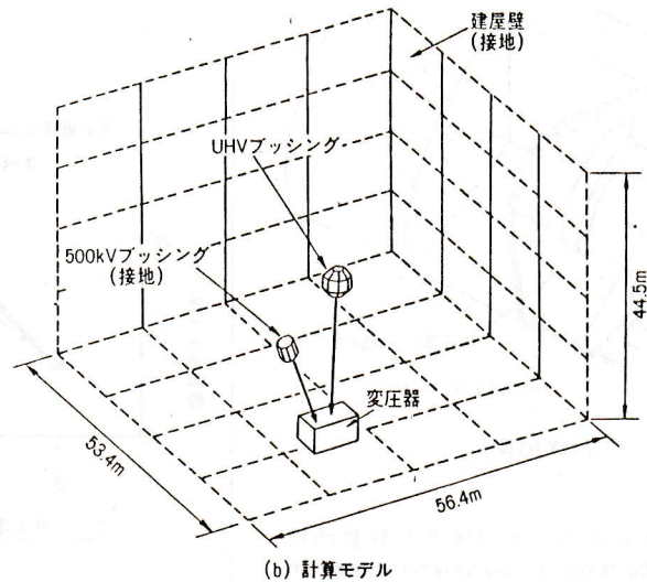
(b) 計算モデル
