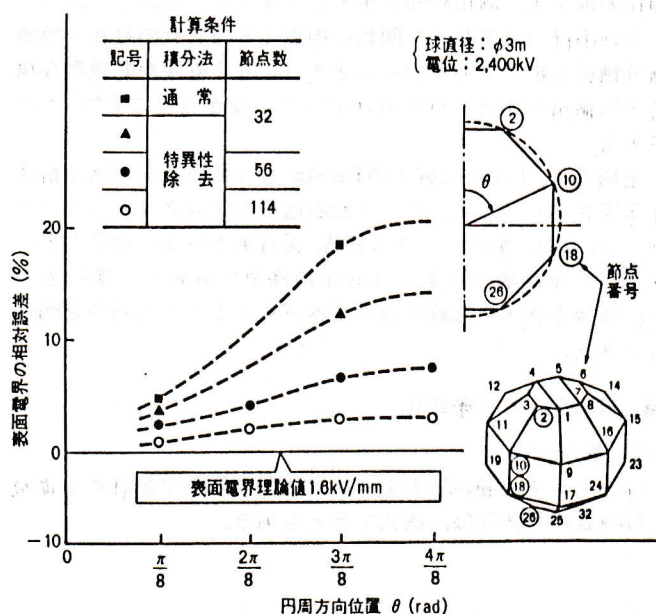
図3 積分法と節点数が数値解の精度に及ぼす影響 特異性を除去した新積分法では、精度が40%向上する。
