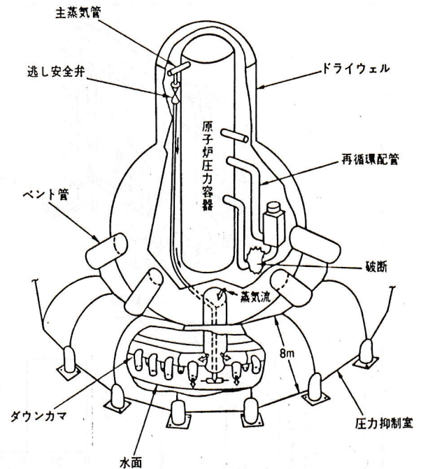
図5 マークI型原子炉格納容器の概要 原子炉格納容器の構成と配管破断事故時での冷却材(蒸気)の流れを示す。原子炉压力容器から流出した冷却材は、圧力抑制室の水中に至り凝縮する。このとき、水力学的な動荷重が発生し、圧力抑制室の壁に作用する。
