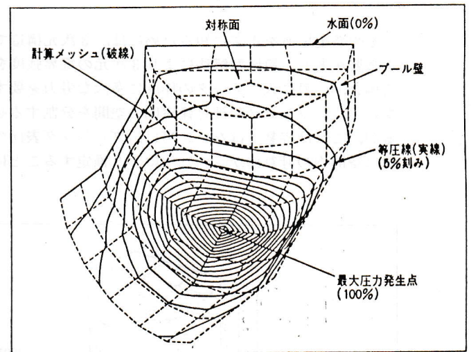
図6 圧力抑制プール壁上の圧力分布 プール中への蒸気流入に伴って発生する動的圧力の距離による減衰、圧力抑制室(トーラス形状)の \frac{1}{8} セクタの水浸部を計算領域とした。
