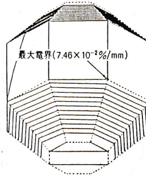
(b) UHVブッシング頭部シールド上の電界分布
