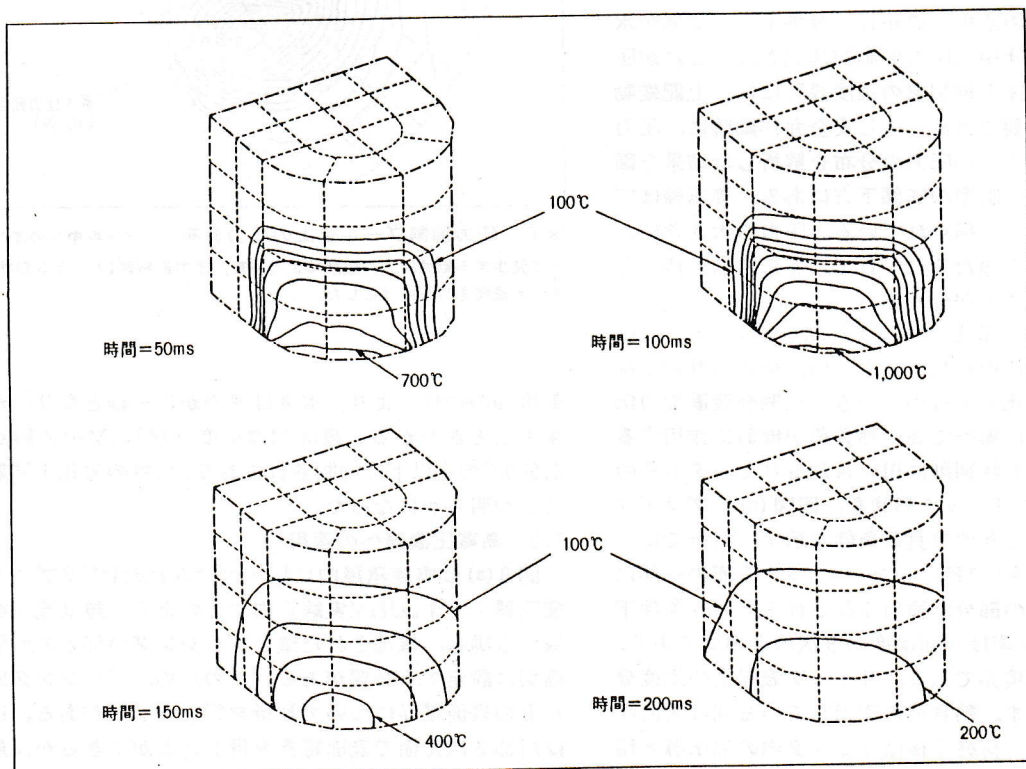
図8 プラズマ接触後のリミッタ表面上温度分布過渡変化 プラズマとの接触による高い熱負荷により、表面温度は短時間に急上昇するが、表面からの輻射冷却、材料内の熱拡散効果により、最高到達温度は材料(Mo)の融点(2,600°C)の \frac{1}{2} 以下に抑制されており、材料の損傷上問題はない。
