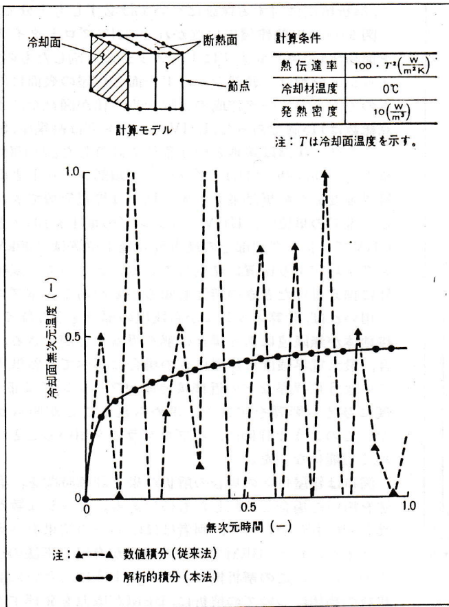
図4 非定常問題での時間積分の方法と解の安定性 熱伝達率がタイムステップ内で一定として数値積分すると、熱伝達率が温度(未知数)の関数である場合に解は発散する。しかし、解析的方法により厳密に積分すると解は収束する(本法)。
