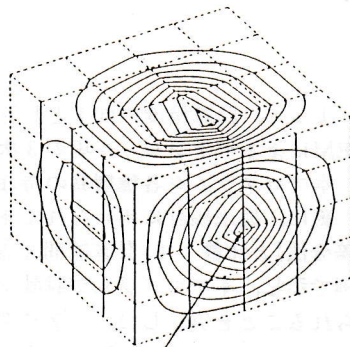
(a) 建屋上の電界分布
