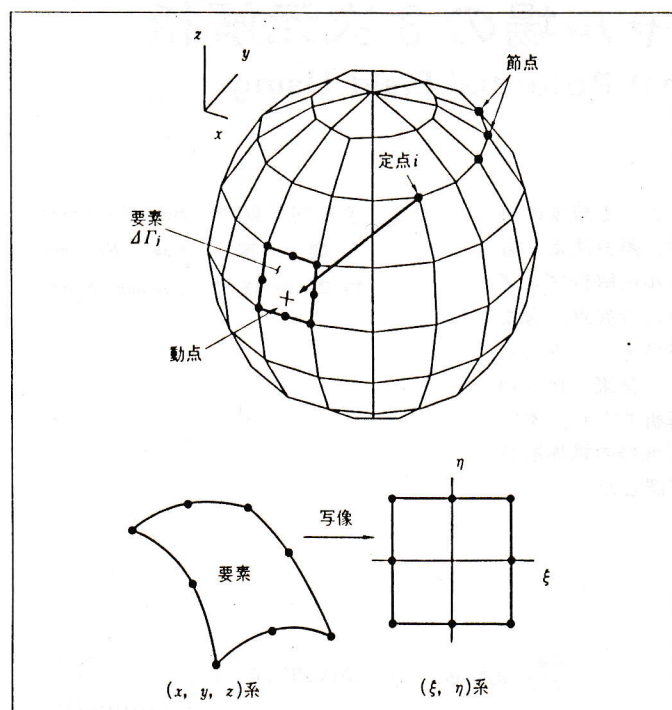
図1 BEM(境界要素法)の数値積分法 局所曲線座標変換法による積分の2次元化により、任意形状の表面積分が可能である。
