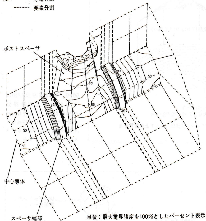
図13 ガス絶縁開閉装置ポストスペーサ部周りの電界強度3次元分布 スペーサ端部に電界の集中が見られ、相対的に他の部分の電界強度が抑制されている。
