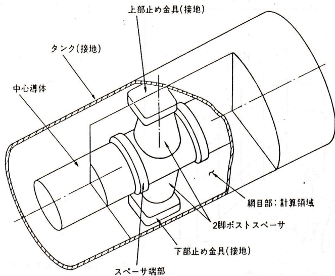
図12 ガス絶縁開閉装置のポストスペーサ部構造と計算領域 スペーサ、その端部及び止め金具部表面の電界強度分布が絶縁設計に必要である。
