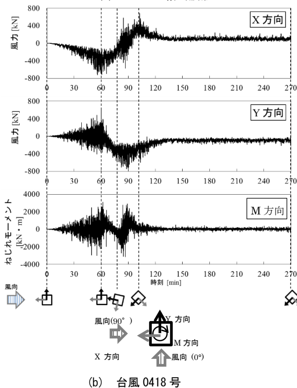
図 6 各成分の風力の時刻歴と構造軸
