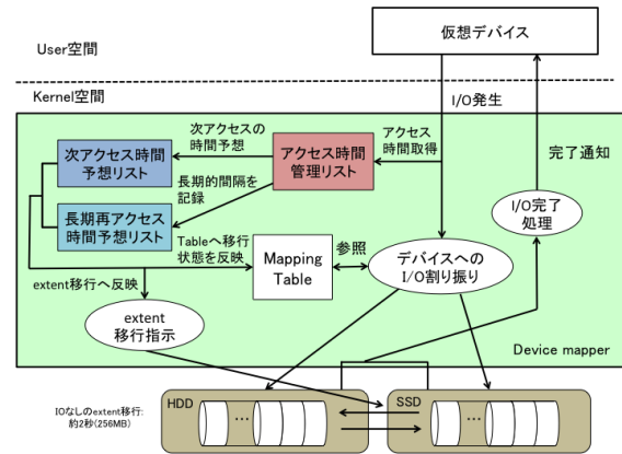
図 7 システム概要図
