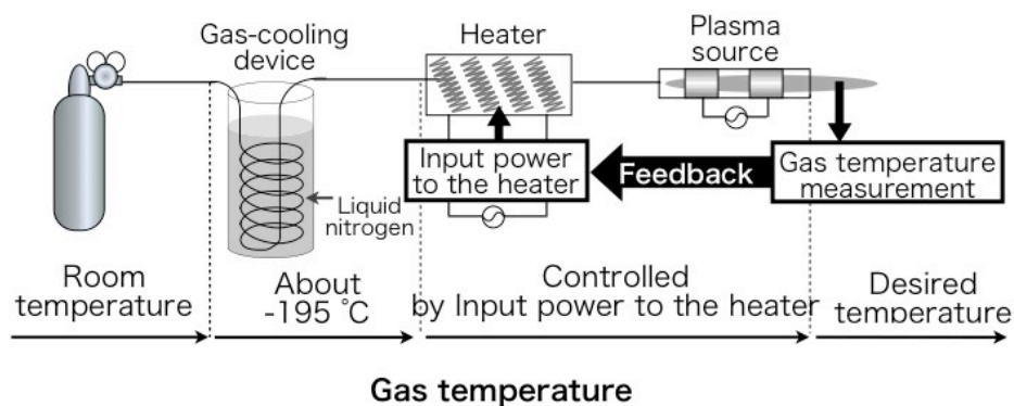
Figure 3-4 本実験の温度制御プラズマ
