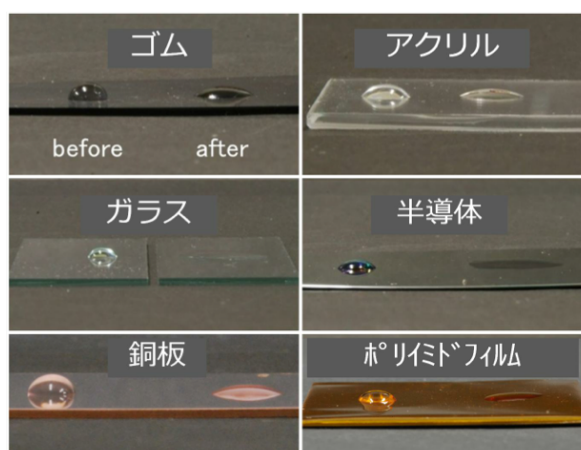
Figure 6-3 プラズマによる様々な基材の親水化
