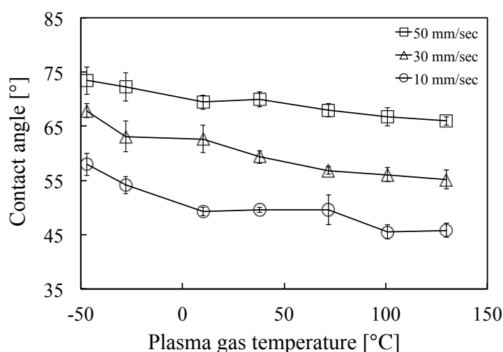
Figure 6-7 銅板におけるプラズマガス温度とプラズマ処理後の水接触角の関係
