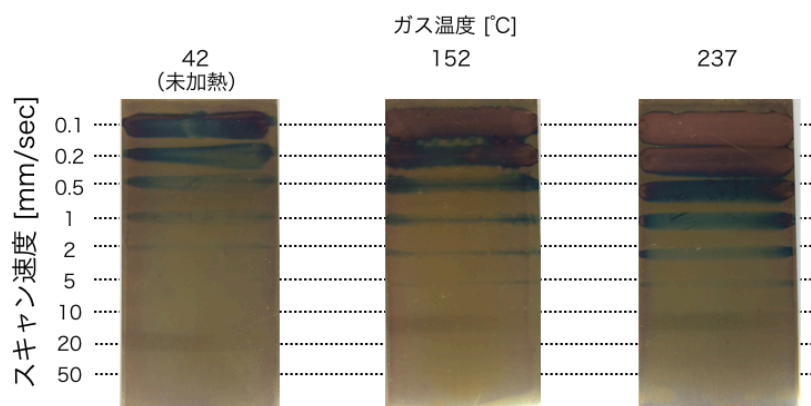
Figure 6-15 プラズマガス温度による還元効果の違い
