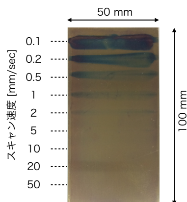
Figure 6-14 42 °C (未加熱) のプラズマで処理した銅板の様子
