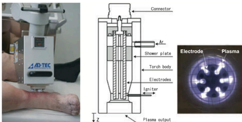
Figure 2-13 マイクロ波アルゴンプラズマ発生装置
