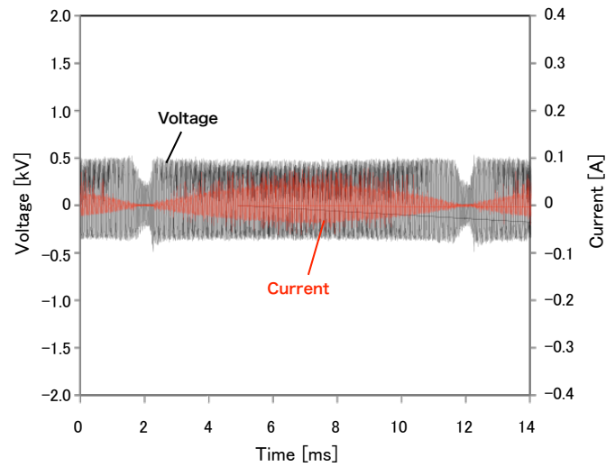
Figure 3-38 マルチガスプラズマジェットで生成したヘリウムプラズマの放電波形 [9]
