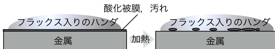
Figure 6-10 フラックスの働き
