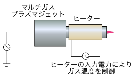
Figure 3-41 マルチガスプラズマジェットの加熱機構
