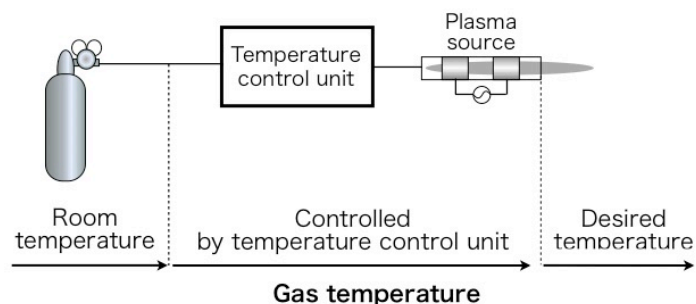
Figure 3-3 温度制御プラズマ装置の概略図
