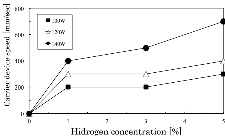
Figure 6-19 混合酸素濃度と還元処理速度の関係 [6]
