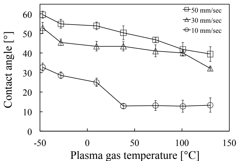
Figure 6-8 ポリイミドフィルムにおけるプラズマガス温度とプラズマ処理後の水接触角の関係
