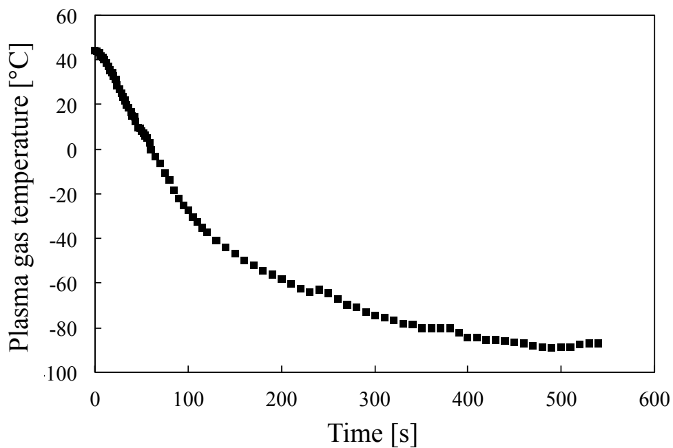
Figure 3-13 冷却実験におけるガス温度の時間変化
