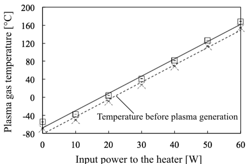
Figure 3-14 ヒーターへの入力電力とプラズマガス温度の関係
