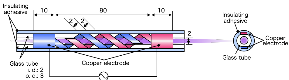
Figure 3-30 マルチガス DBD プラズマジレットの構造
