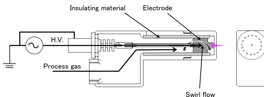
Figure 3-36 マルチガスプラズマジェットの構造
