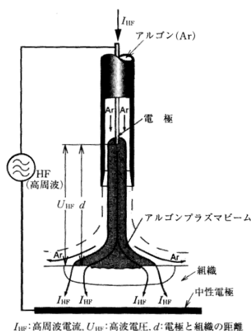
Figure 2-10 アルゴンプラズマ凝固装置
