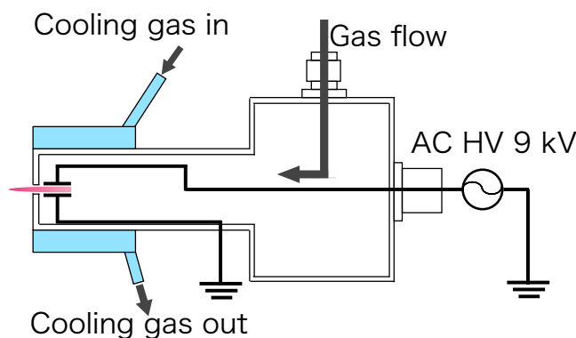
Figure 3-40 マルチガスプラズマジェットの冷却機構
