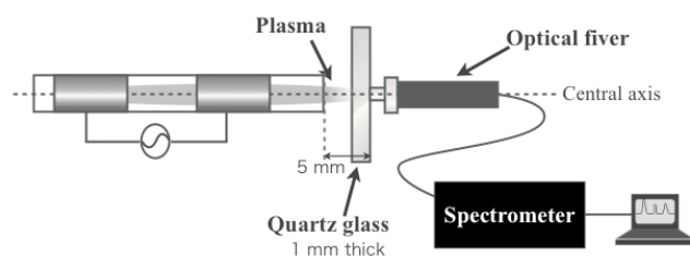
Figure 3-21 分光実験の測定システム
