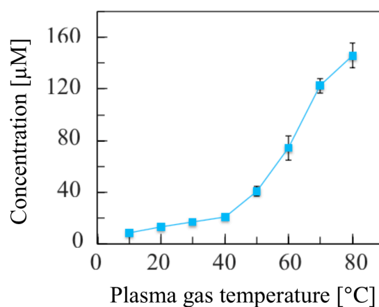
Figure 5-12 ^1O_2 生成量のプラズマガス温度依存性
