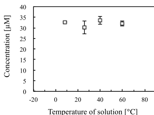
Figure 5-17 水温と OH \cdot 生成量の関係
