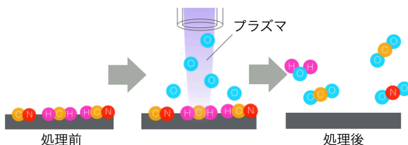
Figure 6-1 プラズマによる表面洗浄の模式図
