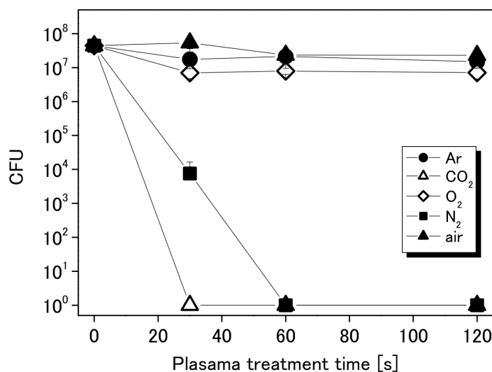
Figure 5-4 大腸菌殺菌効果のガス種依存性 [1]
