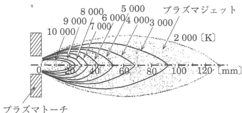
Figure 2-2 熱プラズマの温度分布
