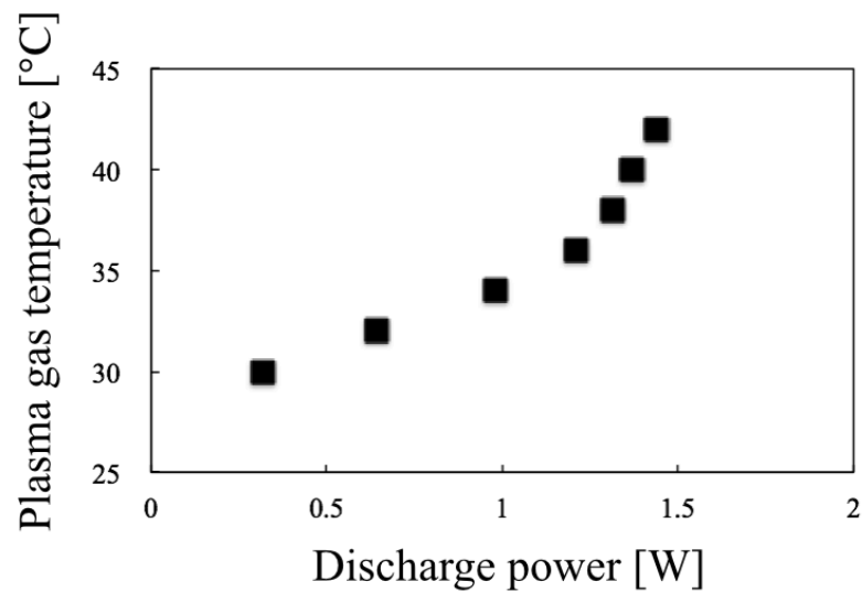
Figure 4-3 プラズマガス温度と電子密度の関係
