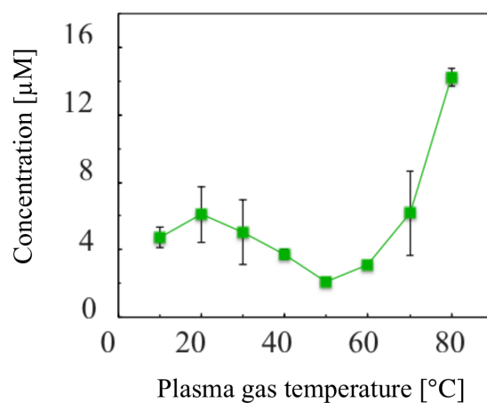
Figure 5-14 H 2 O 2 生成量のプラズマガス温度依存性
