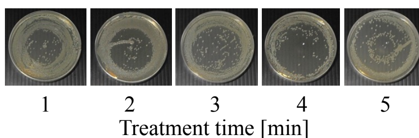
Figure 4-8 照射時間と殺菌範囲の関係
