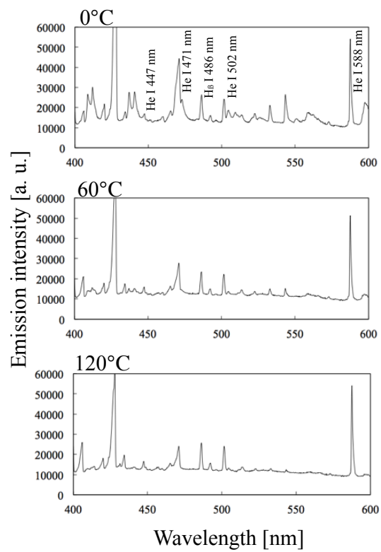
Figure 3-22 ガス温度による可視光スペクトルの変化
