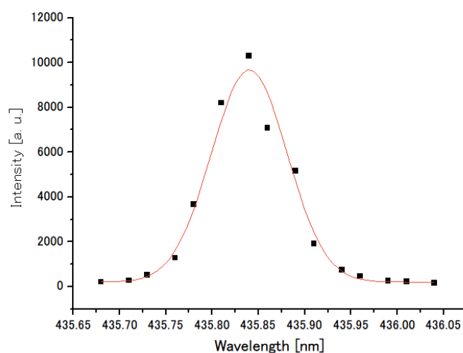
Figure 3-19 Hg I 435.83\text{ nm} 発光スペクトルのガウス関数によるフィッティング
