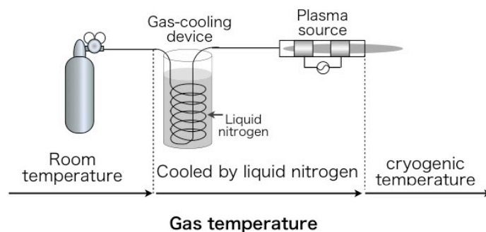
Figure 3-2 大気圧クライオプラズマのガス温度推移
