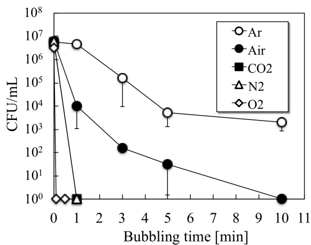
Figure 5-29 プラズマバブリング法による S. aureus の殺菌
