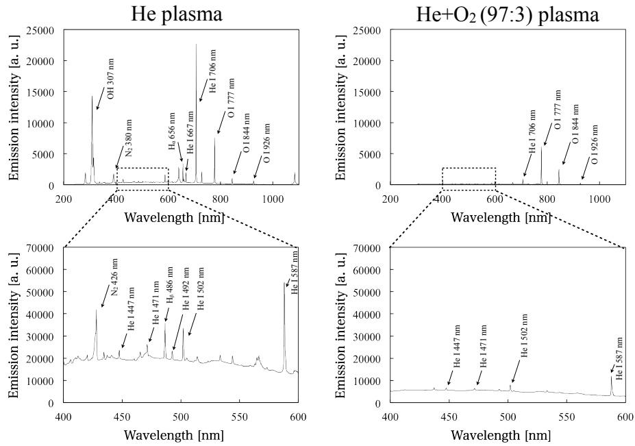
Figure 4-15 ヘリウムプラズマと酸素混合ヘリウムプラズマの発光スペクトル
