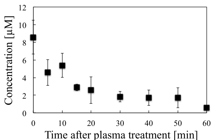
Figure 5-35 時間経過によるオゾン濃度の減衰
