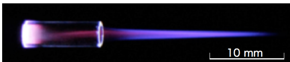
Figure 3-6 ヘリウムマイクロプラズマジェットの放電の様子
