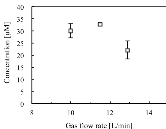
Figure 5-15 ガス流量と OH·生成量の関係
