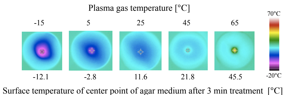
Figure 4-11 サーモグラフィーによる寒天培地の表面温度観察
