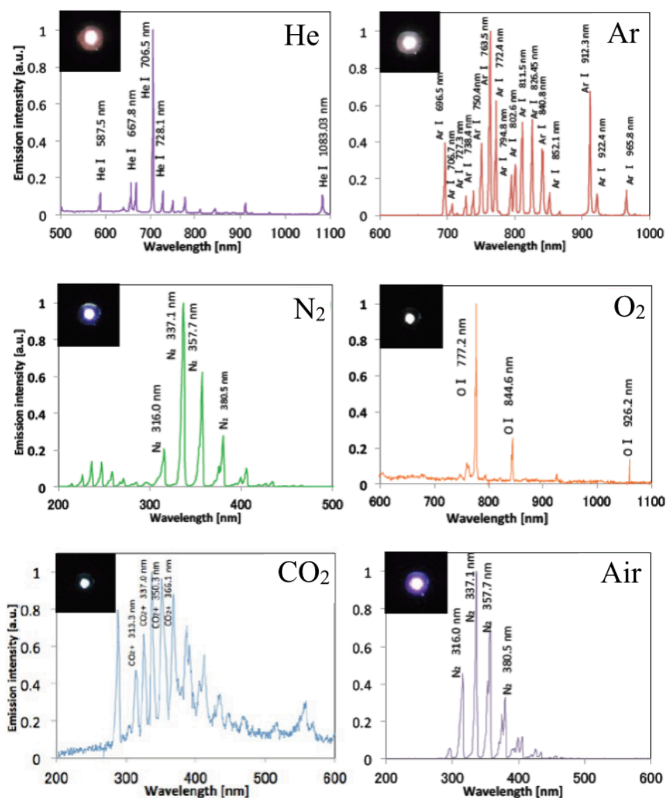
Figure 3-32 各ガス種で生成したプラズマの発光スペクトル
