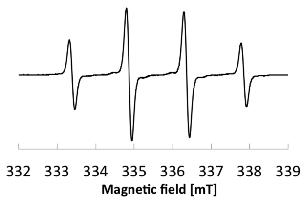
Figure 5-9 DMPO-OH の ESR スペクトル
