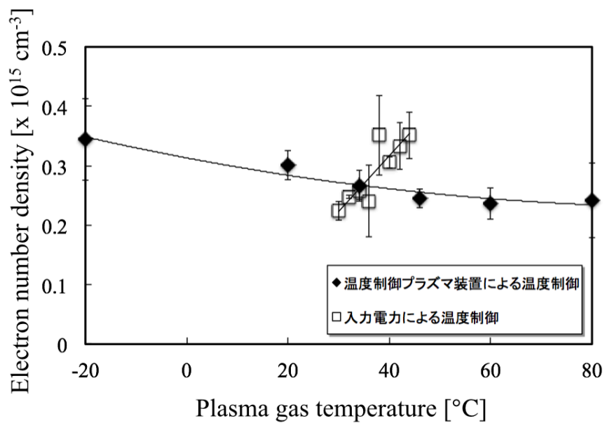
Figure 4-4 プラズマガス温度と電子密度の関係
