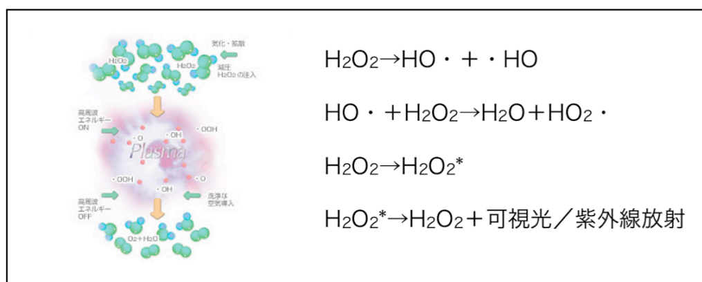
Figure 2-11 ステラッドにおける反応過程
