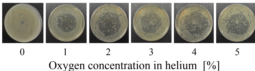
Figure 4-7 酸素混合濃度と殺菌範囲の関係
