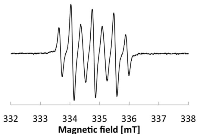
Figure 5-21 DMPO-X の ESR スペクトル
