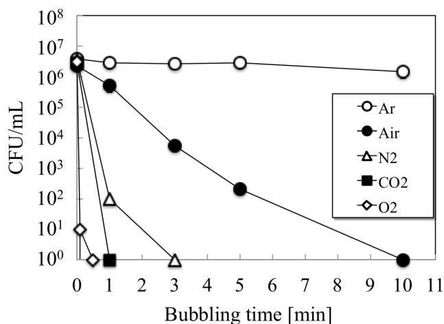
Figure 5-25 E.coli に対するプラズマバブリング法による殺菌効果
