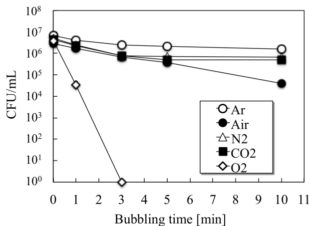
Figure 5-31 プラズマバブリング法による B. safensis の殺菌
