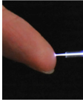
Figure 3-33 マルチガス DBD プラズマジェットで生成したプラズマに触れる様子
