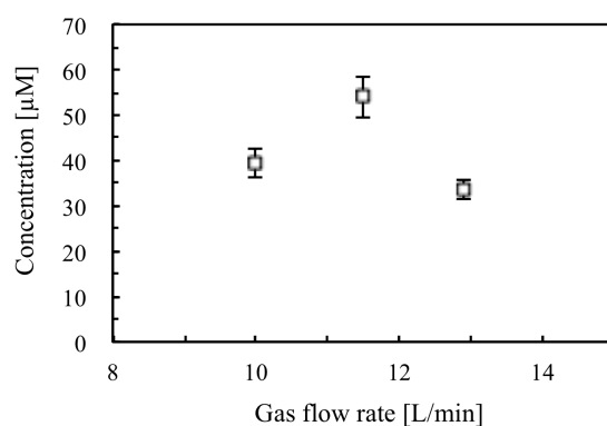
Figure 5-16 ガス流量と ^1\text{O}_2 生成量の関係
