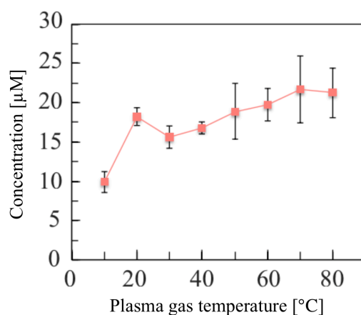
Figure 5-11 OH\cdot 生成量のプラズマガス温度依存性
