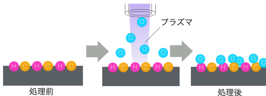
Figure 6-2 プラズマによる官能基付与の模式図
