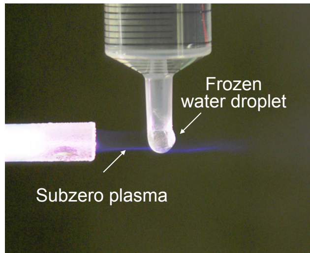
Figure 3-15 零下のプラズマで水滴が氷結する様子
