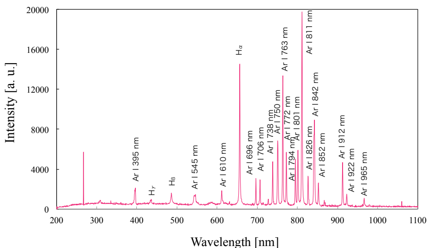
Figure 6-17 水素混合アルゴンプラズマの発光スペクトル
