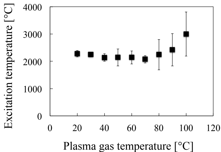
Figure 3-35 マルチガス DBD プラズマジェットにおける ヘリウム励起温度のプラズマガス温度依存性
