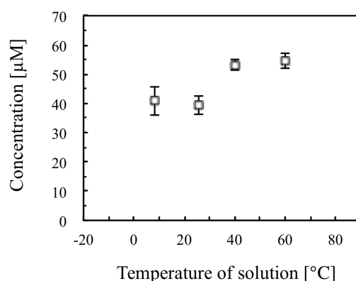
Figure 5-18 水温と ^1\text{O}_2 生成量の関係
