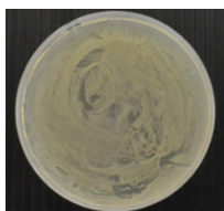
Figure 4-13 65 °Cのガスのみを3分間吹き付けた寒天培地の様子
