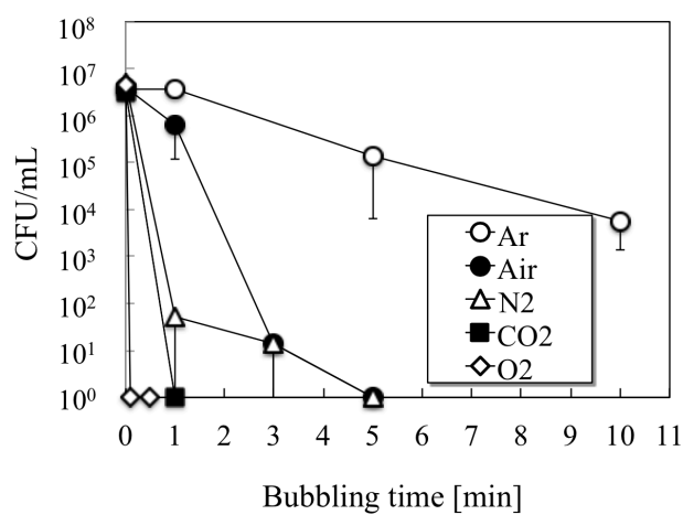
Figure 5-30 プラズマバブリング法による E. faecalis の殺菌
