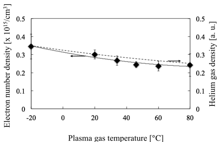
Figure 3-24 電子密度のプラズマガス温度依存性
