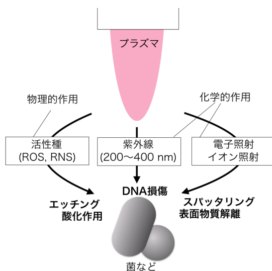
Figure 4-2 プラズマによる殺菌メカニズム
