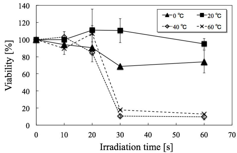
Figure 4-23 NIH3T3-3-4 細胞の生存率とプラズマガス温度の関係
