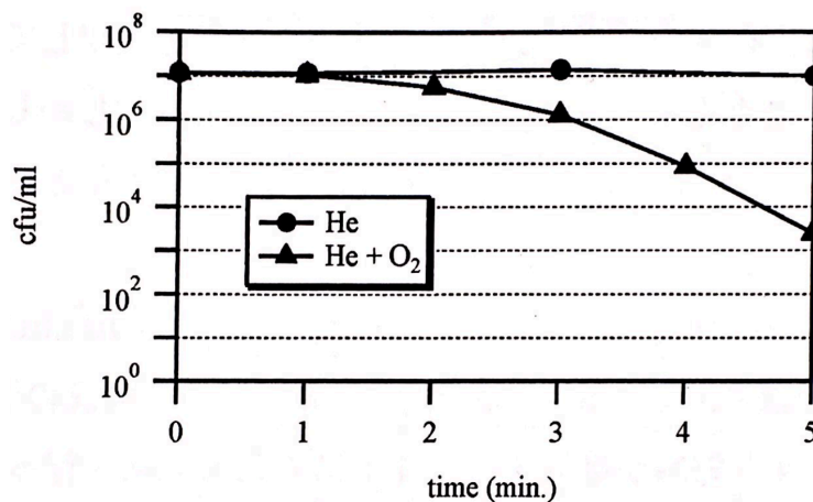
Figure 5-3 大腸菌の殺菌時における雰囲気ガス依存性 [4]
