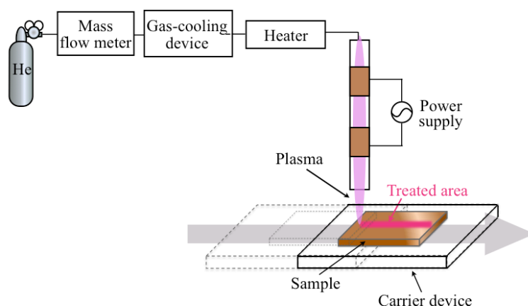
Figure 6-6 親水化実験のセットアップ
