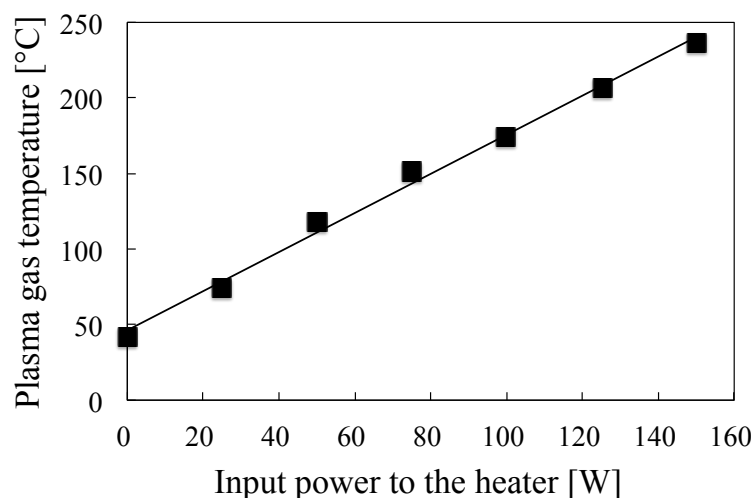
Figure 3-43 高温制御の温度測定
