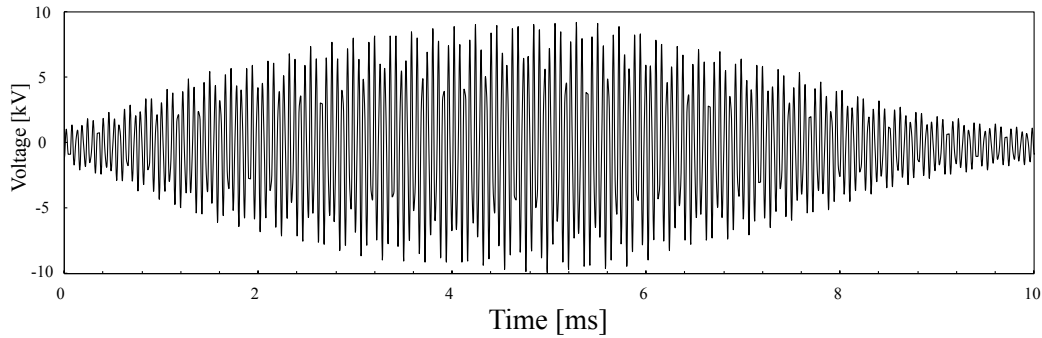
Figure 3-11 電源の開放電圧波形
