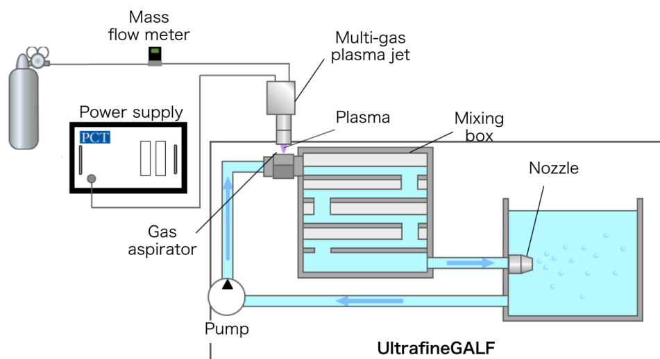
Figure 5-32 プラズマを用いた UFB 生成用実験装置
