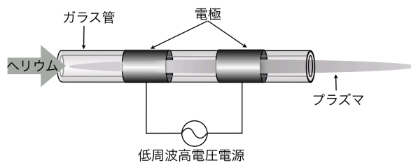
Figure 2-6 マイクロプラズマジェット
