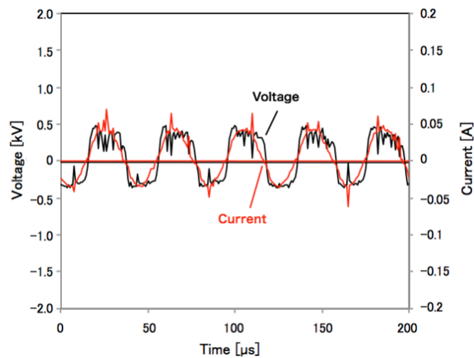
Figure 3-39 マルチガスプラズマジェットで生成したヘリウムプラズマの放電波形の拡大図 [9]
