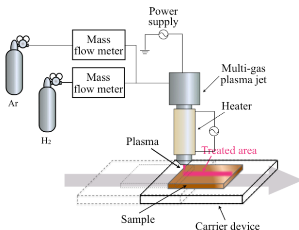
Figure 6-12 酸化膜還元実験のセットアップ
