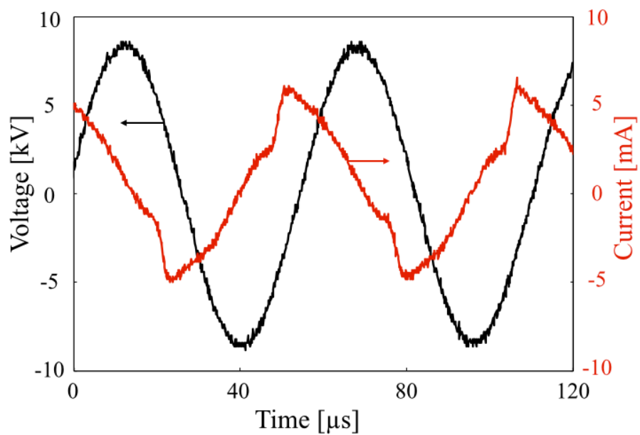
Figure 3-10 9 kV 印加時の放電波形
