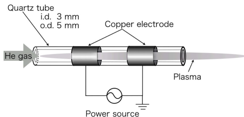
Figure 3-5 本研究で用いたマイクロプラズマジェット
