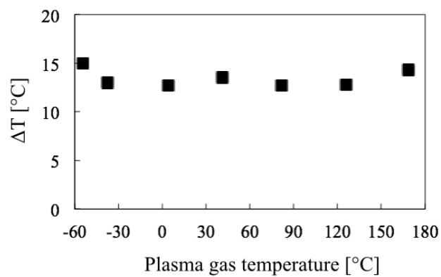
Figure 3-16 プラズマ生成前後の温度変化
