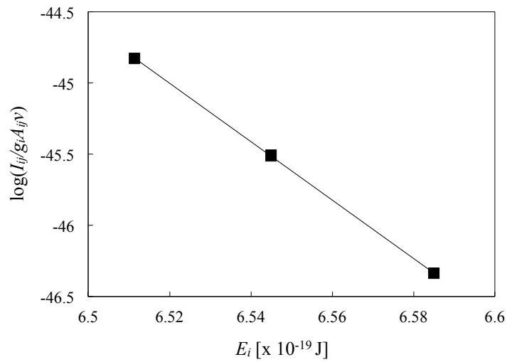
Figure 3-26 熱電対で測定した温度が 40 °C のプラズマにおける OH 回転スペクトルのボルツマンプロット(この時 OH 回転温度は 62 °C)
