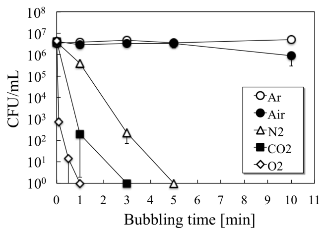
Figure 5-28 プラズマバブリング法による P. aeruginosa の殺菌
