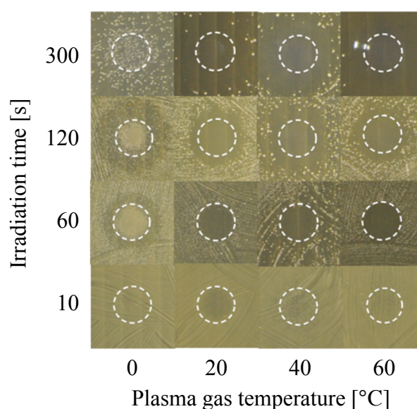
Figure 4-21 殺菌範囲のプラズマガス温度依存性
