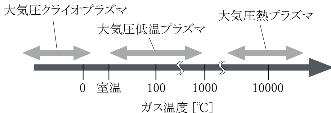
Figure 2-1 ガス温度に着目したときの大気圧プラズマの分類
