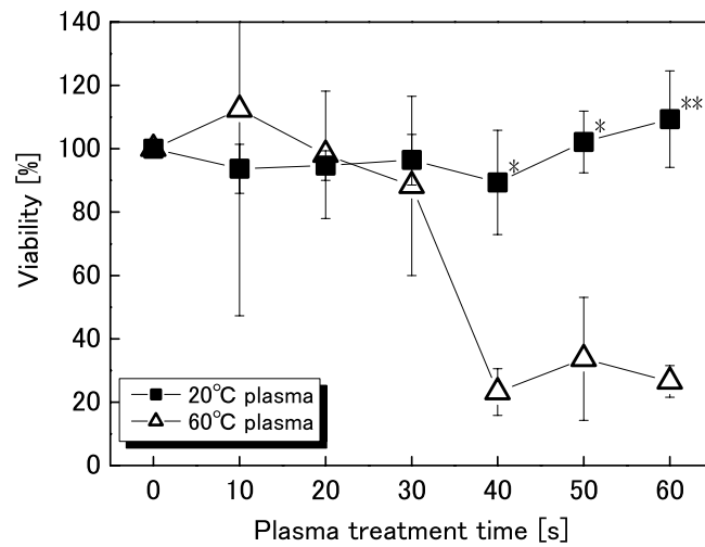
Figure 4-24 アルゴン二酸化炭素混合プラズマ照射後の HeLa 細胞の生存率にプラズマガス温度が与える影響 [13]
