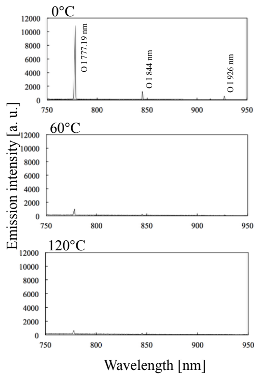
Figure 3-23 ガス温度による赤外光スペクトルの変化
