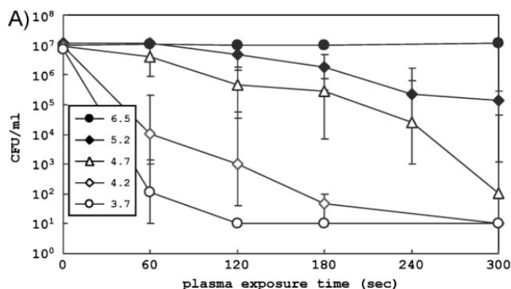
Figure 5-2 大腸菌の殺菌時における pH 依存性 [2]
