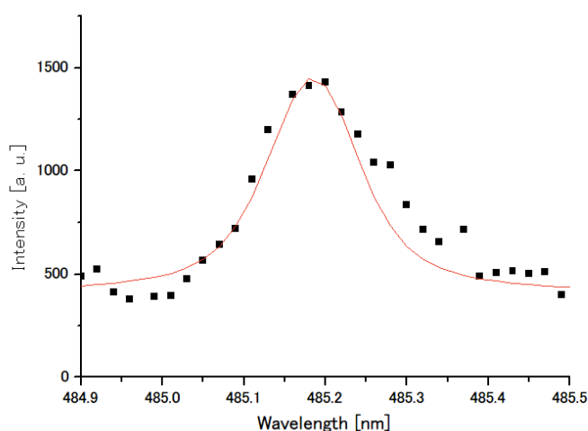
Figure 3-20 20\text{ }^{\circ}\text{C} に制御して生成したプラズマの \text{H}_{\beta} 線のスペクトルをフォークト関数でフィッティングした例
