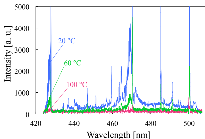
Figure 3-34 マルチガス DBD プラズマジェットのヘリウム発光スペクトルのガス温度による変化
