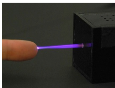
Figure 2-7 放電損傷のないプラズマに手で触れる様子
