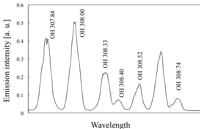
Figure 3-25 熱電対で測定したガス温度が 40 °C のプラズマの OH 回転スペクトル
