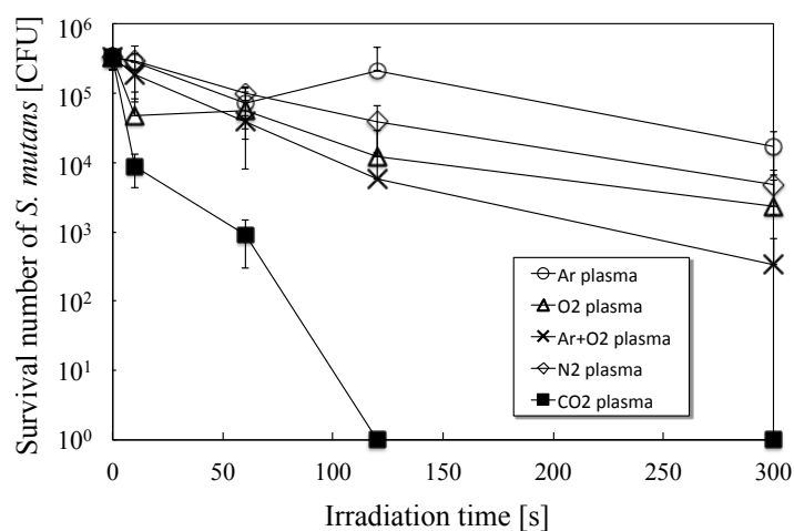
Figure 4-20 ガス種による生存菌数の違い
