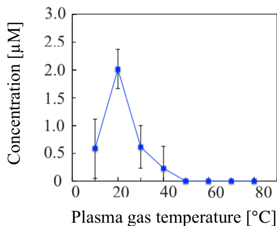
Figure 5-13 O 3 生成量のプラズマガス温度依存性
