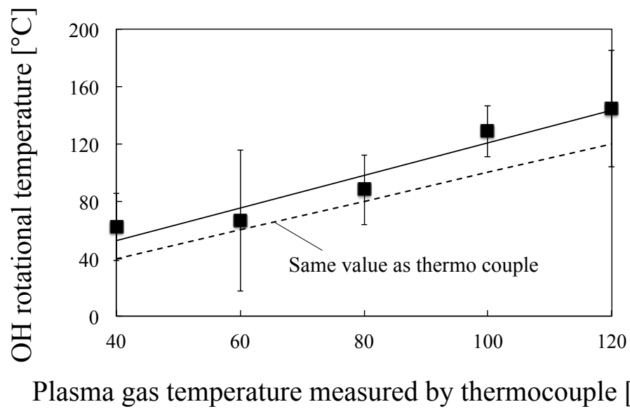
Figure 3-27 熱電対で測定したガス温度と OH 回転温度の関係
