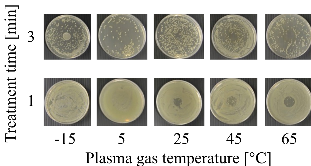
Figure 4-9 殺菌範囲のプラズマガス温度依存性
