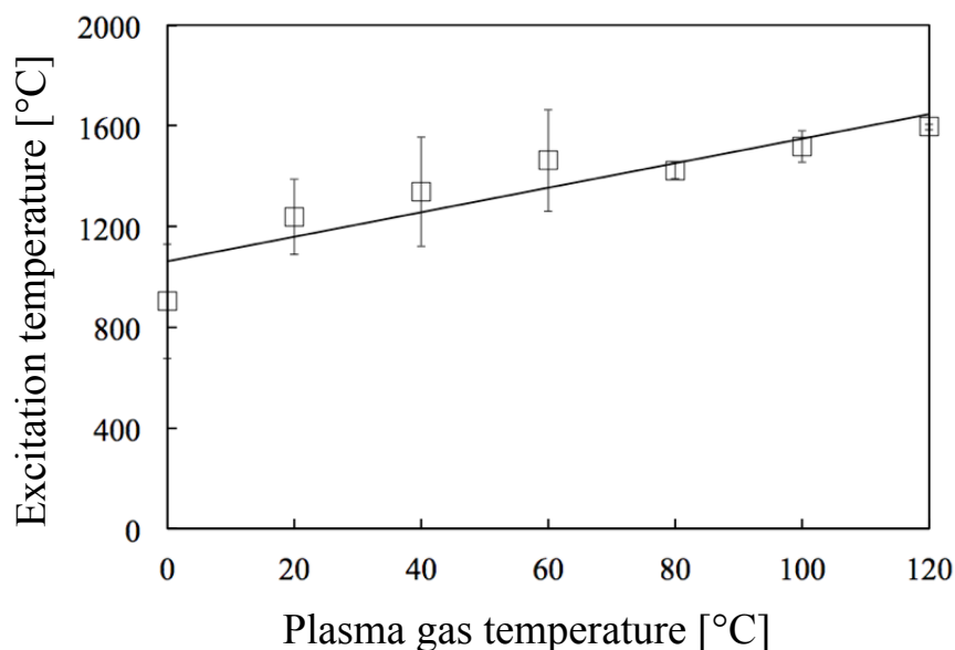
Figure 3-29 ヘリウム励起温度のプラズマガス温度依存
