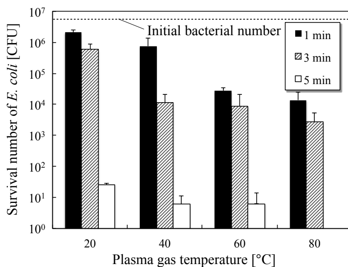
Figure 4-12 寒天培地中央部直径 15 mm の範囲の生存菌数
