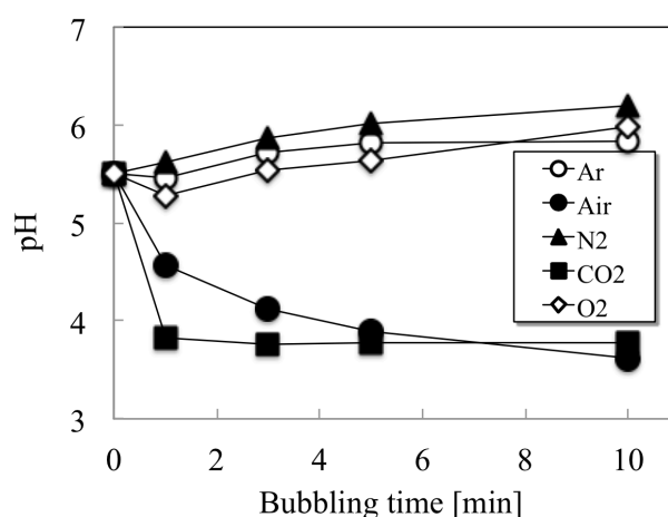
Figure 5-26 プラズマバブリングによる pH の変化
