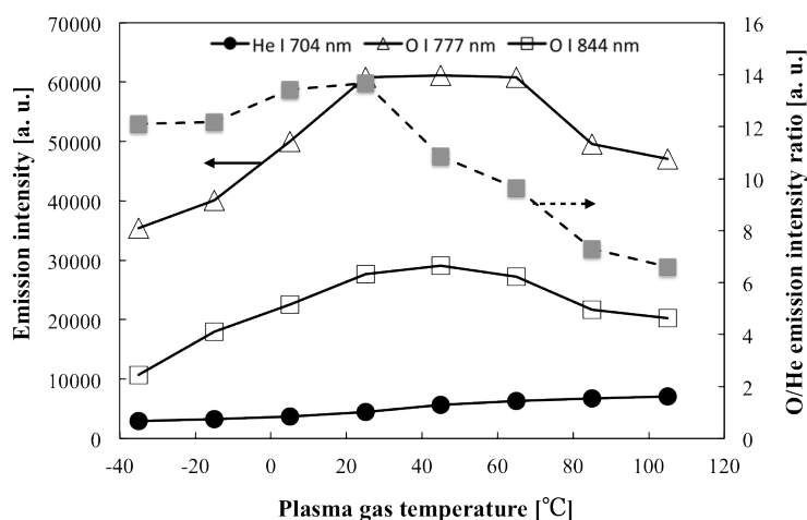
Figure 4-17 プラズマガス温度と発光強度比の関係
