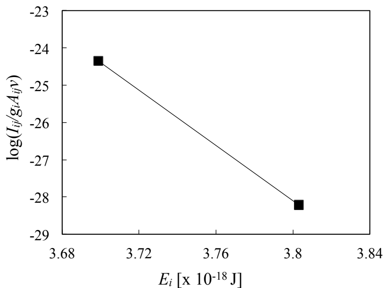
Figure 3-28 40 °Cのプラズマにおけるヘリウム原子線のボルツマンプロット
