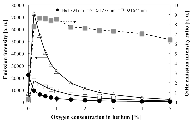
Figure 4-16 酸素混合濃度と発光強度比の関係
