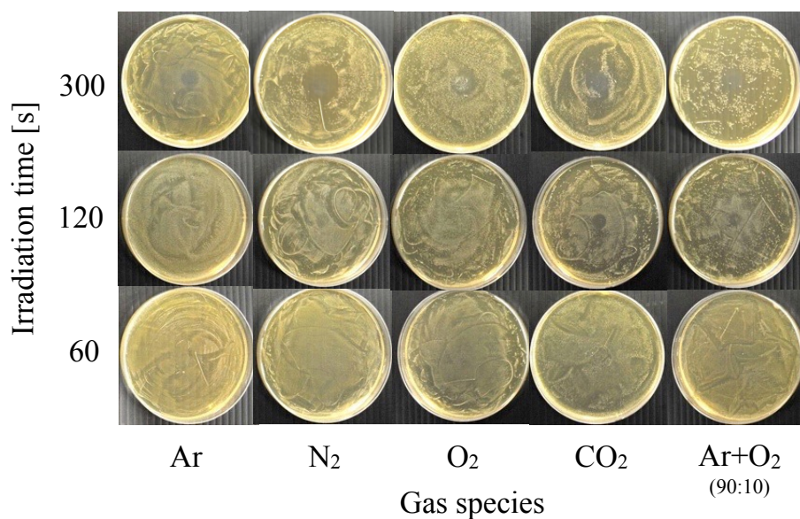
Figure 4-19 殺菌範囲のプラズマガス種依存性
