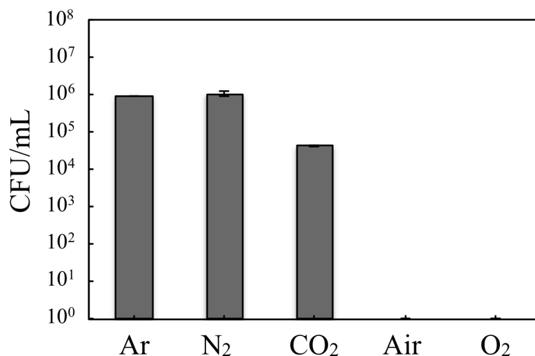
Figure 5-33 プラズマを用いて生成した UFB 水の殺菌効果
