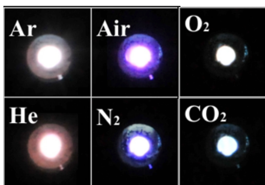
Figure 3-31 マルチガス DBD プラズマジェットで生成したプラズマの様子
