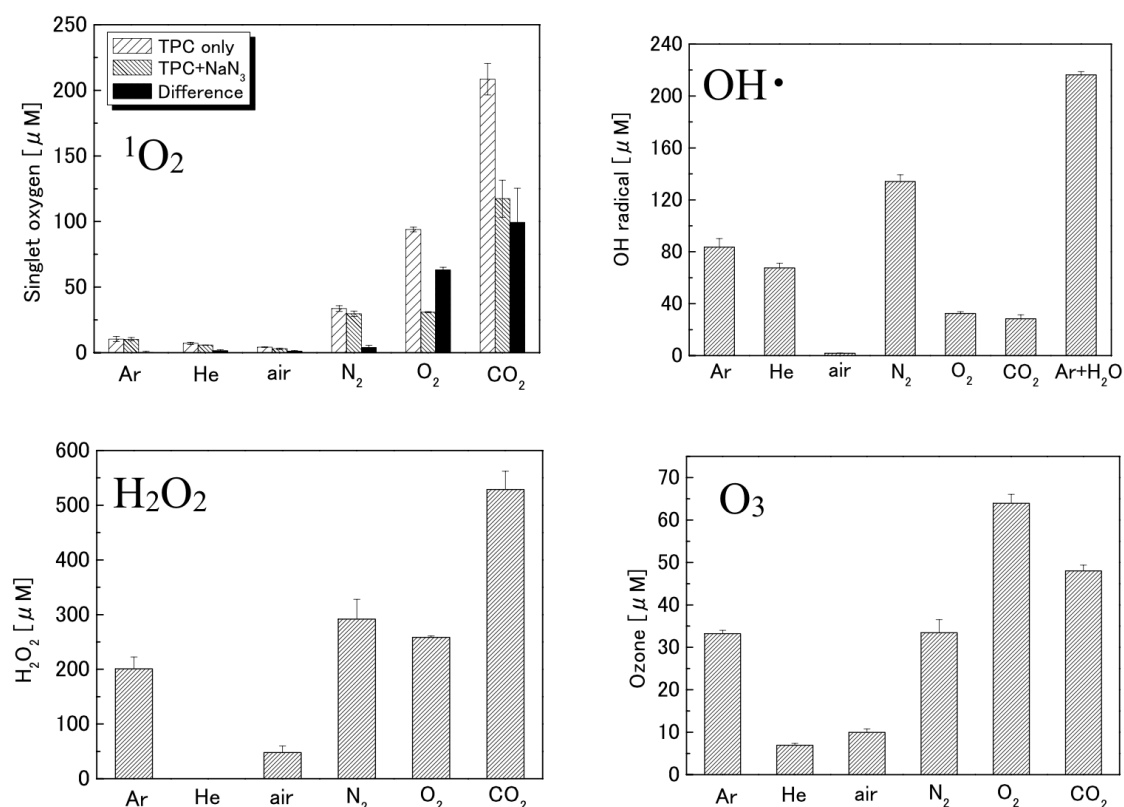
Figure 5-7 活性種生成量のガス種依存性
