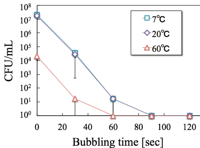
Figure 5-27 水温による殺菌効果の変化
