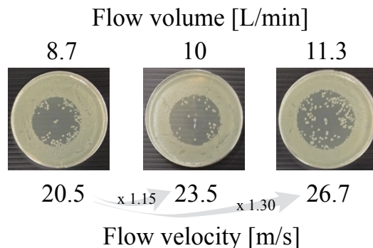
Figure 4-14 ガス流速と殺菌範囲の関係
