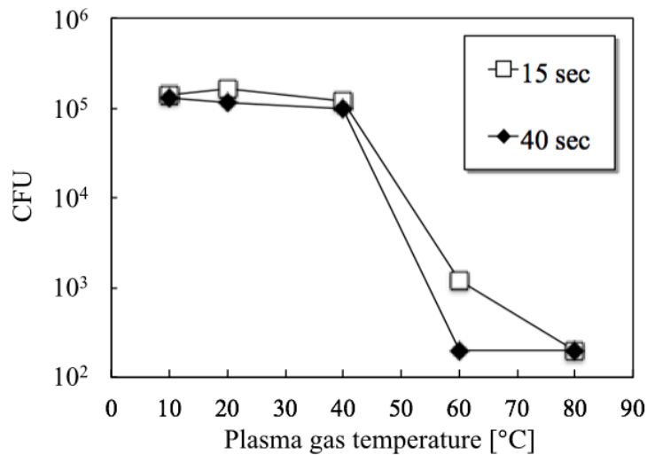
Figure 5-22 液中殺菌効果のプラズマガス温度依存性
