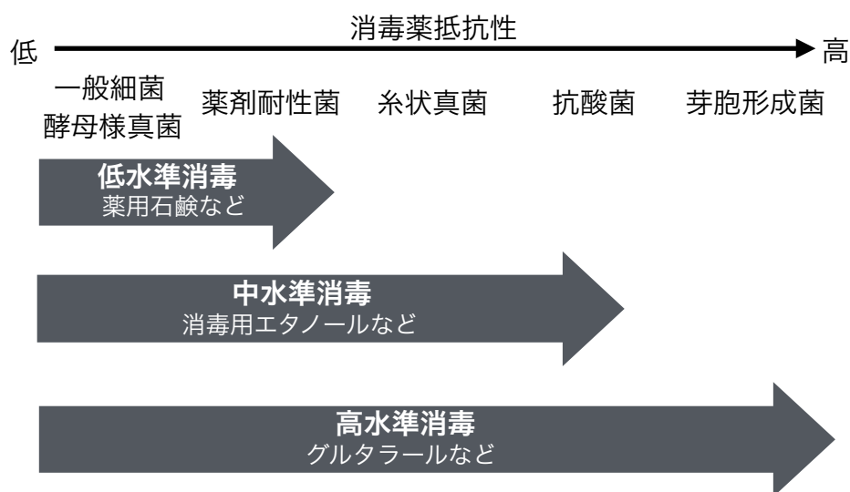
Figure 4-1 微生物の消毒薬抵抗性と消毒薬の作用範囲
