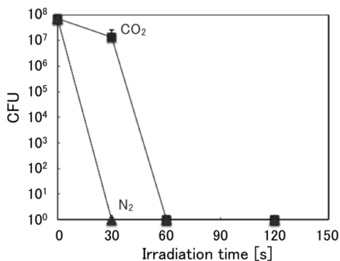
Figure 5-5 MRSA に対する殺菌効果のガス種依存性 [1]
