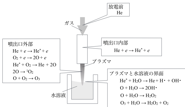
Figure 5-1 ヘリウムプラズマジェットの反応例
