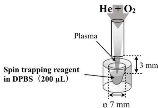
Figure 5-10 活性種測定実験の実験系
