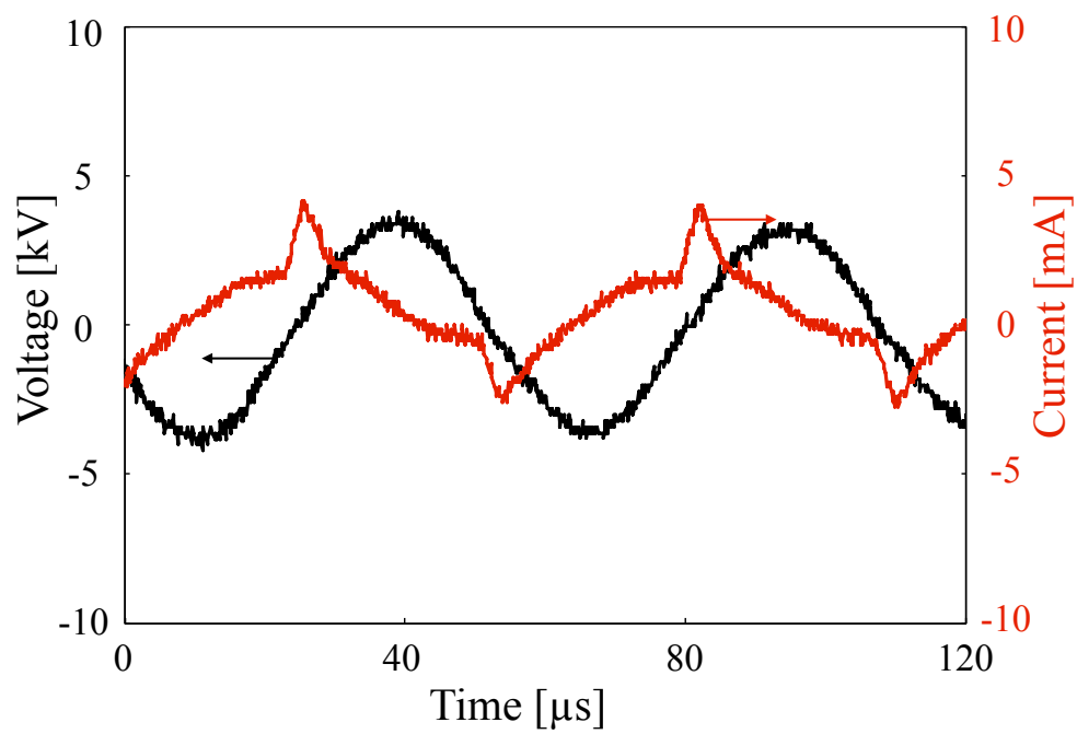
Figure 3-9 4 kV 印加時の放電波形
