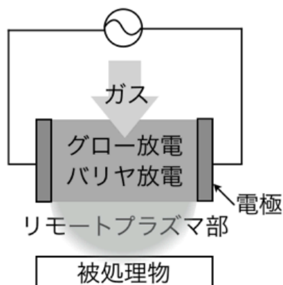
Figure 2-8 リモートプラズマ
