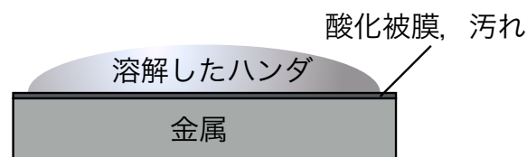
Figure 6-9 酸化した金属表面にハンダ付けした様子
