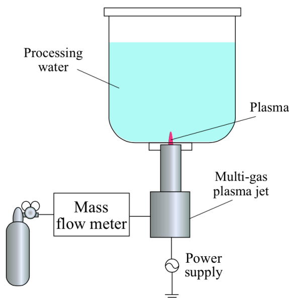
Figure 5-24 プラズマバブリング法の概略図
