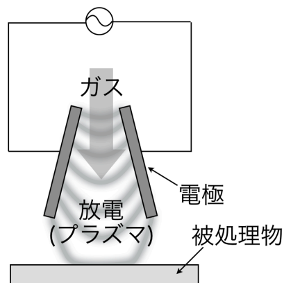
Figure 2-4 コロナ放電プラズマ
