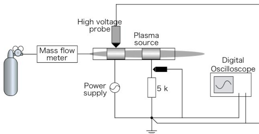
Figure 3-8 電流電圧測定のセットアップ
