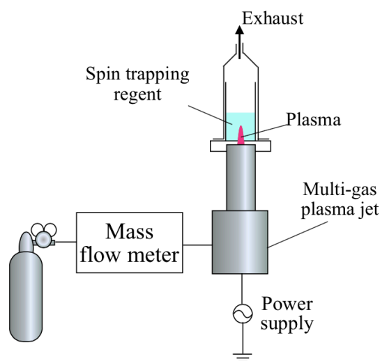
Figure 5-19 空気遮断条件下での活性種測定の実験系
