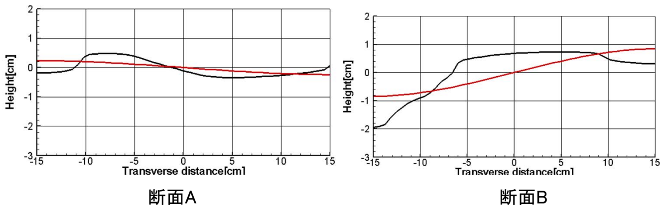
図3-2 横断面形状とそのモード関数化の一例
