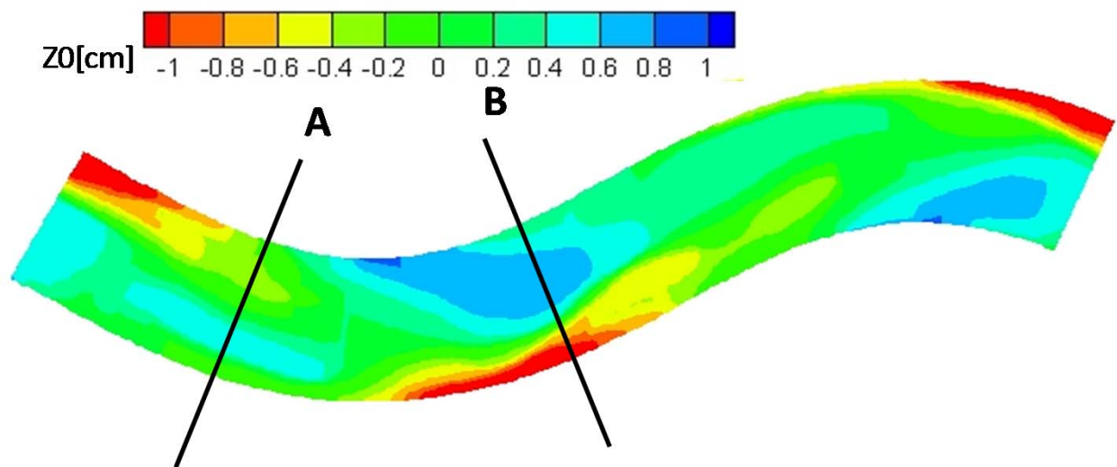
図3-1 蛇行実験水路での安定河床形状
