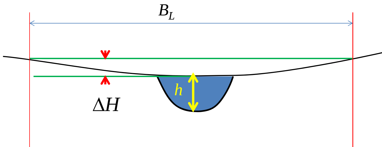
(b) 断面図
