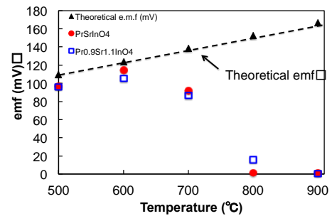
Figure 3. Pr 1-x Sr 1+x InO 4 ( x=0, 0.1 )の水素濃淡電池における起電力
