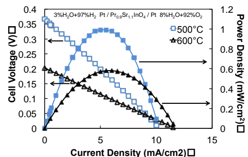
Figure 4. Pr 0.9 Sr 1.1 InO 4 の発電特性
