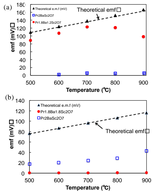
Figure 6. Pr 2-x Ba 1+x Sc 2 O 7 (x=0, 0.2)の(a)水素濃淡電池及び(b)酸素濃淡電池における
