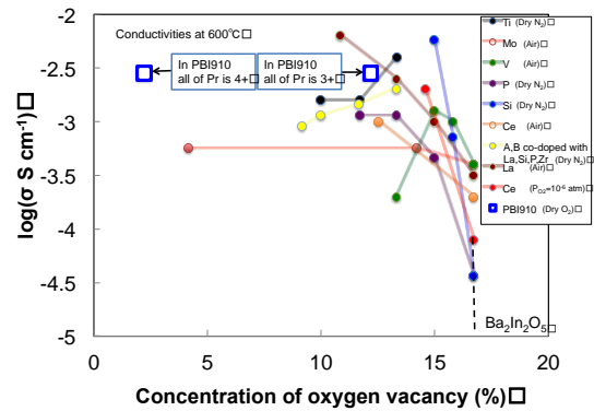
Figure 2. ドーピングしたBa 2 In 2 O 5 系材料の伝導率と酸素欠陥濃度の関係
