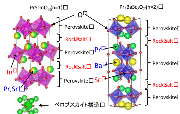
Figure 1. PrSrInO 4 と Pr 2 BaSc 2 O 7 の構造
