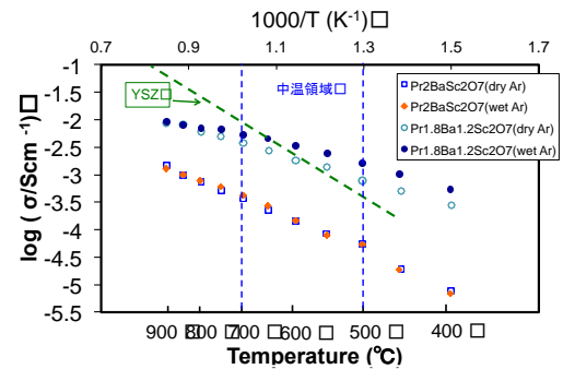
Figure 5. Pr 2-x Ba 1+x Sc 2 O 7 (x=0, 0.2) の wet, dry Ar における伝導率
