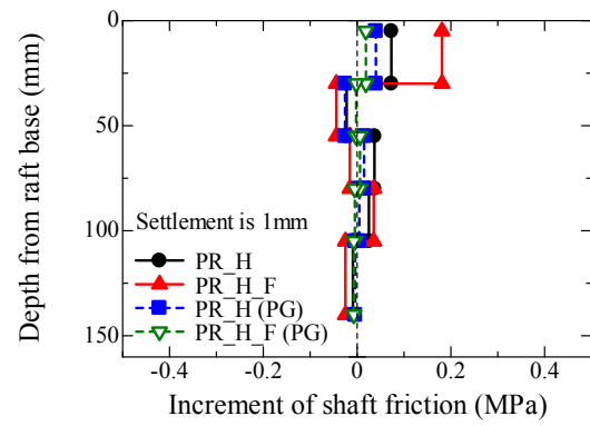
(d) Heavy case (Increment value)
