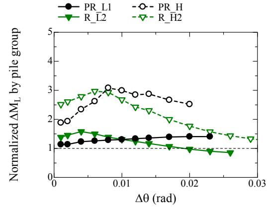
(d) \delta_{LDT} = \pm 2\text{mm} , h/S=1.8
