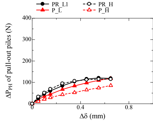
(d) Pull-out piles ( \delta_{LDT} = \pm 1 \text{ mm} , h/S=1.8 )
