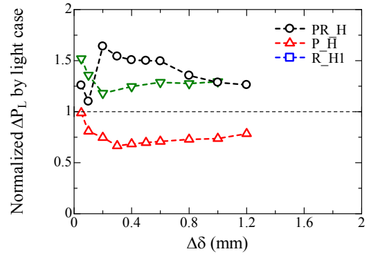
(d) \delta_{LDT} = \pm 2 \text{ mm} , h/S=1.8
