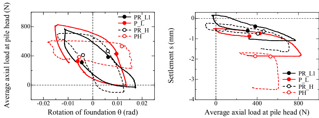
(d) Axial load at pile head (Right pile)
