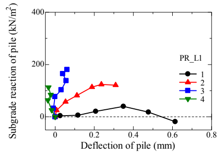
(d) Pull-out pile ( \delta_{LDI} = \pm 1 \text{ mm} , h/S=1.8 )
