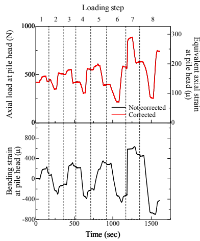
(d) Pile 3 (P_H)
