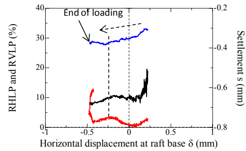
(d) Loading step 4 ( \delta_{LDT} = -1\text{mm} , h/S = 1.8 )
