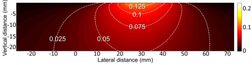
Figure 4.6 L-mode ABR using \theta_{PA} = 16^\circ .
