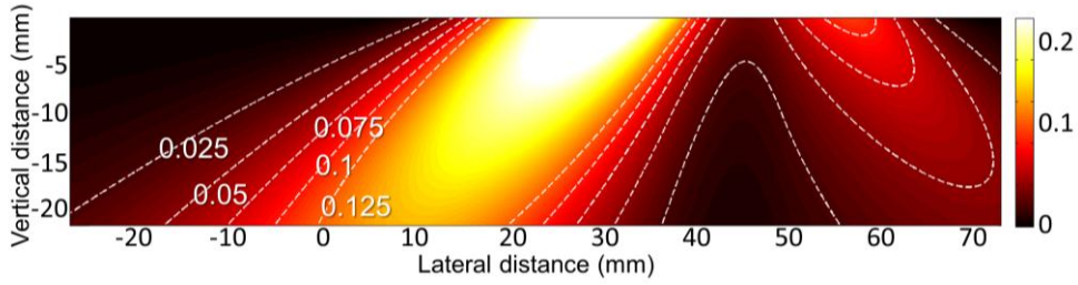
Figure 4.7 T-mode ABR using \theta_{PA} = 38^\circ .
