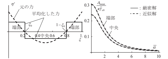
図 22 静的水平力の平均化の概念
