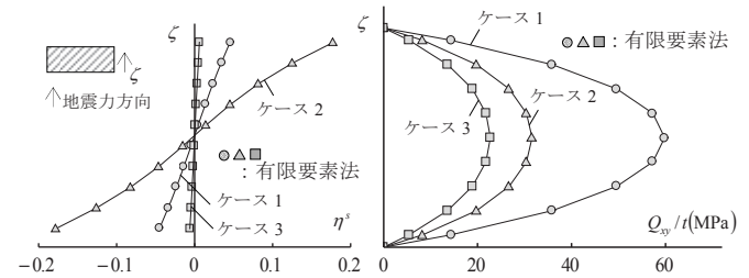
図 30 検討直交方向の静的水平力
