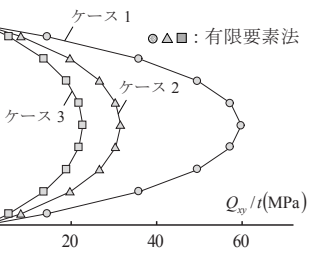
図 31 天井面最大せん断応力
