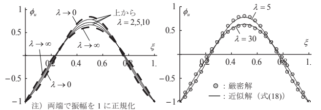
図 12 2 次振動モードの変化
