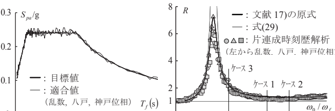
図32 地震応答スペクトル
