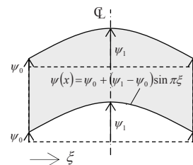
図 27 屋根面の変形仮定
