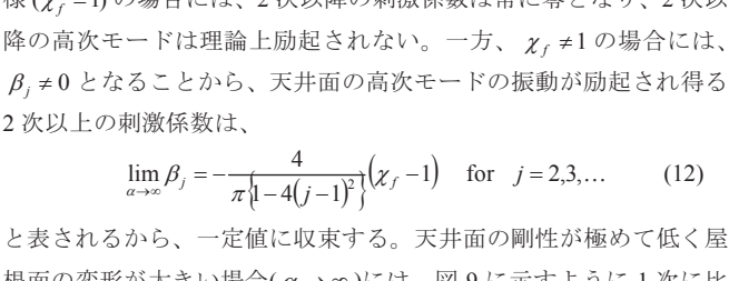
図 8 2 次以降の刺激係数
