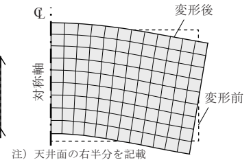
図 28 2次振動モード(有限要素法)
