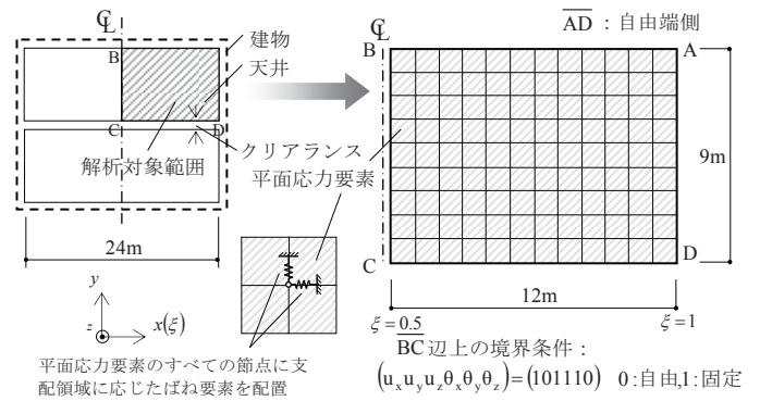
図 26 天井の地震応答解析モデル
