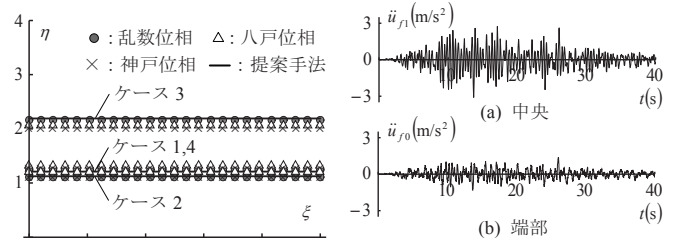
図34 水平力(一様加速度)
