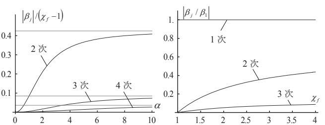
図 6 天井面の静的振幅比
