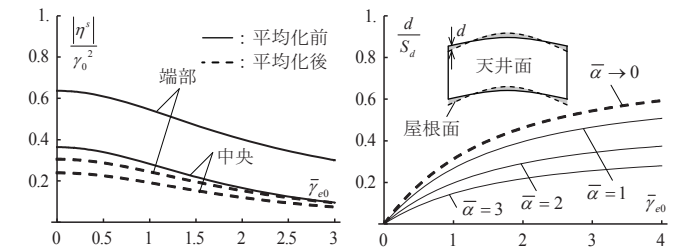
図 24 平均化した静的水平力
