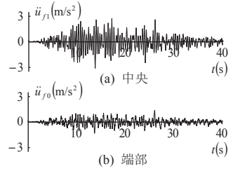
図35 天井への入力の例(乱数)
