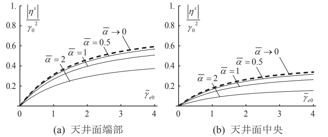
図19 静的水平力と建物の剛比の関係
