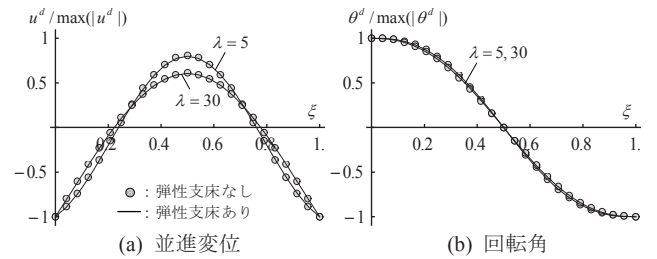
図 10 弾性支床が 2 次モードの変化に及ぼす影響
