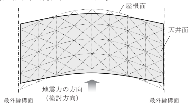
図1 屋根面および天井面の地震時変形
