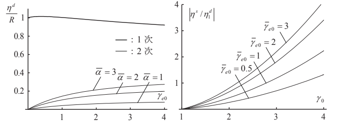
図 20 動的水平力
