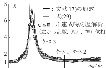
図33 床応答加速度の比較
