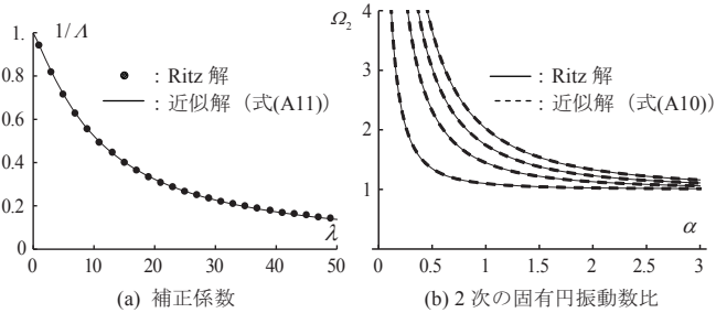
付図 2 2 次固有円振動数の近似式の精度
