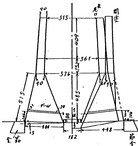
價谷鑪（銑押）
