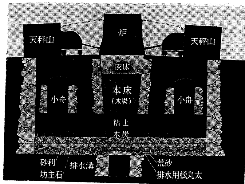
図 2 - 2 日刀保たたら地下構造図
