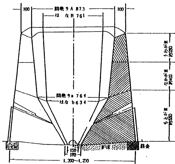
図7-2 各たたら炉の外観比較
