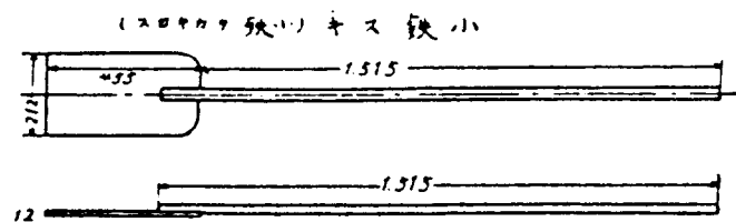
図3-7 小鉄スキ
