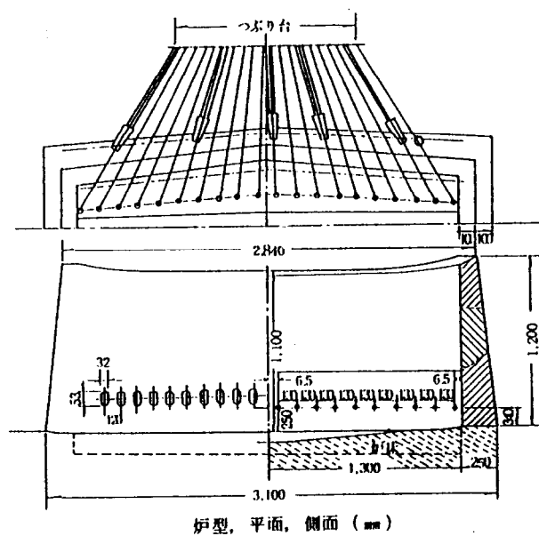
図 3 - 11 日刀保たたら炉型断面図・平面図・側面図
