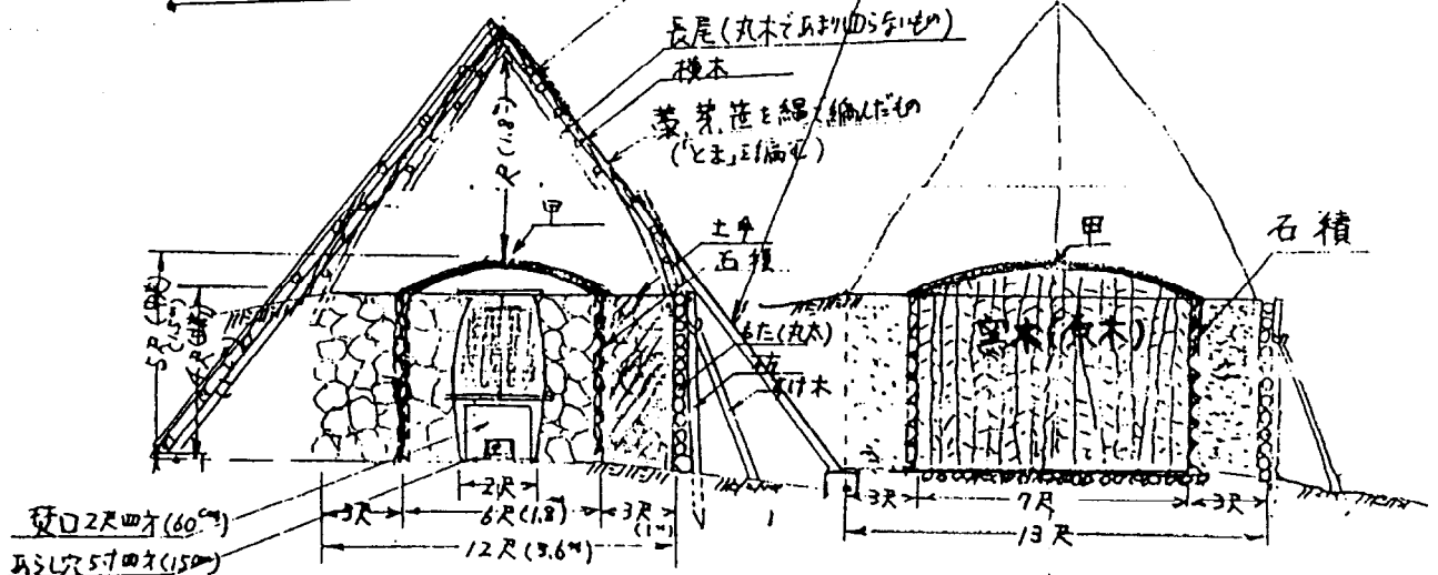
※2図 正面図(A-A)
