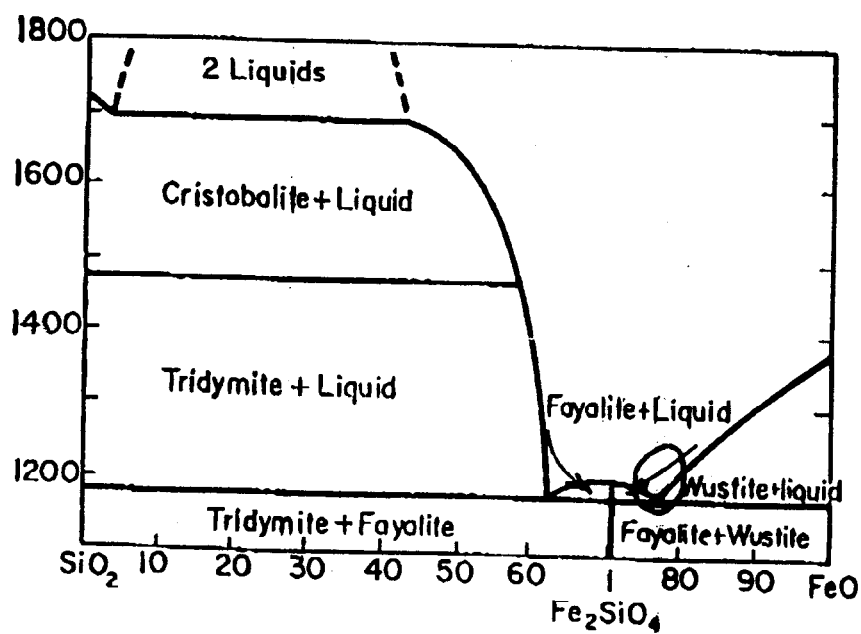
图 6-6 \text{FeO-SiO}_2 二元状态图
