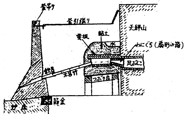
図3-12 日刀保たたらをつぶり台・木呂管などの据え付け
