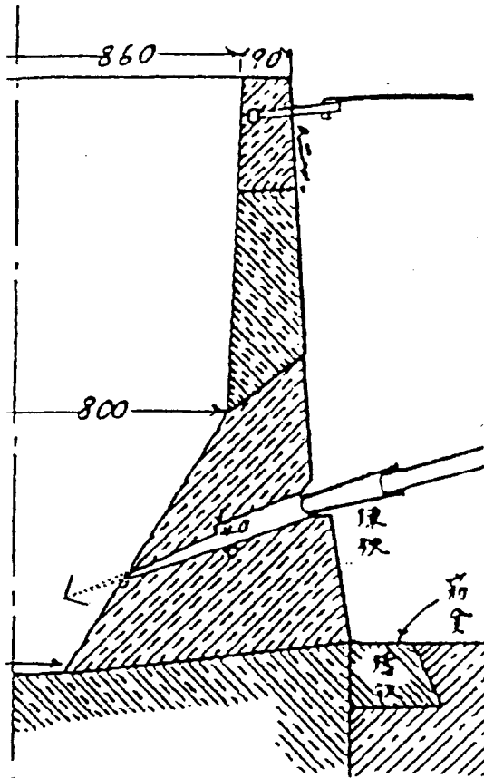
図7-6 砥波鑪（鋸押）の炉とホド穴の断面図
