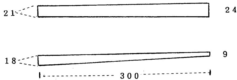
図7-5 鋤押し法と鉄押し法におけるホドの形状と法量の比較 単位：mm
