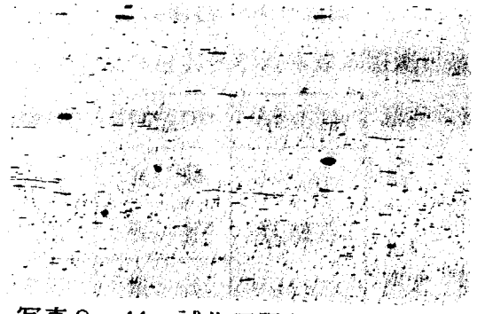
写真 8-11 試作刀隅谷の介在物
