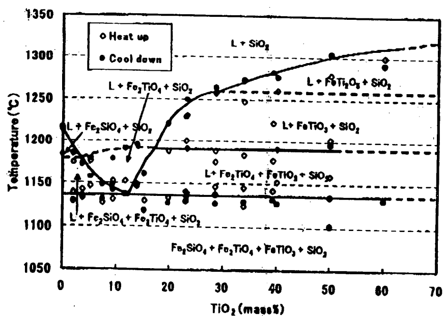
图 6-5 \text{Fe}_2\text{SiO}_4\text{-TiO}_2 拟二元系状态图
