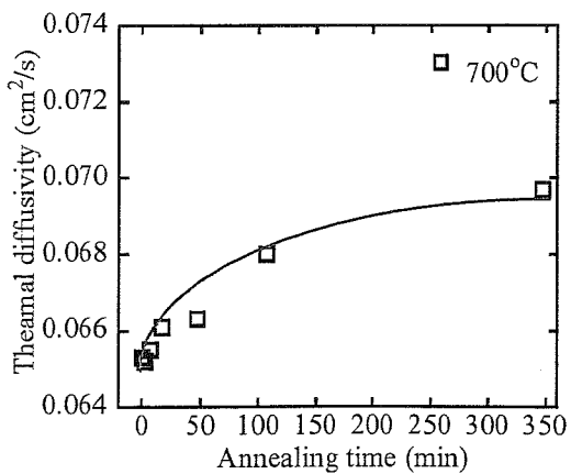
Fig.3.33-a x 軸は保持時間
