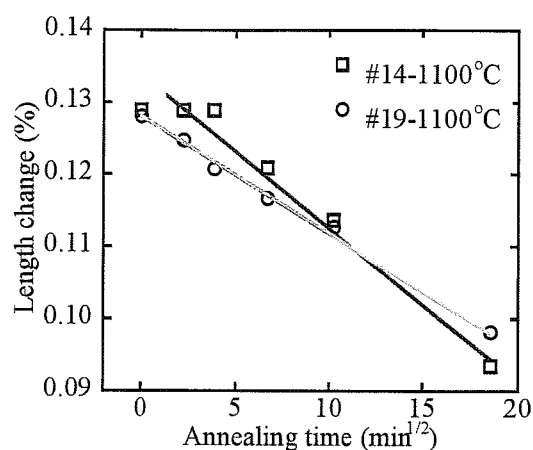
Fig.2.20-b x 軸は保持時間の 1/2 乗
