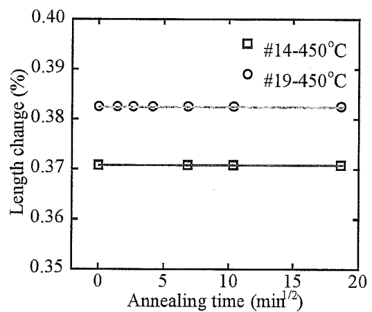
Fig.2.7-b x 軸は保持時間の 1/2 乗
