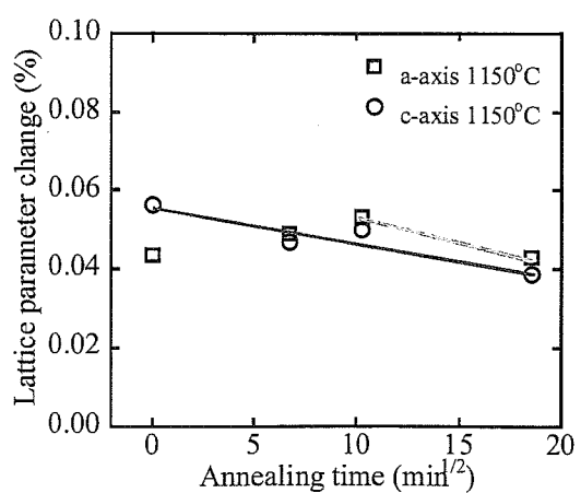
Fig.4.21-b x 軸は保持時間の 1/2 乗
