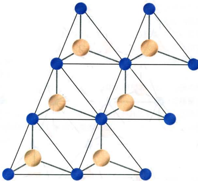
Fig.1.5-a 3C-SiC における、 \text{SiC}_4 ( \text{CSi}_4 ) 四面体の積み重ね 上図：四面体を上から見た場合、「同一方向」に並んで積層している。 下図：横から見た場合でも同様に、「同一方向」にならんで積層している。
