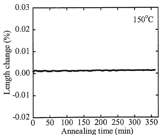
Fig.5.3-1-a Al 2 O 3 添加 SiC
