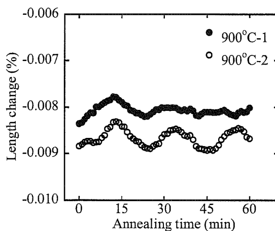
Fig.6.1-16 900°C アニール
