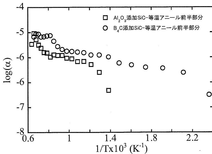
Fig.5.7-3 等温アニール前半部分の変化より求めた両試料のアレニウスプロット
