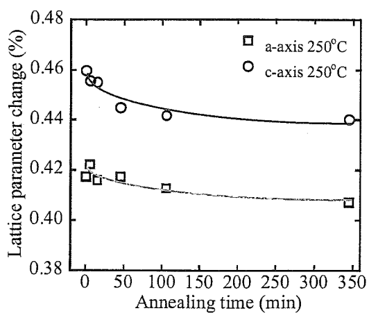
Fig.4.3-a x 軸は保持時間
