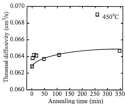
Fig.3.1-a x 軸は保持時間
