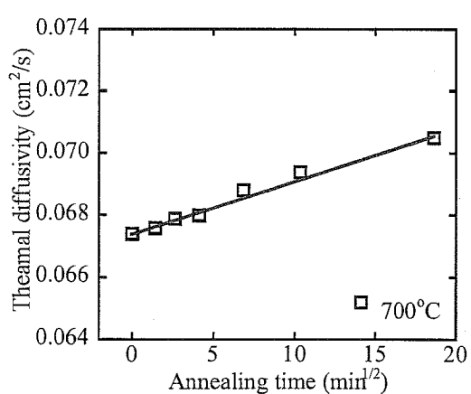
Fig.3.6-b x 軸は保持時間の 1/2 乗
