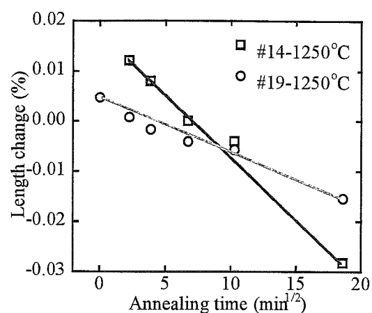
Fig.2.23-b x 軸は保持時間の 1/2 乗
