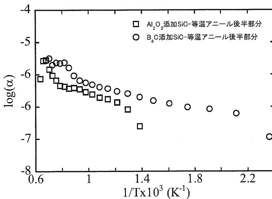
Fig.5.7-4 等温アニール後半部分の変化より求めた両試料のアレニウスプロット
