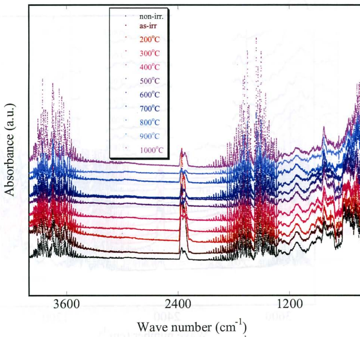
Fig6.5-2 中性子照射 Si (照射量 : 6.9 \times 10^{23} n/m 2 、照射温度 : 300°C) の測定範囲 全域
