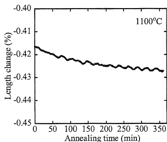
Fig.5.3-20-b \text{B}_4\text{C} 添加 SiC
