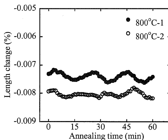
Fig.6.1-14 800°C アニール
