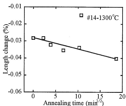
Fig.2.24-b x 軸は保持時間の 1/2 乗
