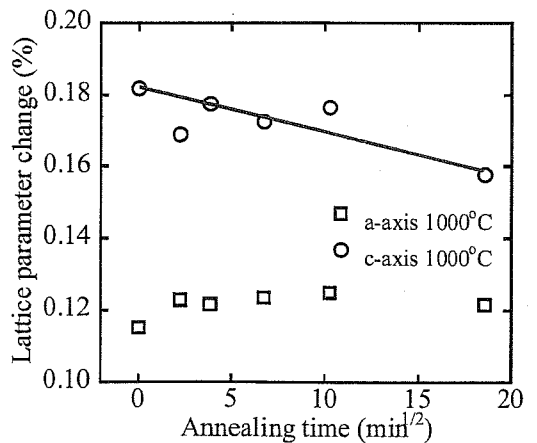
Fig.4.18-b x 軸は保持時間の 1/2 乗
