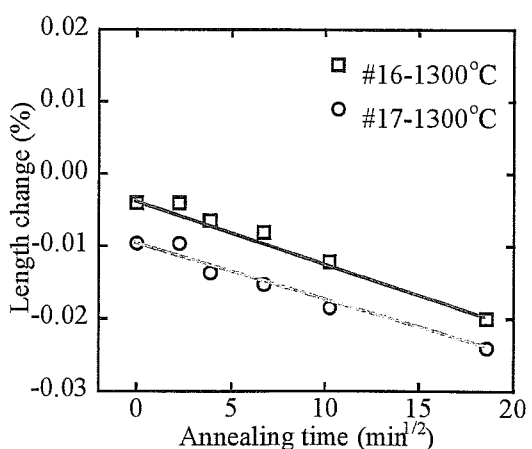
Fig.2.50-b x 軸は保持時間の 1/2 乗
