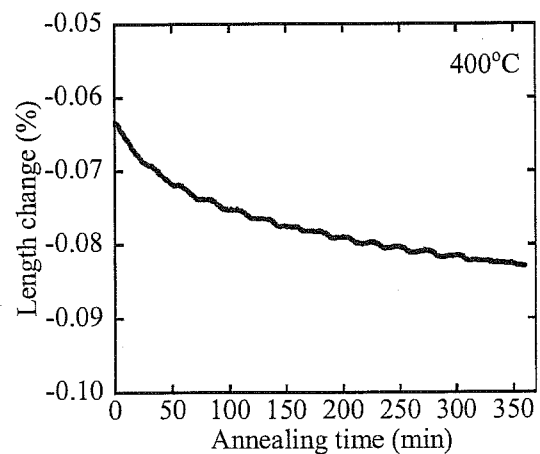
Fig.5.3-6-b B 4 C 添加 SiC
