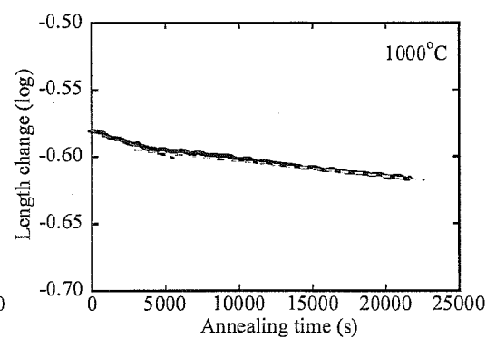
Fig.5.5-12 1000°C アニール
