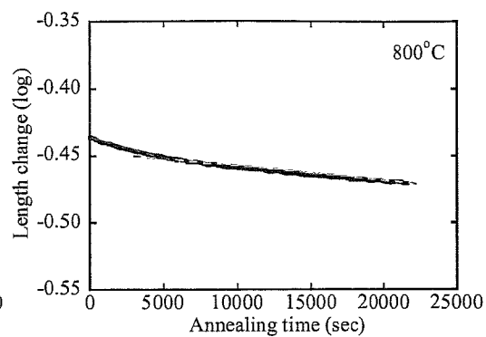
Fig.5.5-8 800°C アニール
