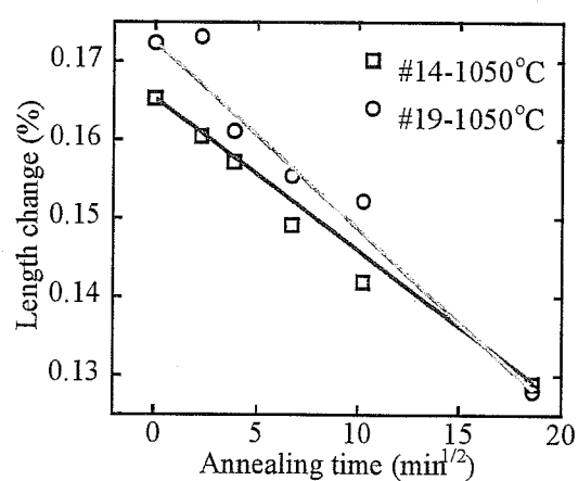
Fig.2.19-b x 軸は保持時間の 1/2 乗
