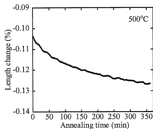
Fig.5.3-8-b \text{B}_4\text{C} 添加 SiC
