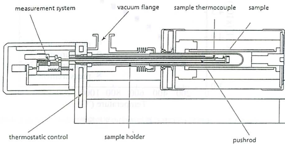
Fig.5.1-4 熱膨張計 本体構造
