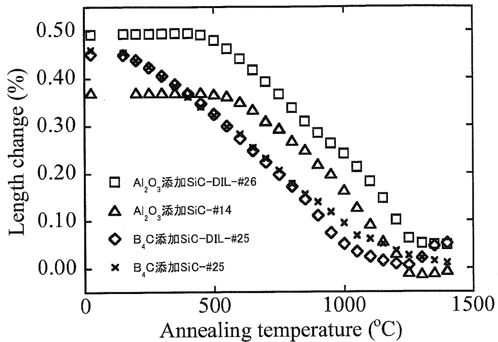
Fig.5.4-1 熱膨張率変化から求めた保持時間 360 分における、等時アニールによる巨視的寸法変化と、第二章で求めた巨視的寸法変化（試料は、Al 2 O 3 添加 SiC：試料番号 14、B 4 C 添加 SiC：試料番号 17、それぞれ高温での未照射試料における収縮を補正した後の値）
