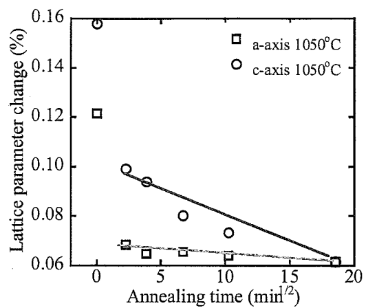
Fig.4.19-b x 軸は保持時間の 1/2 乗
