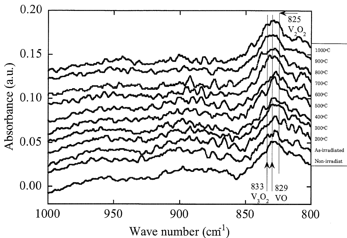
Fig.6.4-3 中性子照射 Si (照射量 : 6.9 \times 10^{23} \text{ n/m}^2 、照射温度 : 300^\circ\text{C} ) の赤外吸収スペクトル (下から順に、未照射、照射直後、アニール温度 200、300、400、500、600、700、800、900、 1000^\circ\text{C} )
