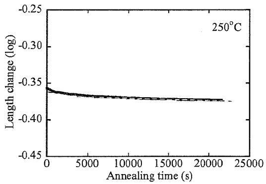
Fig.5.6-3 250°C アニール
