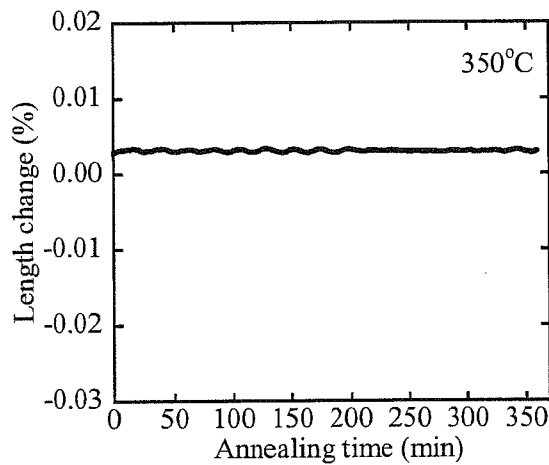
Fig.5.3-5-a Al 2 O 3 添加 SiC
