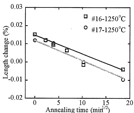
Fig.2.49-b x 軸は保持時間の 1/2 乗
