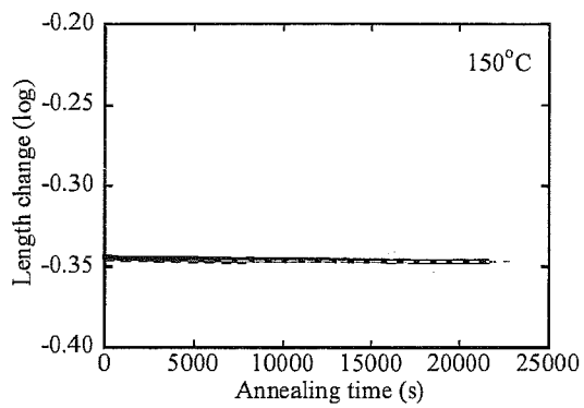
Fig.5.6-1 150°C アニール
