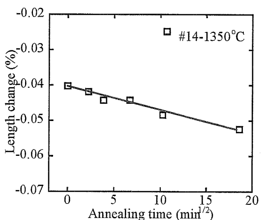
Fig.2.25-b x 軸は保持時間の 1/2 乗
