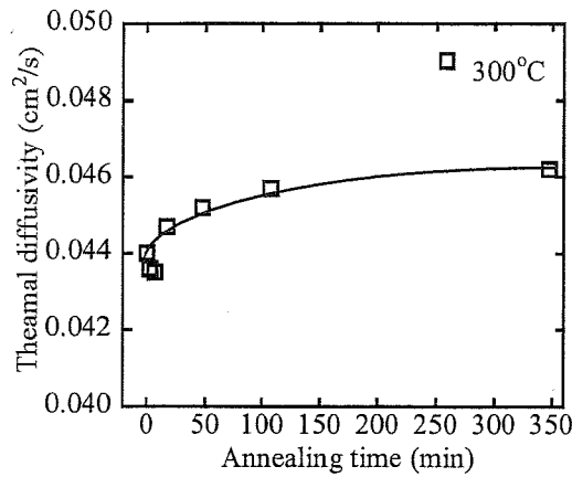
Fig.3.25-a x 軸は保持時間
