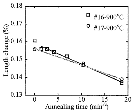
Fig.2.42-b x 軸は保持時間の 1/2 乗
