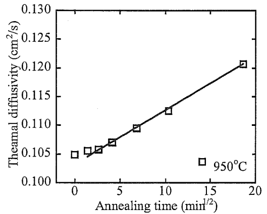
Fig.3.38-b x 軸は保持時間の 1/2 乗
