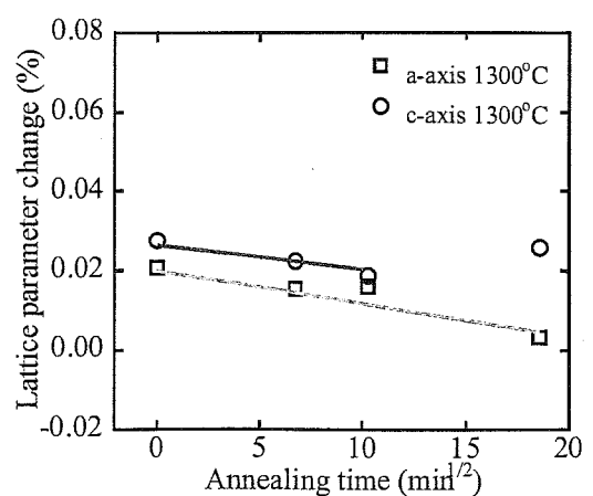
Fig.4.24-b x 軸は保持時間の 1/2 乗
