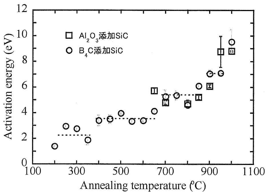
Fig.2.56 巨視的寸法変化の等時、等温アニールより求めた回復の活性化エネルギー
