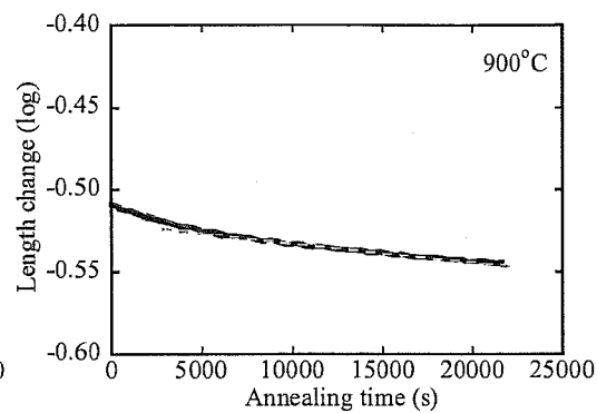
Fig.5.5-10 900°C アニール
