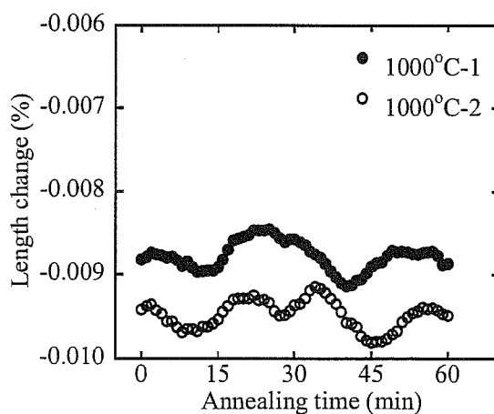
Fig.6.1-18 1000°C アニール
