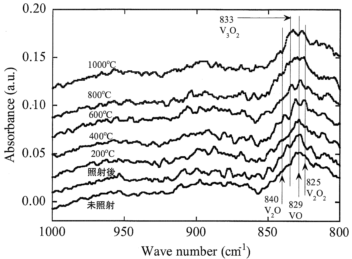
Fig.6.4-2 中性子照射 Si (照射量 : 3.0 \times 10^{23} \text{ n/m}^2 、照射温度 : 120 \sim 150^\circ\text{C} ) の赤外吸収スペクトル (Fig.6.4-1 から間引きしたもの) (下から順に、未照射、照射直後、アニール温度 200^\circ\text{C} 、 400^\circ\text{C} 、 600^\circ\text{C} 、 800^\circ\text{C} 、 1000^\circ\text{C} )
