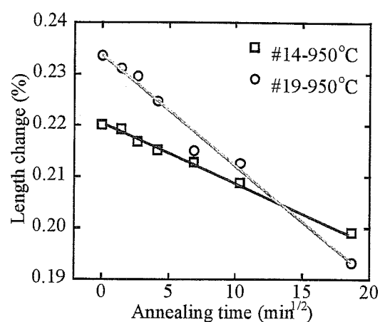
Fig.2.17-b x 軸は保持時間の 1/2 乗
