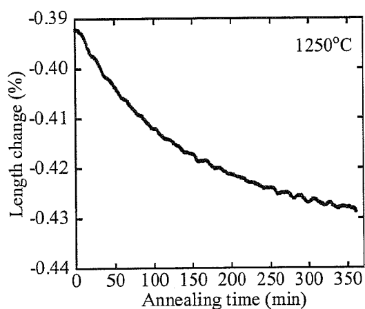
Fig.5.3-23-a Al 2 O 3 添加 SiC
