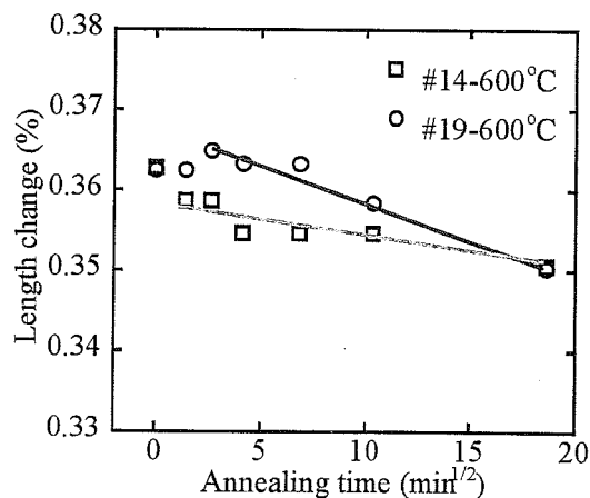
Fig.2.10-b x 軸は保持時間の 1/2 乗
