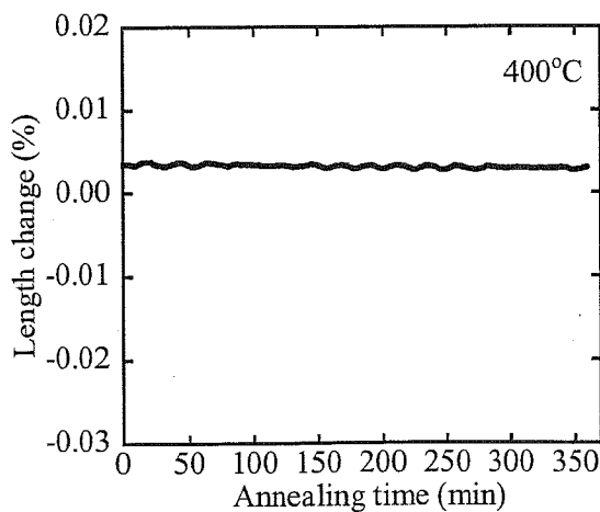
Fig.5.3-6-a Al 2 O 3 添加 SiC
