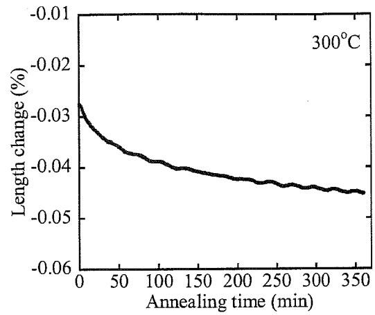
Fig.5.3-4-b B 4 C 添加 SiC
