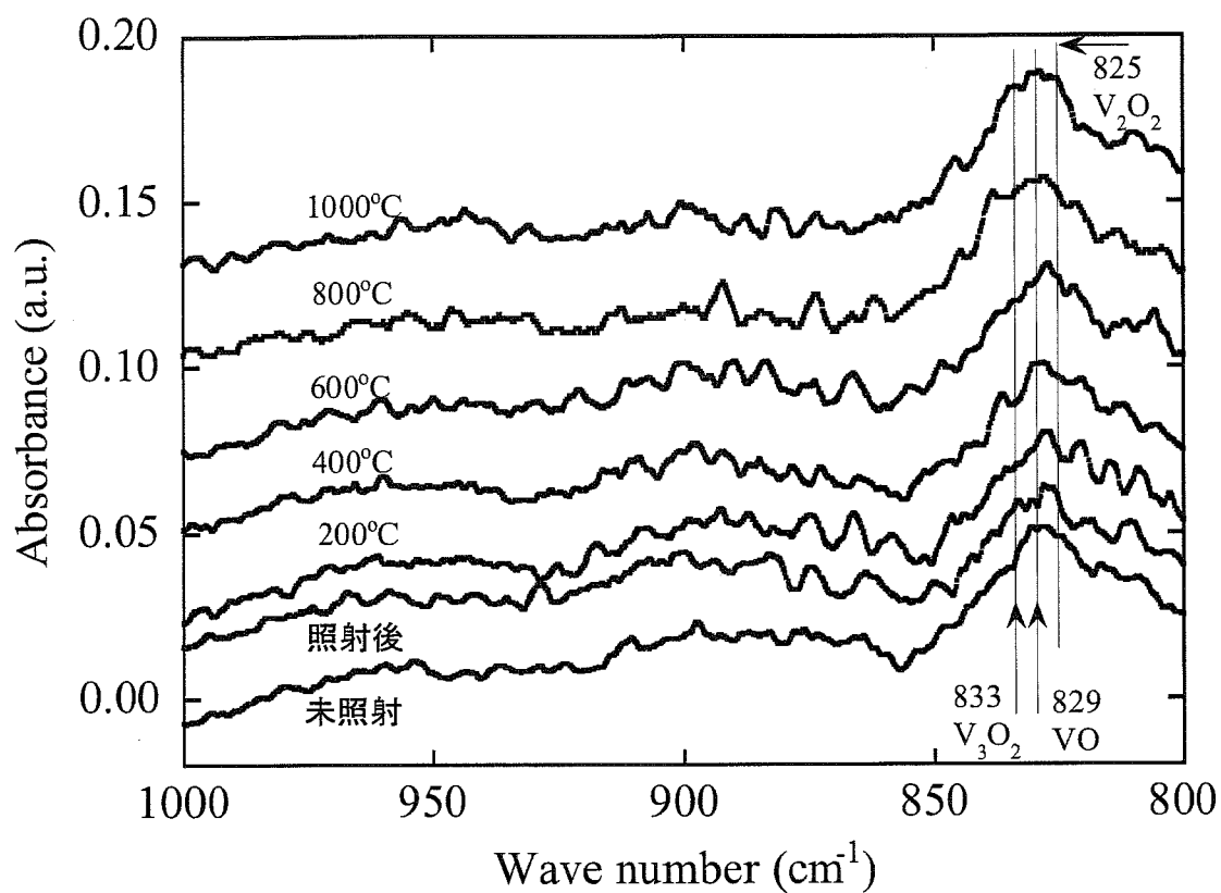
Fig.6.4-4 中性子照射 Si (照射量 : 6.9 \times 10^{23} \text{ n/m}^2 、照射温度 : 300^\circ\text{C} ) の赤外吸収スペクトル (Fig.6.4-3 から間引きしたもの)
