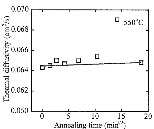
Fig.3.3-b x 軸は保持時間の 1/2 乗
