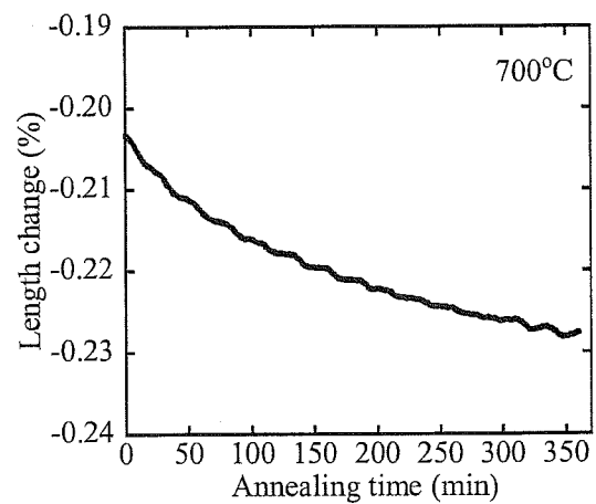
Fig.5.3-12-b \text{B}_4\text{C} 添加 SiC
