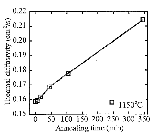
Fig.3.15-a x 軸は保持時間
