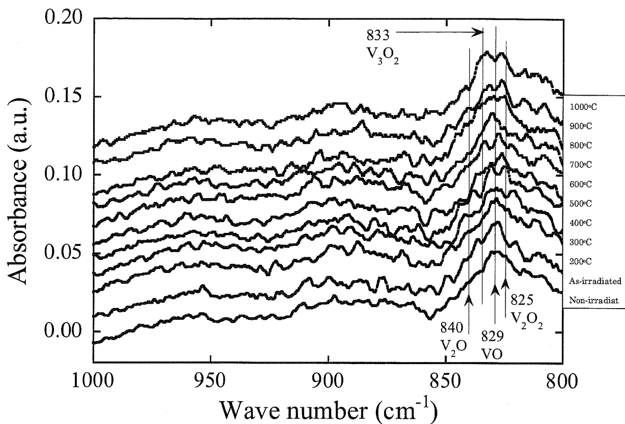
Fig.6.4-1 中性子照射 Si (照射量 : 3.0 \times 10^{23} \text{ n/m}^2 、照射温度 : 120 \sim 150^\circ\text{C} ) の赤外吸収スペクトル (下から順に、未照射、照射直後、アニール温度 200、300、400、500、600、700、800、900、1000°C)
