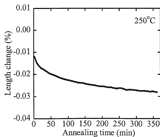
Fig.5.3-3-b B 4 C 添加 SiC
