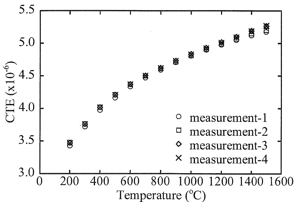
Fig.5.2-2 未照射α-SiC(B₄C添加試料)の平均線熱膨張率 (繰り返し4回測定)
