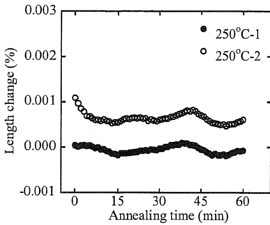
Fig.6.2-3 250°C アニール
