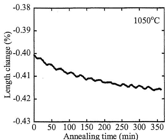
Fig.5.3-19-b \text{B}_4\text{C} 添加 SiC
