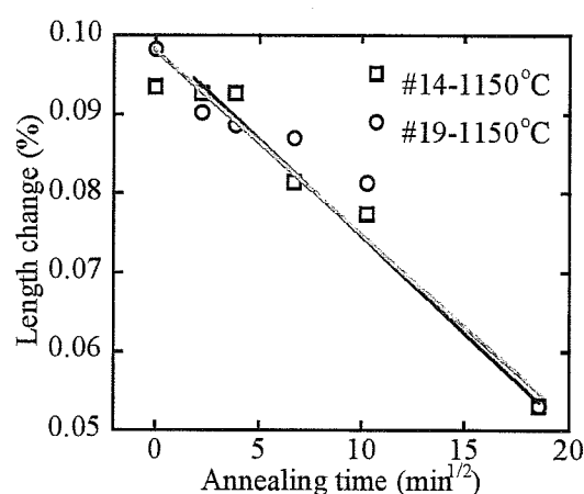
Fig.2.21-b x 軸は保持時間の 1/2 乗
