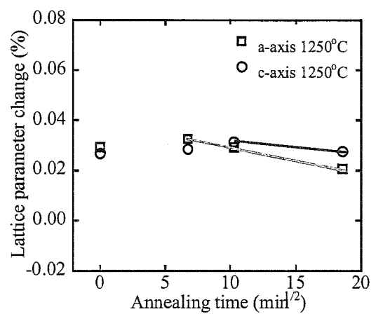
Fig.4.23-b x 軸は保持時間の 1/2 乗
