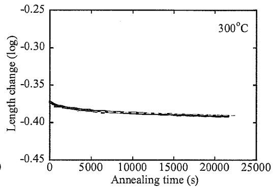
Fig.5.6-4 300°C アニール
