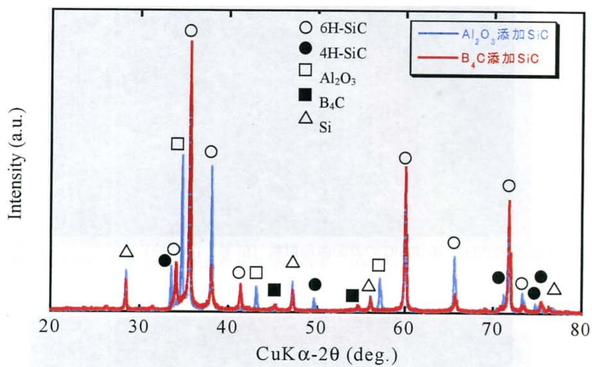
Fig.2.1-1 各試料の XRD プロファイル
