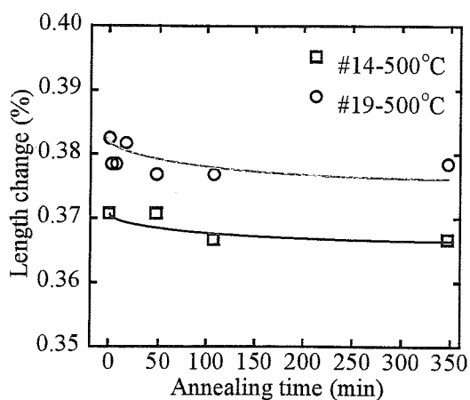
Fig.2.8-a x 軸は保持時間
