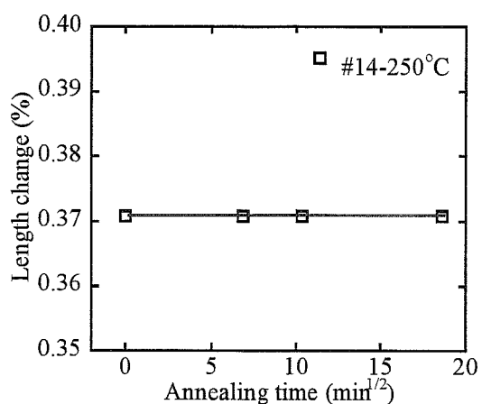
Fig.2.3-b x 軸は保持時間の 1/2 乗
