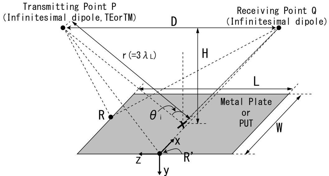
図 5.5: PO による検討モデル
