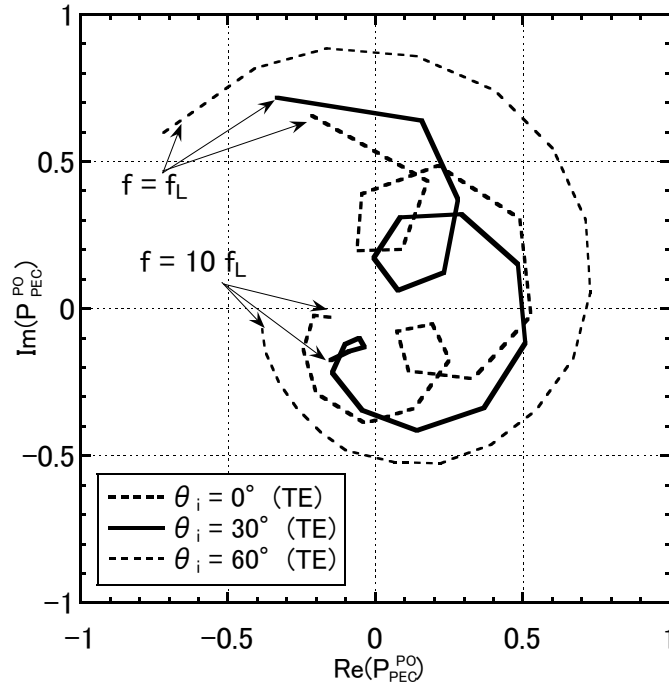
図 5.8: PO 計算結果におけるエッジ散乱波の比率 P_{\text{PEC}}^{\text{PO}} ( L/W = 2 )
