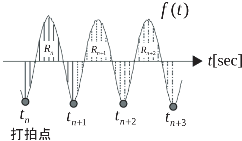
図 6.6: 振幅 RMS 値の測定法
