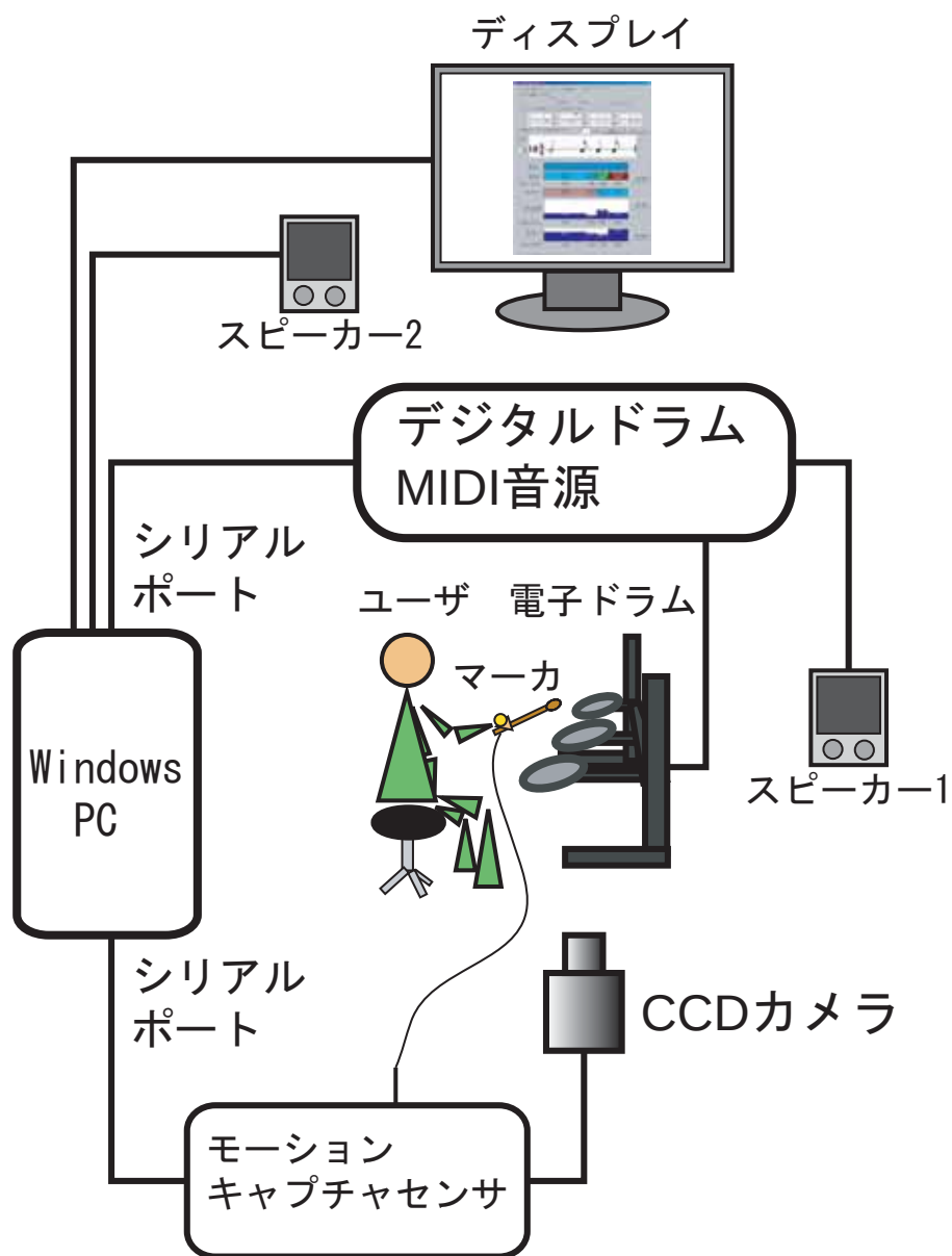
図 9.1: 打楽器学習支援システムの装置構成図
