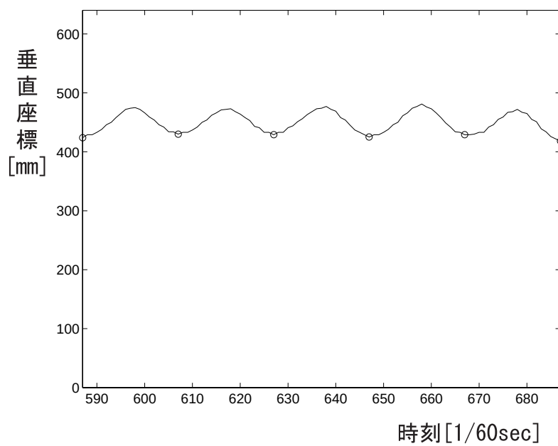
図 6.12: 180bpm における打楽器経験者のストローク波形の例
