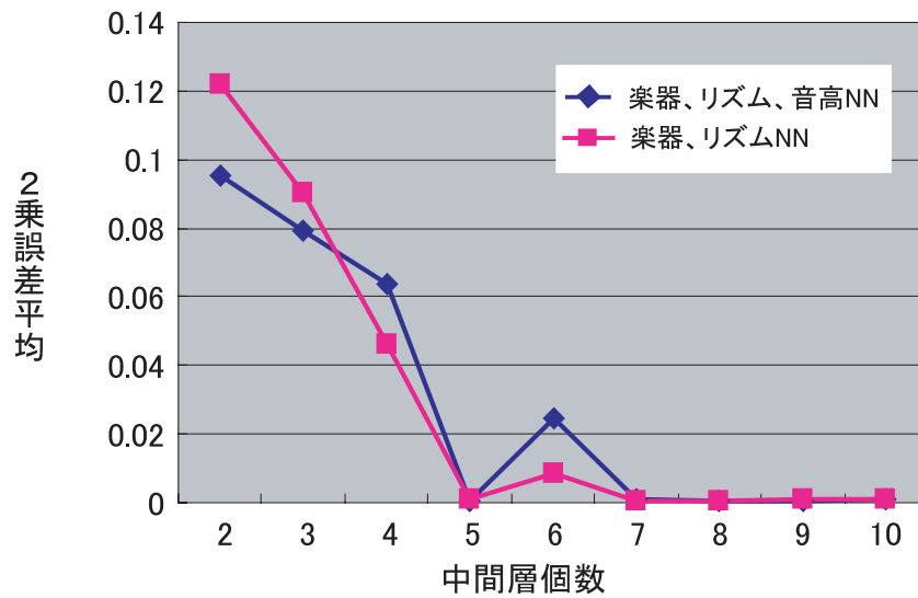
図 3.1: 中間層各ノード数による学習の収束
