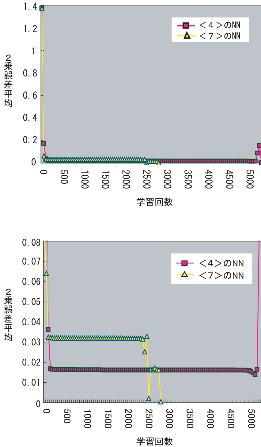
図 3.2: ニューラルネットワークの2乗誤差平均の変化 (上図と下図は、縦軸の縮尺が異なる同一のグラフである)
