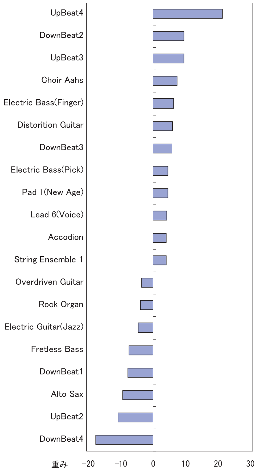
図 4.10: 入力層からノード 5 へのリンクの重みの大きさが大きなもの
