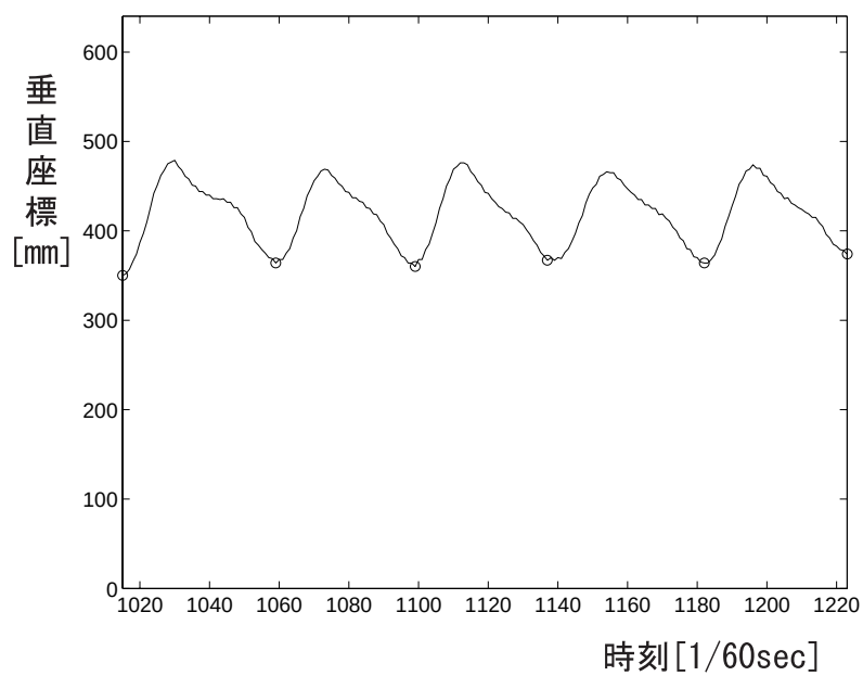
図 6.8: 90bpm における打楽器経験者のストローク波形の例
