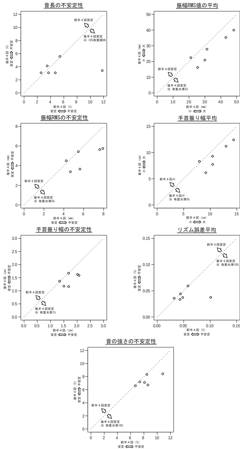
図 9.8: 各特徴量の前半4回と後半4回の平均値の比較
