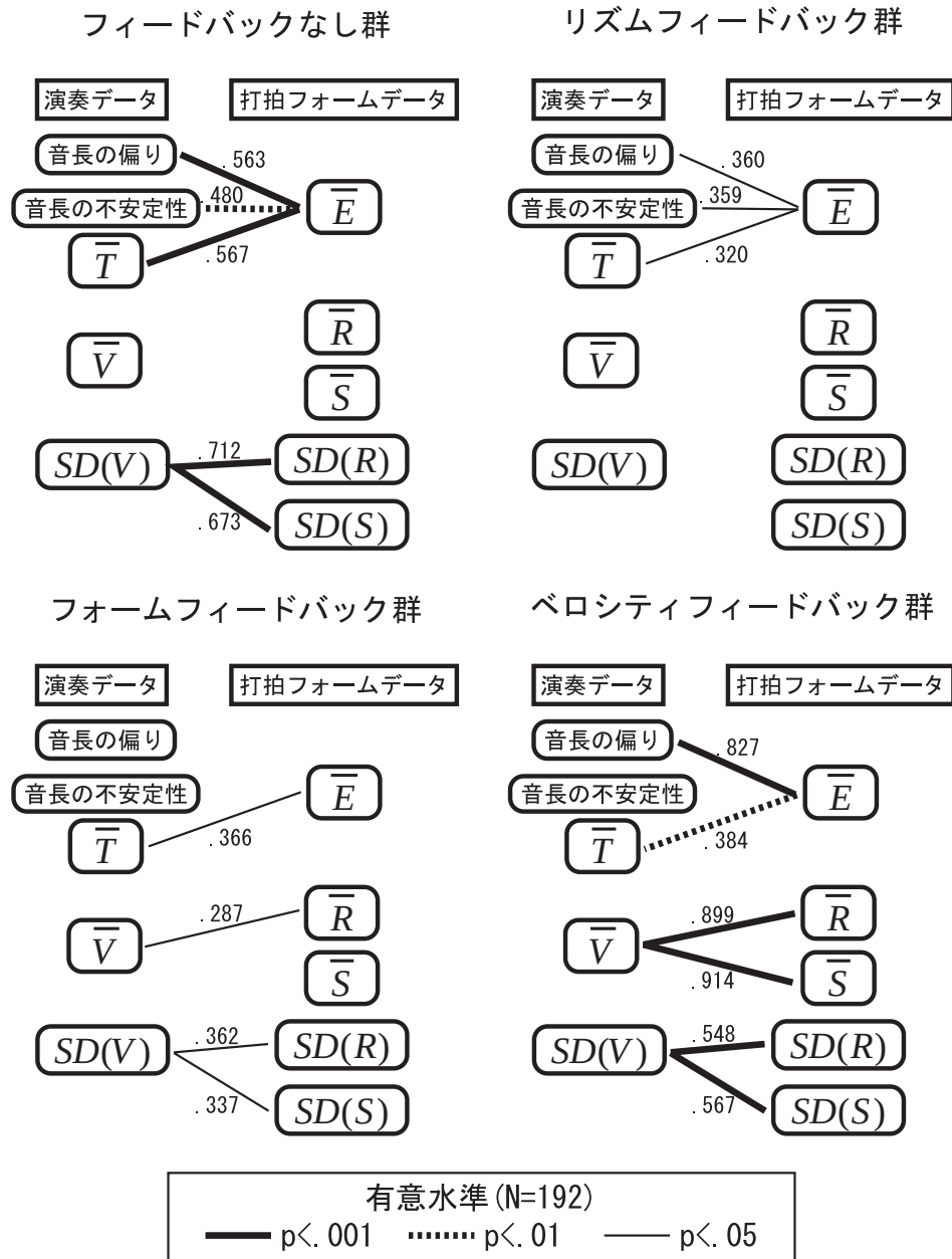
図 9.10: 打楽器未経験者の特徴量間の相関
