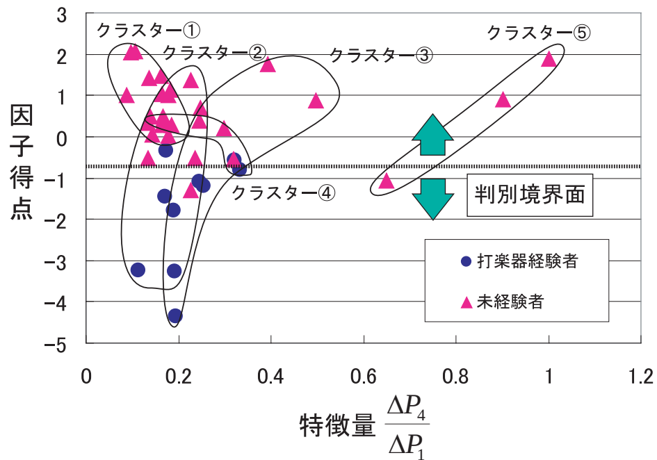
図 6.15: 90bpm の演奏における散布図-(2)
