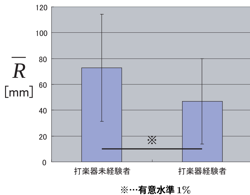
図 7.5: 打楽器経験者、未経験者における振幅 RMS 値平均の t 検定
