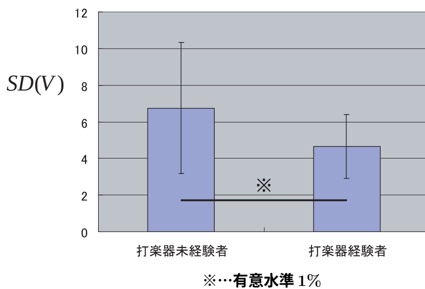
図 7.8: 打楽器経験者、未経験者におけるベロシティ標準偏差の t 検定
