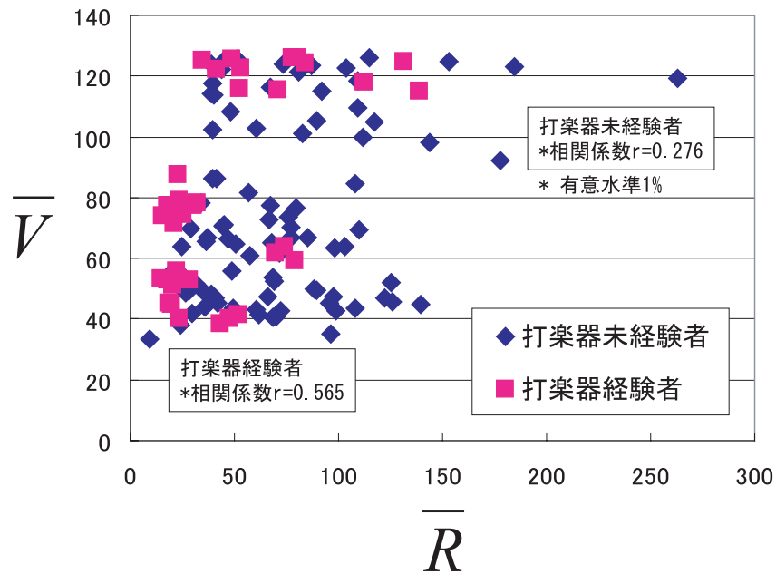
図 7.12: \overline{R}, \overline{V} の散布図
