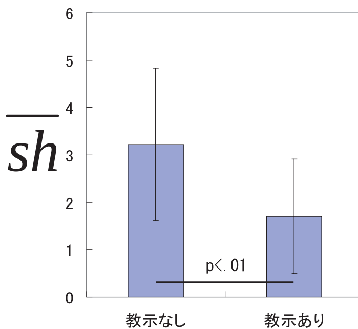
図 5.2: 教示あり、なし群間における音長の偏りの t 検定
