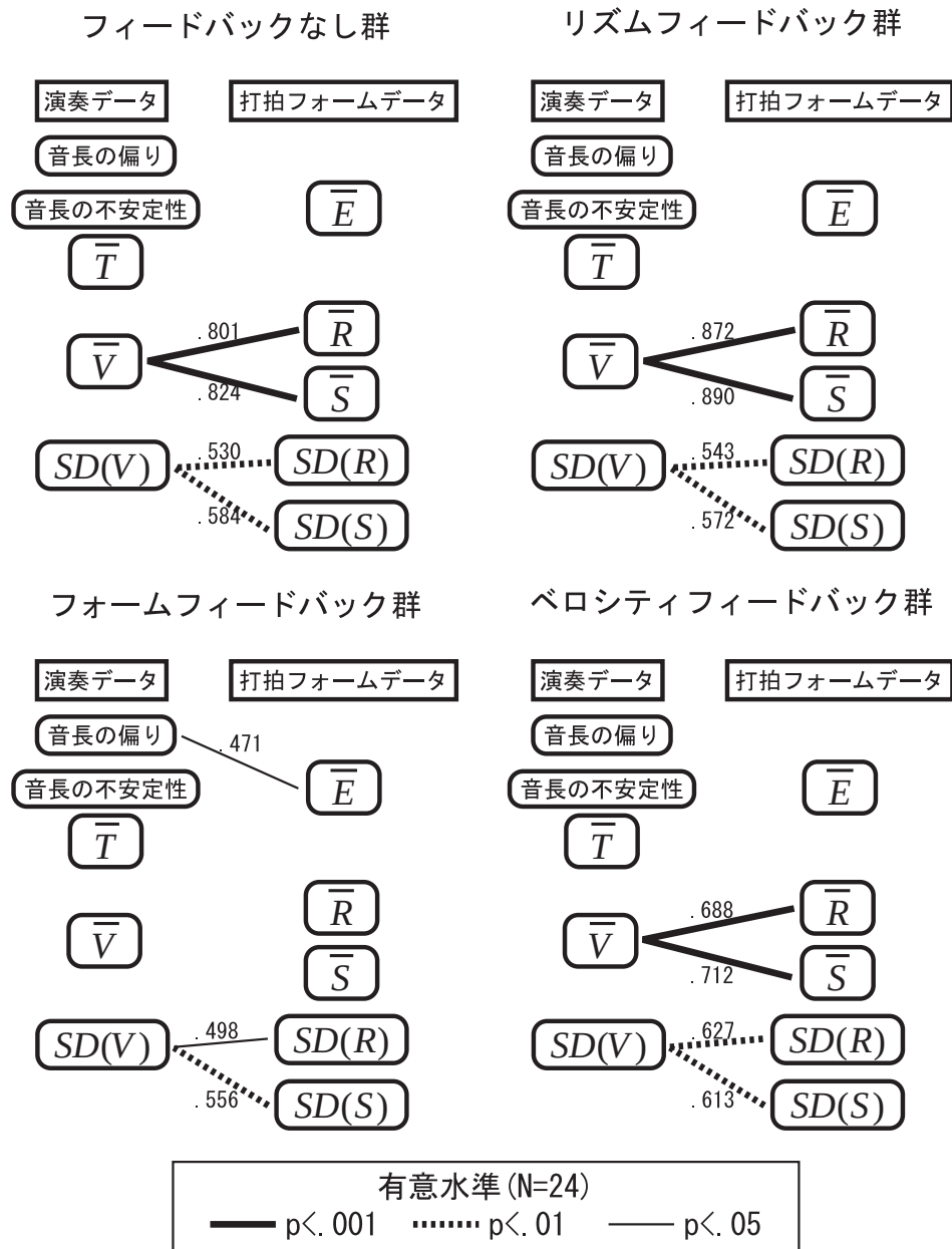
図 9.9: 打楽器経験者の特徴量間の相関
