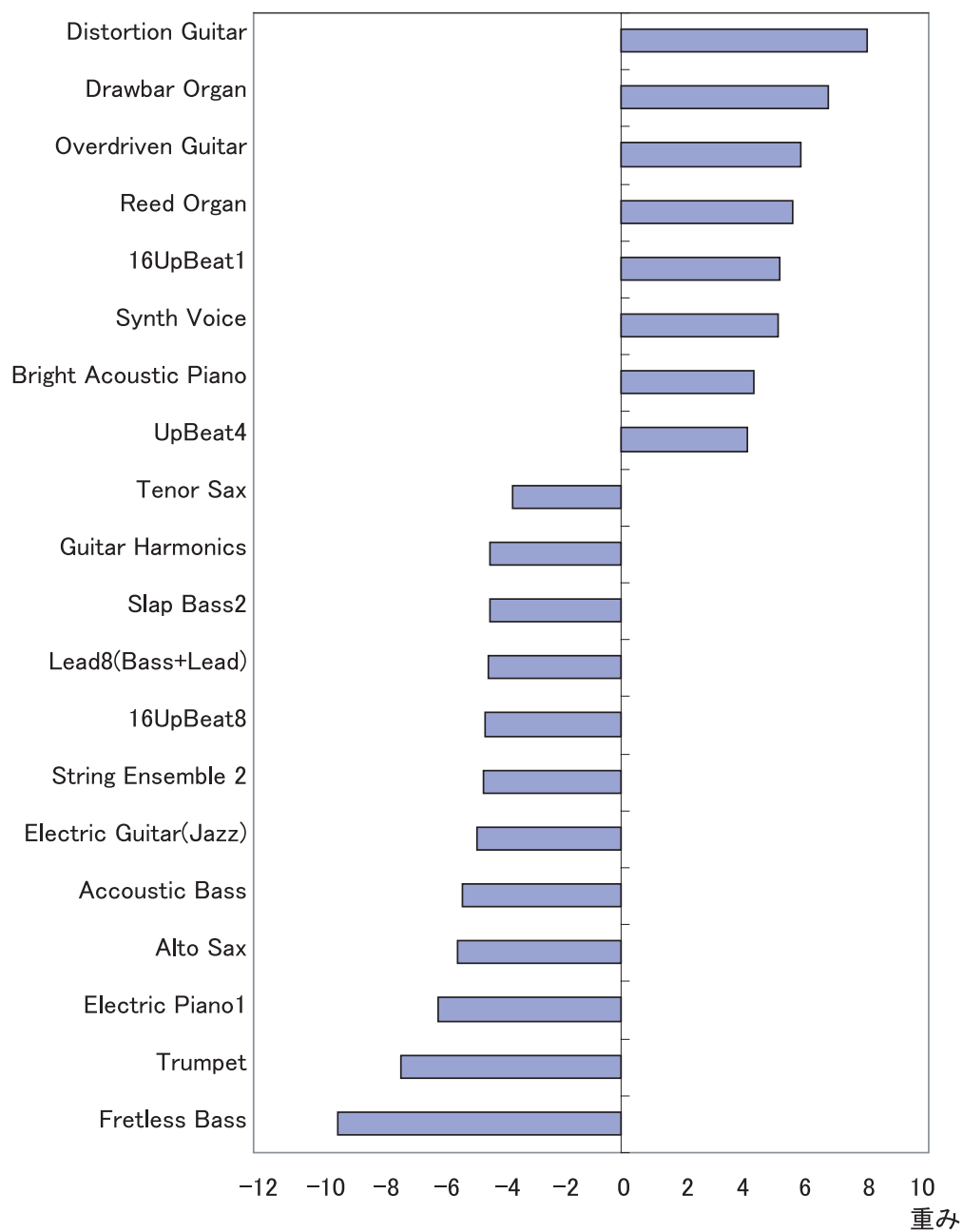
図 4.6: 入力層からノード 1 へのリンクの重みの大きさが大きなもの
