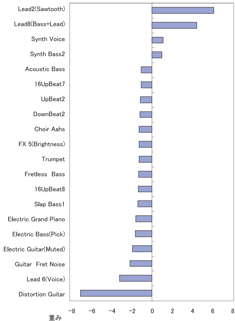
図 4.7: 入力層からノード 2 へのリンクの重みの大きさが大きなもの
