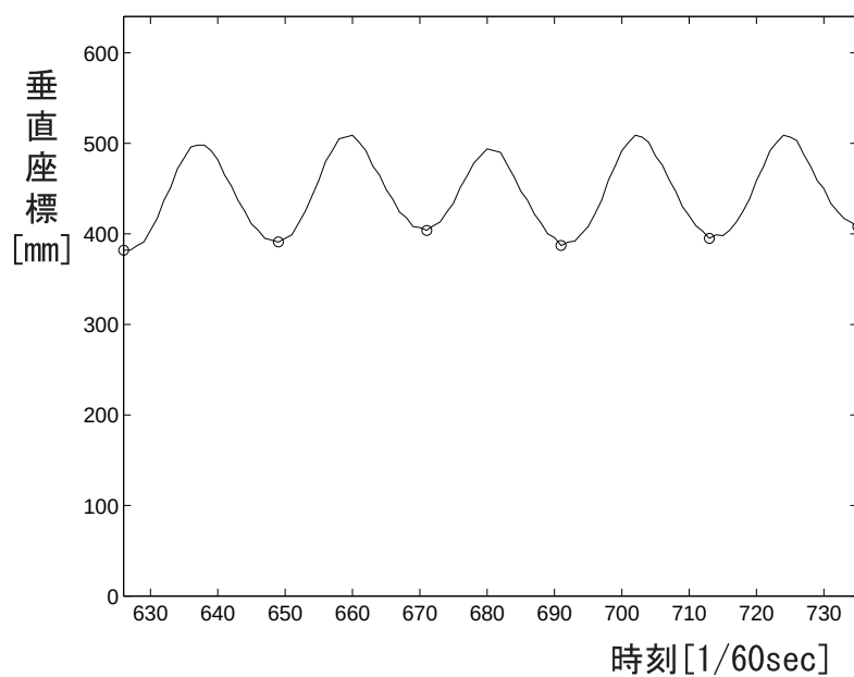
図 6.11: 180bpm における打楽器未経験者のストローク波形の例
