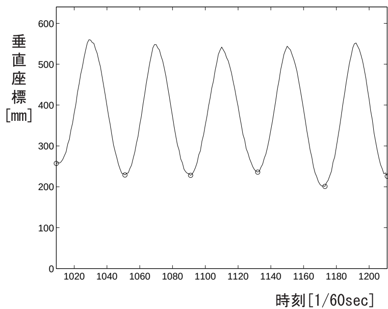
図 6.7: 90bpm における打楽器未経験者のストローク波形の例
