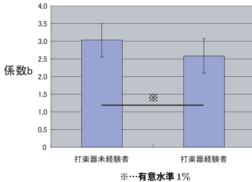
図 7.10: 打楽器経験者、未経験者における一次近似式の係数 b
