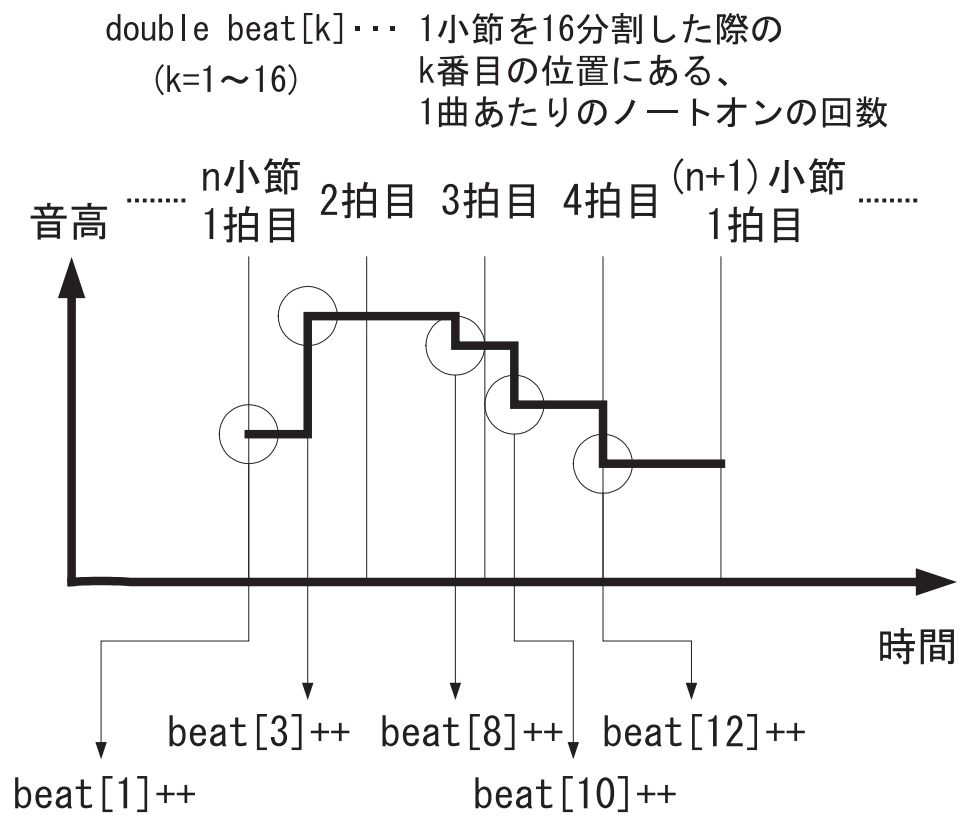
図 2.3: リズムの分布
