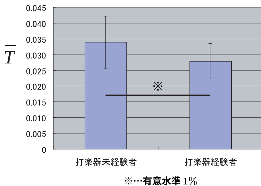
図 7.7: 打楽器経験者、未経験者におけるリズム誤差平均値の t 検定
