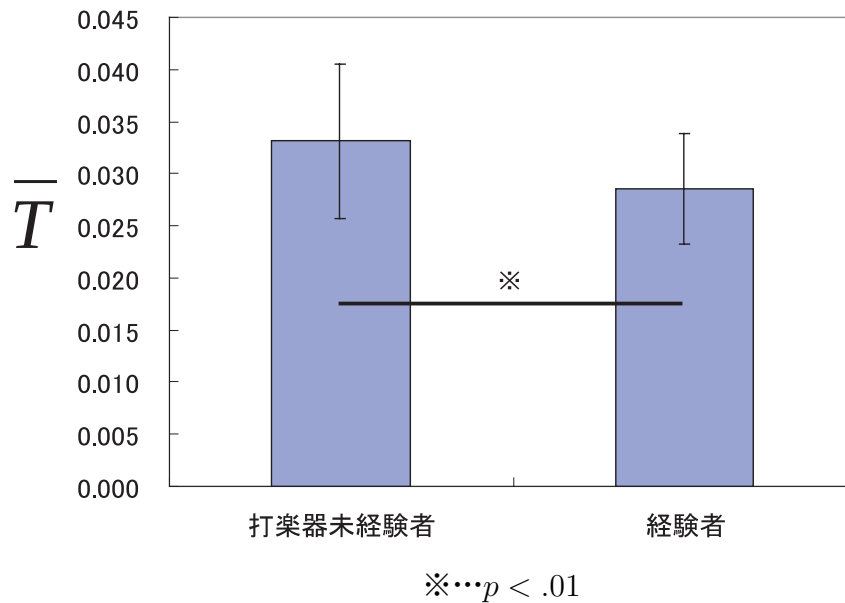
図 8.1: リズム誤差 \bar{T} の比較
