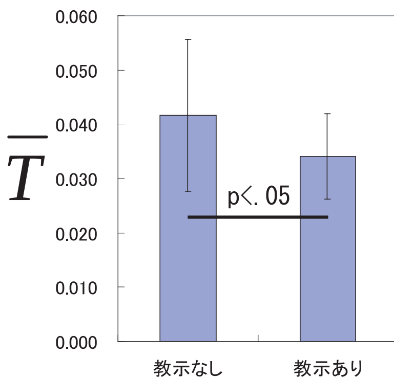
図 5.6: 教示あり、なし群間におけるリズム誤差の t 検定
