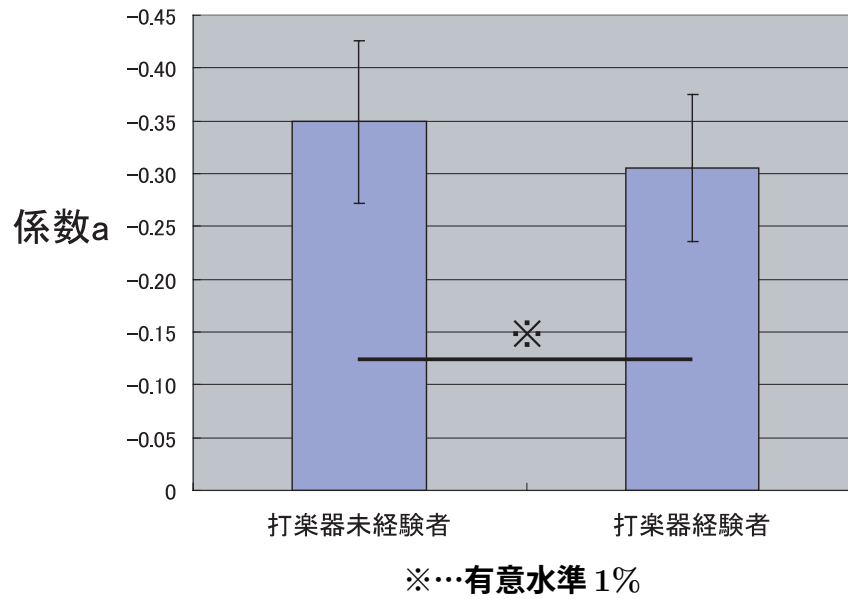
図 7.9: 打楽器経験者、未経験者における一次近似式の係数 a
