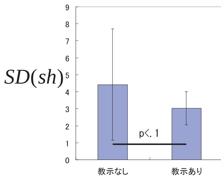
図 5.3: 教示あり、なし群間における音長の偏りの t 検定
