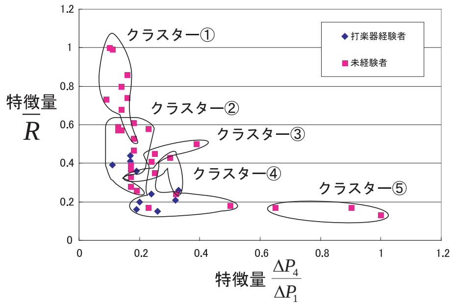
図 6.14: 90bpm の演奏における散布図-(1)
