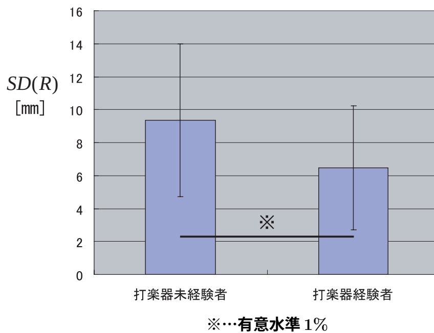
図 7.6: 打楽器経験者、未経験者における振幅 RMS 値標準偏差の t 検定
