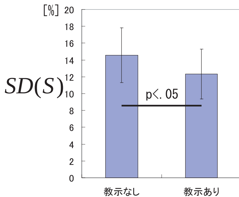
図 5.5: 教示あり、なし群間における振り幅の不安定性の t 検定
