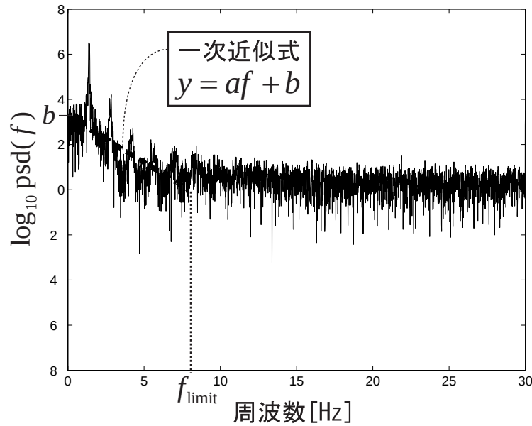
図 7.4: psd 関数の 1 次近似式
