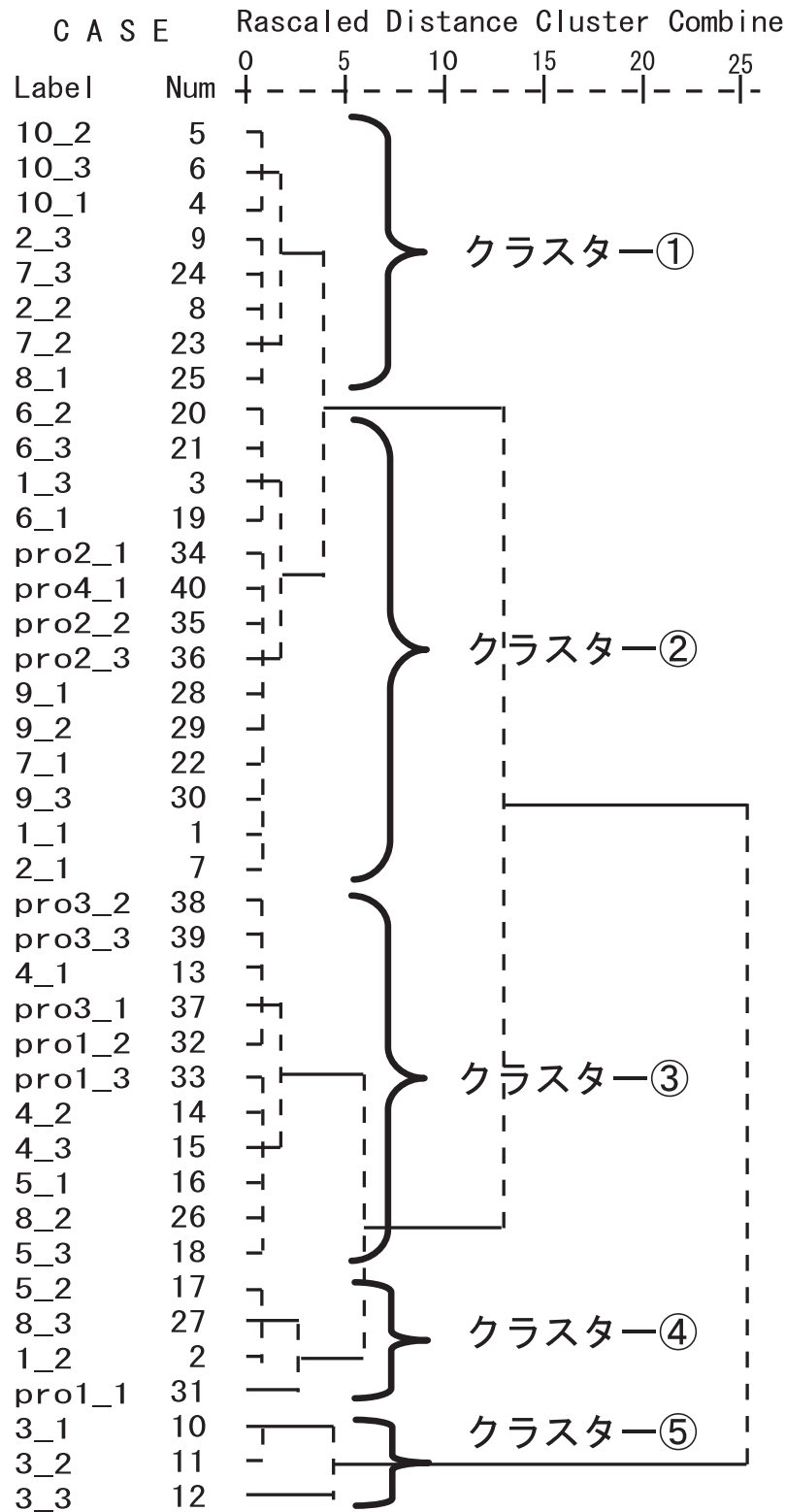
図 6.13: 90bpm の演奏におけるデンドログラム
