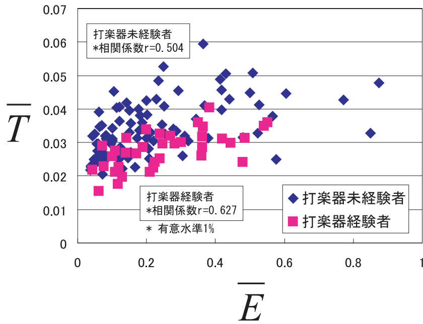
図 7.11: \overline{E}, \overline{T} の散布図
