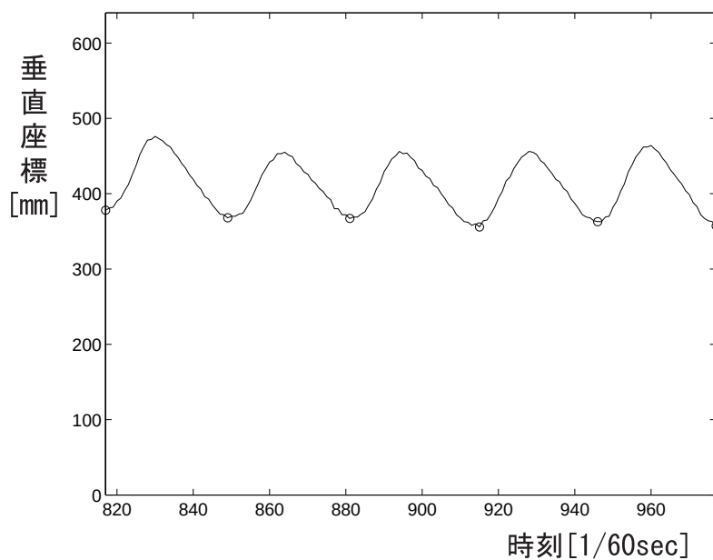
図 6.10: 120bpm における打楽器経験者のストローク波形の例
