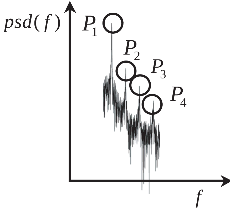
図 6.5: パワースペクトルピーク値の測定法
