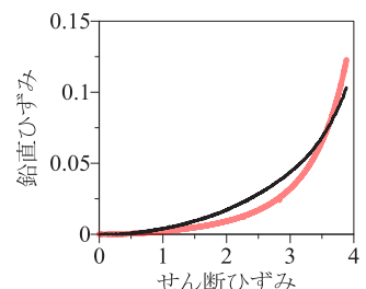
図 6 鉛直ひずみとせん断ひずみの関係
