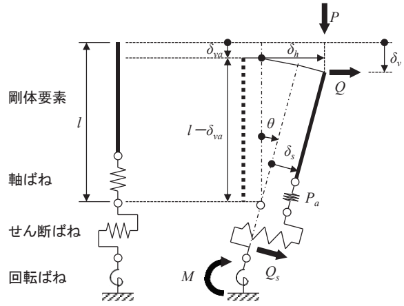
図 1 大変形マクロモデル（修正モデル）
