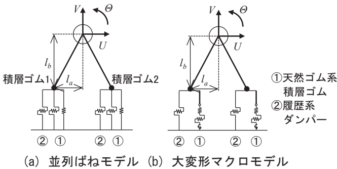
図10 解析モデル
