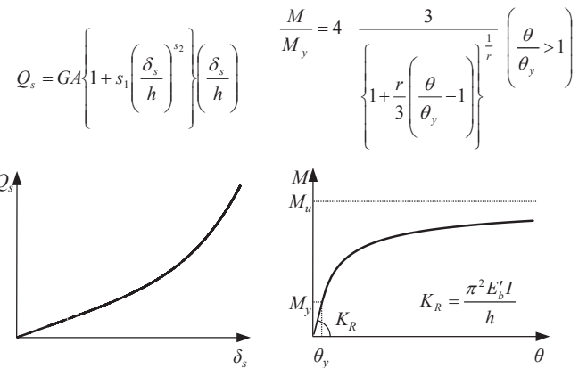
図 2 せん断ばね特性
