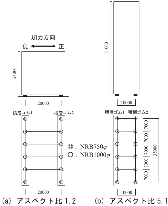
図9 建物モデル
