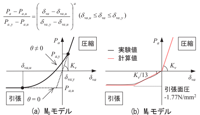
図 4 軸ばね特性
