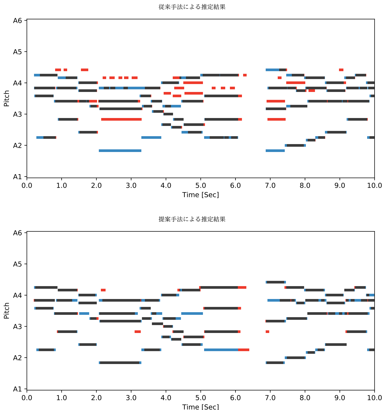
図 2 Bach10 データセット中の楽曲 ‘01-AchGottundHerr’ より、最初の 10 秒間の各手法による音高推定結果ならびに対応する正解音高. 音高 ‘A4’ は 440 Hz の「ラ」に対応している. 図中の黒い領域は音高推定システムが正解した音高, 青い領域は検出しなかった音高, 赤い領域は誤検出した音高を表している.
