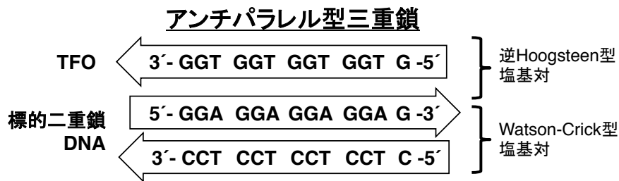
Figure 2-1 アンチパラレル型三重鎖における、各鎖の配向。
