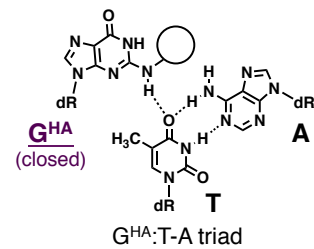
Figure 1-19 三重鎖融解温度( T_m )測定に用いたオリゴデオキシヌクレオチドの配列。
