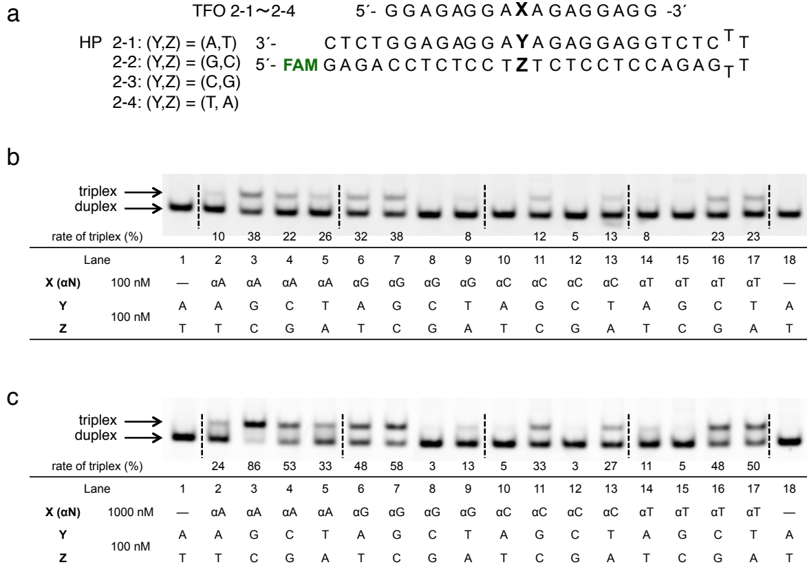
Figure 2-7 ゲルシフトアッセイによる、α-ヌクレオシドを含む TFO の結合能、結合選択性の評価。a)用いた TFO および標的の二重鎖 DNA の配列。b) TFO の濃度が 100 nM の場合の結果。c) TFO の濃度が 1000 nM の場合の結果。 b)および c)のいずれも、Lane1 および 18 は TFO を加えていないコントロール。実験回数はそれぞれ 1 回。実験条件は下記の通り。Incubation: 20 mM Tris-HCl (pH 7.5), 20 mM MgCl 2 , 2.5 mM spermidine, 10% sucrose, 4 °C, 90 min. Electrophoresis: 10% Native gel containing 20 mM Tris-borate, 20 mM MgCl 2 , 180V, 4 °C, 2 h.
