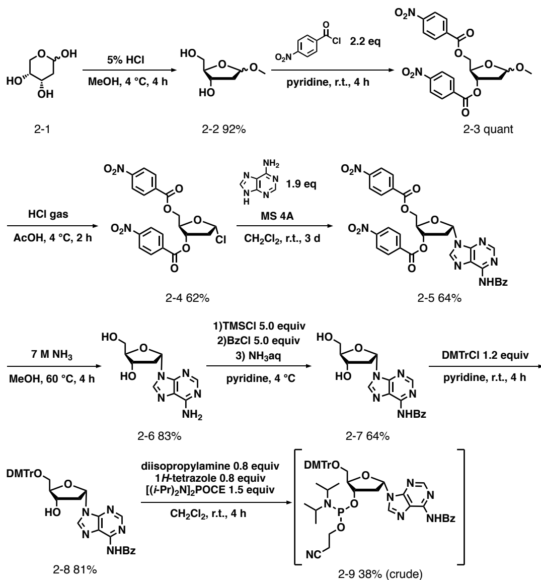
Scheme 2-1 \alpha A ホスホロアミダイトユニットの合成
