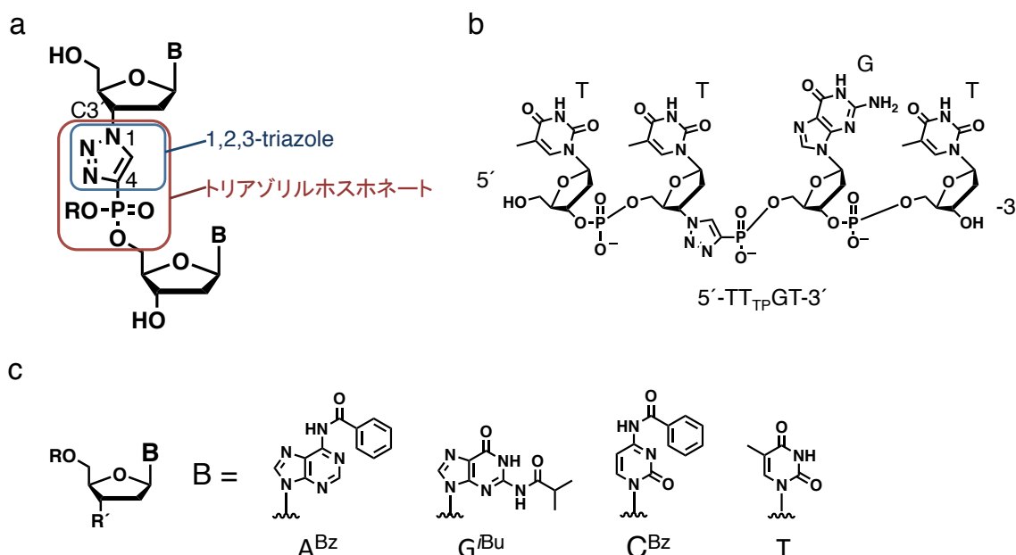
Figure 3-3 本章で用いる、構造についての表記および省略表記。a) トリアゾリルホスホネート構造が示す構造。b) 下付きで T_p と表記される二量体もしくはオリゴヌクレオチド内のトリアゾリルホスホネート構造 c) 塩基部の省略表記
