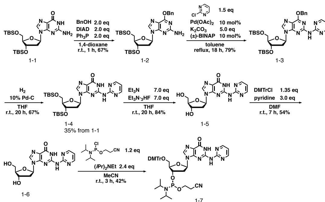
Scheme 1-1. 伊藤らによって行われた G Pym 誘導體の合成
