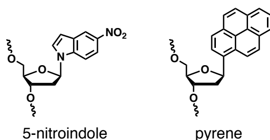
Figure 1-17 5-nitroindoleおよびpyreneを有する人工核酸
