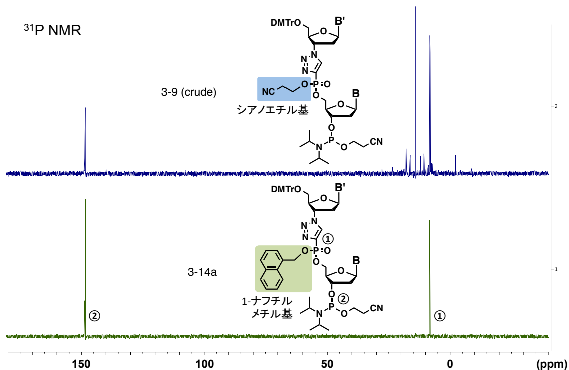
Figure 3-6 シアンエチル基を用いた二量体ホスホロアミダイトユニット 3-9 (crude)と本節で合成した 3-14a の ^{31}\text{P} -NMR の比較。図中の番号は、ピークとその由来となるリン原子の対応を表す。
