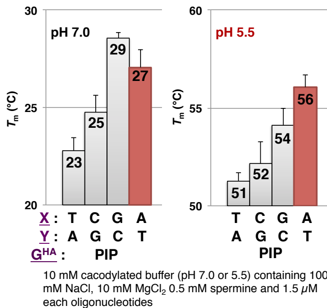
Figure 1-22. (右)G HA sを含む三重鎖のpH 5.5での T_m 値( ^\circ\text{C} )。比較のため、pH 7.0のときの T_m 値( ^\circ\text{C} )も示した(左)。
