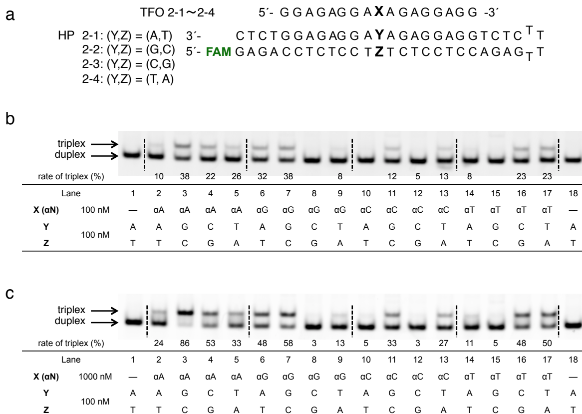
Figure 2-7 ゲルシフトアッセイによる、α-ヌクレオシドを含む TFO の結合能、結合選択性の評価。a)用いた TFO および標的三重鎖 DNA の配列。b) TFO の濃度が 100 nM の場合の結果。c) TFO の濃度が 1000 nM の場合の結果。 b)および c)のいずれも、Lane1 および 18 は TFO を加えていないコントロール。実験回数はそれぞれ 1 回。実験条件は下記の通り。Incubation: 20 mM Tris-HCl (pH 7.5), 20 mM MgCl 2 , 2.5 mM spermidine, 10% sucrose, 4 °C, 90 min. Electrophoresis: 10% Native gel containing 20 mM Tris-borate, 20 mM MgCl 2 , 180V, 4 °C, 2 h.
