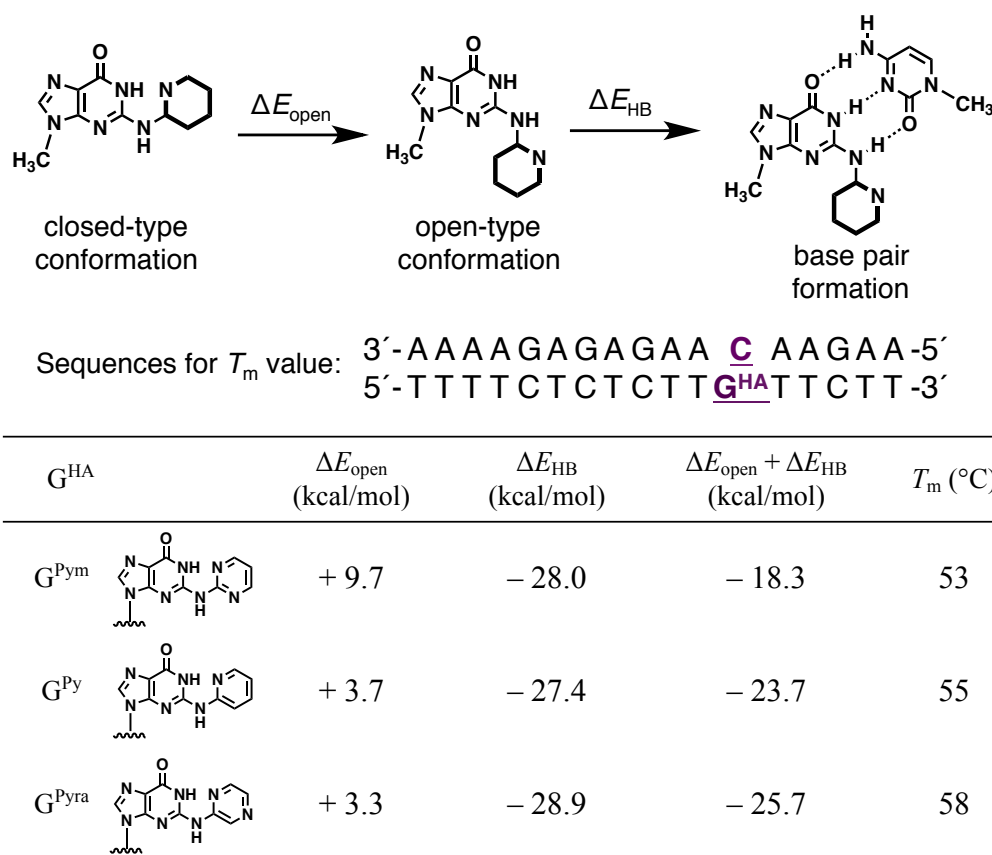
Figure 1-16 G^{\text{Py}} 、 G^{\text{Pym}} 、 G^{\text{Pyra}} の \Delta E_{\text{open}} および \Delta E_{\text{HB}} と G^{\text{HA}}\text{s}-\text{C} 塩基対を含む二重鎖の T_m 値の比較。
