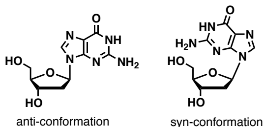
Figure 1-26 a)本節で用いた配列が形成する(3 + 1) hybrid 型グアニン四重鎖の構造。b)ヌクレオシドのコンホメーション。
