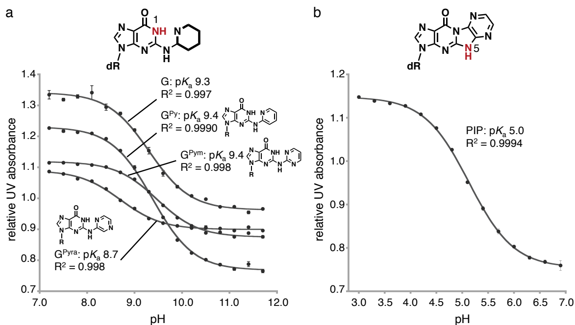
Figure 1-11. G^{HA} の pK_a の測定。条件: デオキシグアノシン ( G )、 1-9a ( G^{Py} )、 1-6 ( G^{Pym} )、 1-9b ( G^{Pyra} ): 25 \mu M、200 mM グリシン-NaOH buffer、1% DMSO。 1-9c (PIP): 25 \mu M、200 mM クエン酸-NaOH buffer、1% DMSO。吸光度比の算出に用いた波長は下記の通り。 G : 254 nm/265 nm、 G^{Py} : 264 nm/275 nm、 G^{Pym} : 266 nm/275 nm、 G^{Pyra} : 266 nm/274 nm、PIP: 268 nm/278 nm。全ての UV 吸収測定は 3 回行い、平均値と標準偏差を示した。
