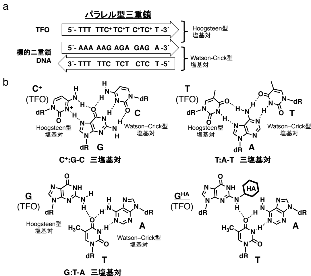
Figure 1-4. G^{HA} を含む TFO による三重鎖形成の可能性。 a) 平行型三重鎖 DNA の鎖の配向。 b) C^+:G-C 、 T:A-T 、 G:T-A 三塩基対の構造と、 G^{HA} が T に結合する予想図。
