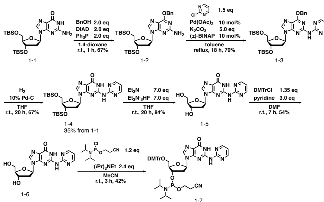
Scheme 1-1. 伊藤らによって行われた G^{\text{Pym}} 誘導体の合成
