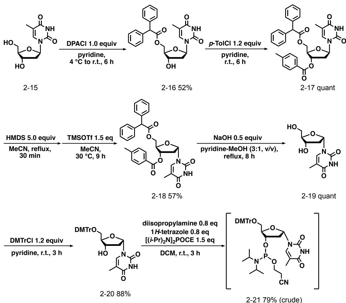
Scheme 2-3 \alpha T ホスホロアミダイトユニットの合成
