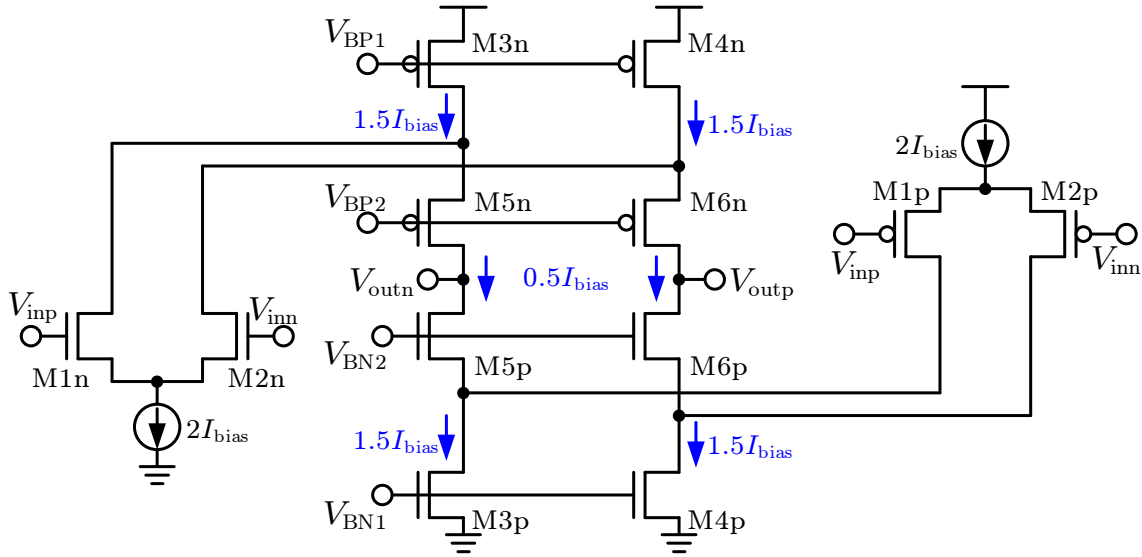
図 3.15: 相補入力型フォールデッドカスコードオペアンプ [10]
