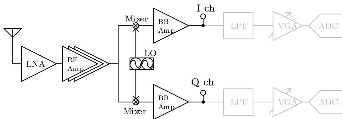
図 2.20: 表 2.1 の回路構成
