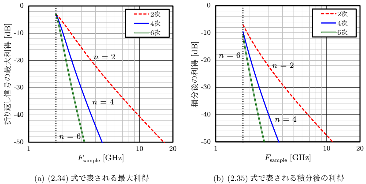
図 2.18: サンプリング周波数と折り返し成分の減衰
