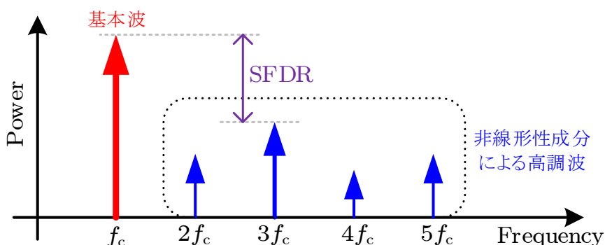
図 1.6: SFDR の評価時のスペクトラム
