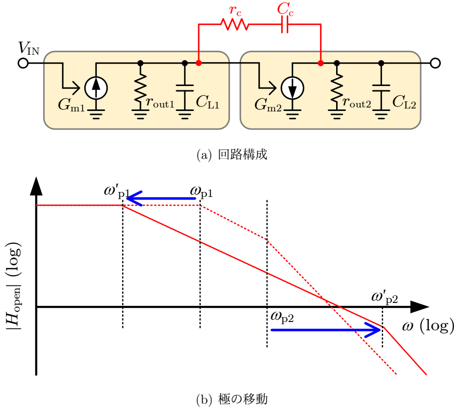
図 3.8: ポールスプリッティング
