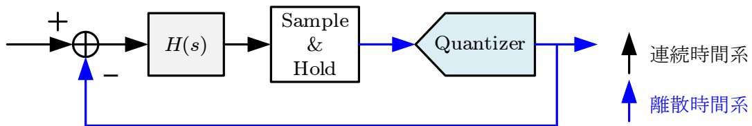
(a) 連続時間型構成
