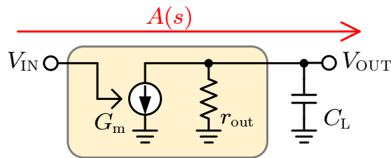
図 3.9: 一段オペアンプのモデル
