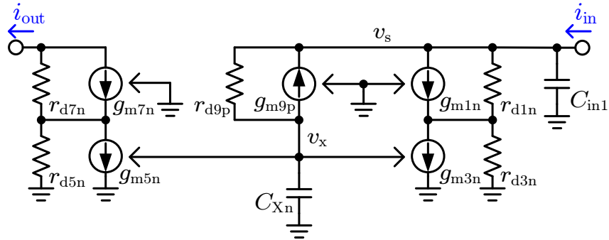
図 7.29: SSF 構造を持つ電流増幅器の小信号等価回路
