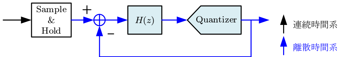
(b) 離散時間型構成
