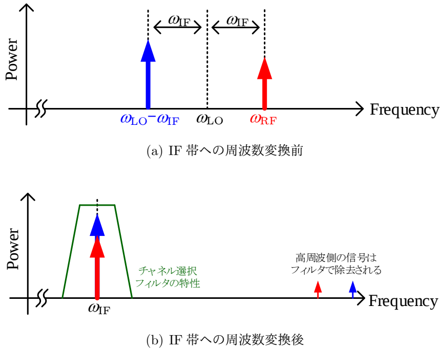
図 2.2: IF 帯への変換とイメージ妨害波
