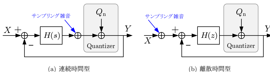
図 6.6: サンプルング雑音の比較
