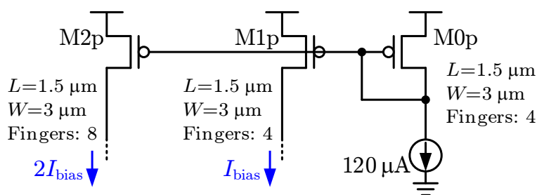
図 5.21: 参照電流源
