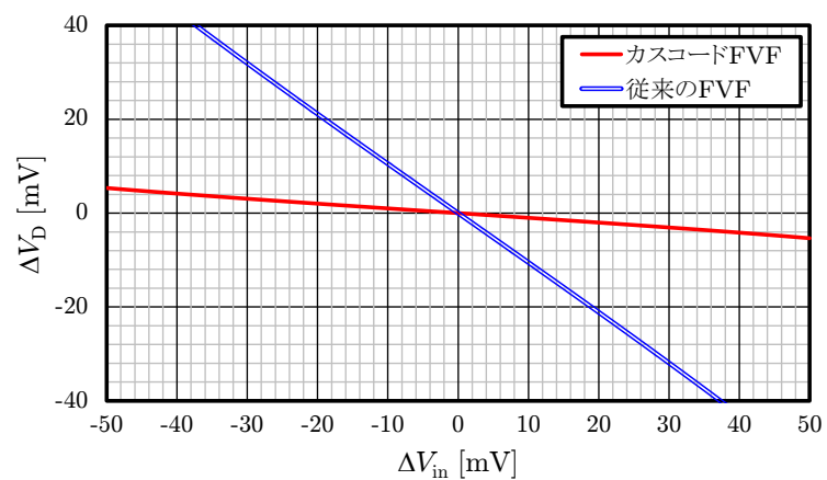
(b) \Delta V_D の DC 特性
