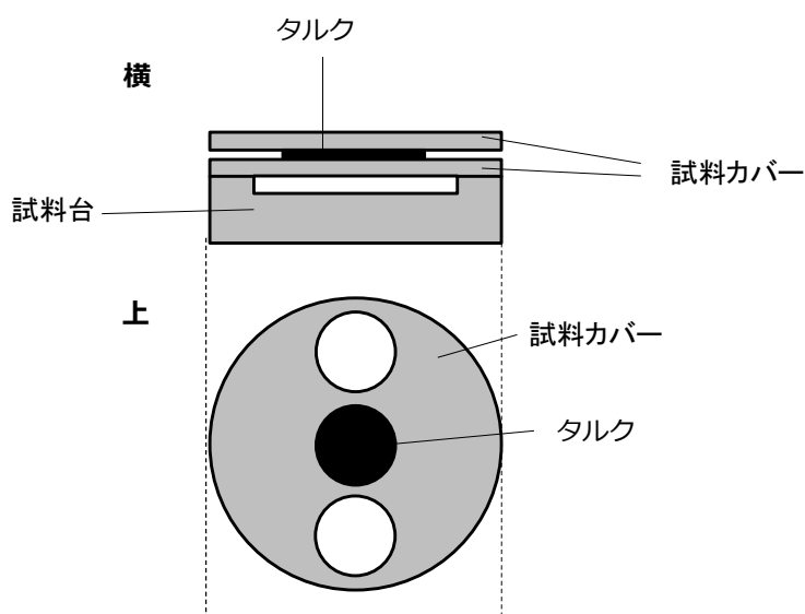
Fig. 2.1 試料台にタルクを取り付けた模式図
