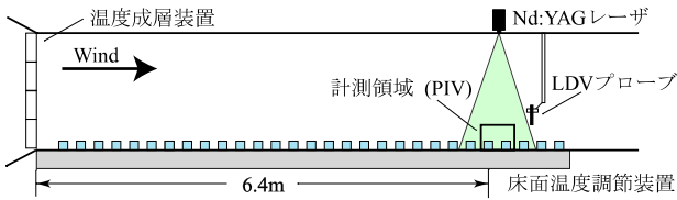
図-3 風洞実験の概要
