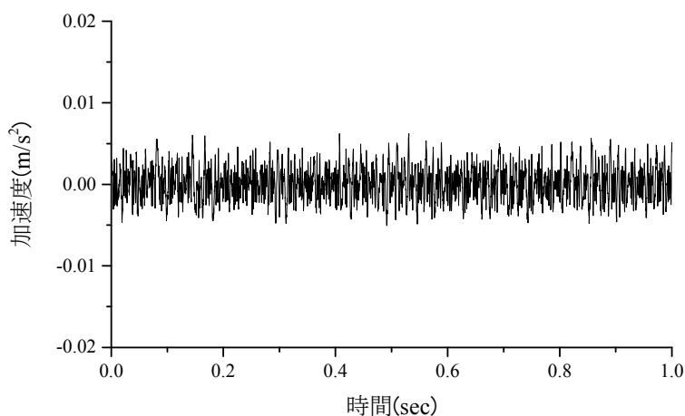
図 2-38 圧電型加速度計のノイズ計測結果
