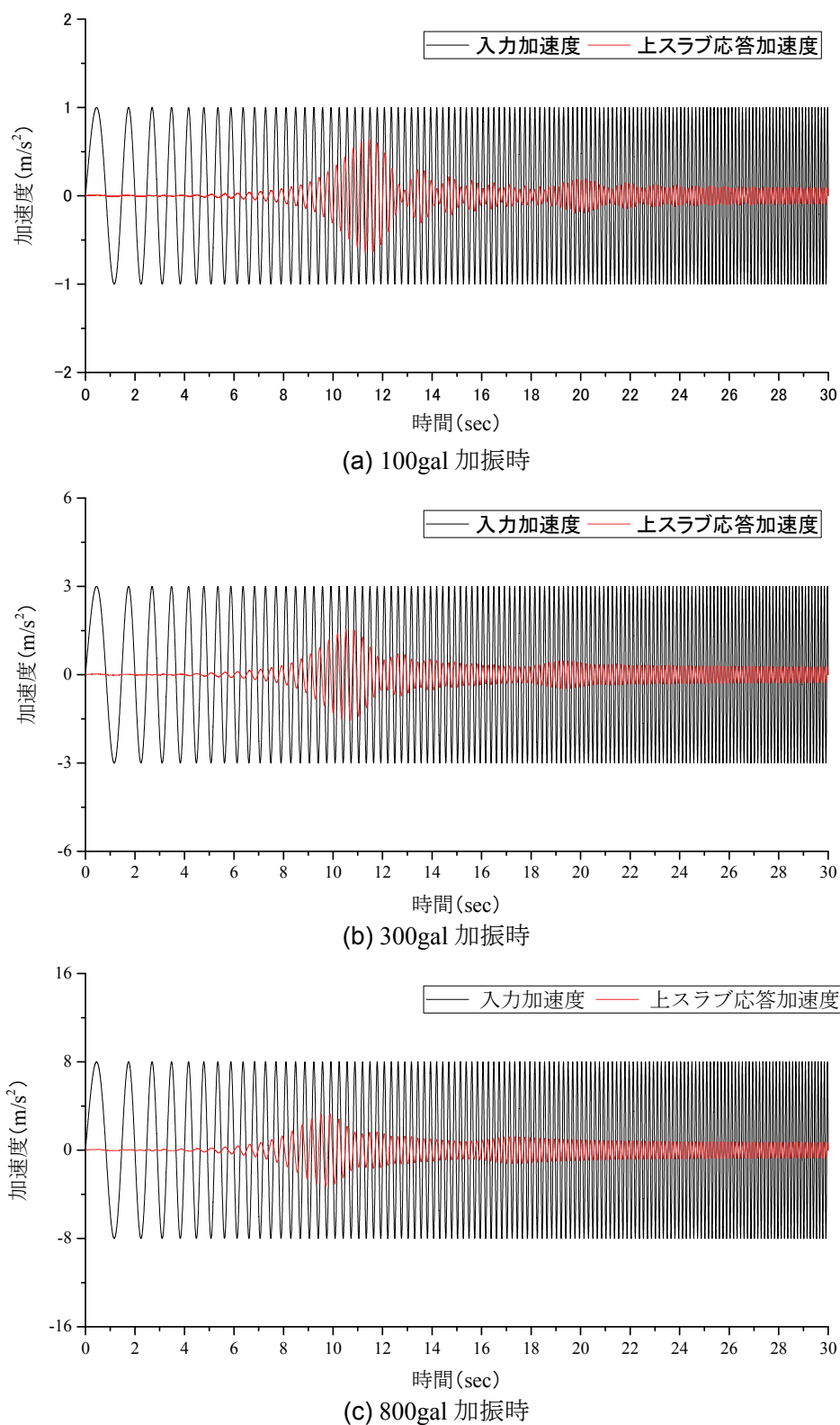
図 4-20 共振実験の再現解析結果 (時刻歴波形)
