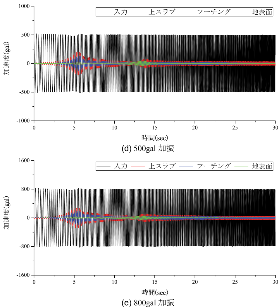
図 4-4 上部工ありの構造における共振実験結果（時刻歴波形）（その2）
