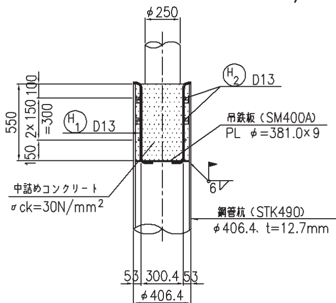
図 6-7 杭頭部の一般図
