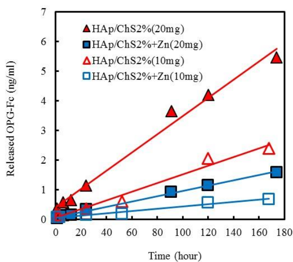
Fig. 3-5 製剤化粒子の重量を変化させたときの OPG-Fc の放出量への影響
