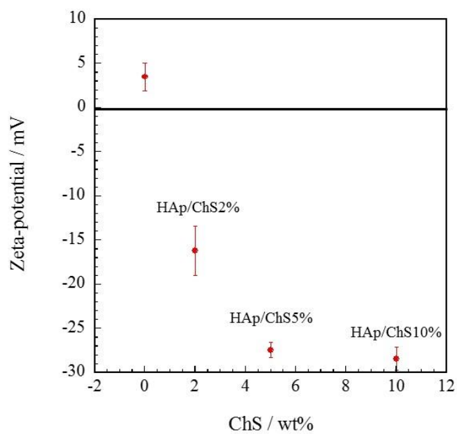
Fig. 2-27 HAp/ChS 多孔質微粒子のゼータ電位 [67]
