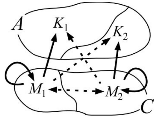
図3 二分可能な合意形成状況 ステークホルダー(意思決定者)が二分され、政策案に対する意見にまったく重なりがない。
