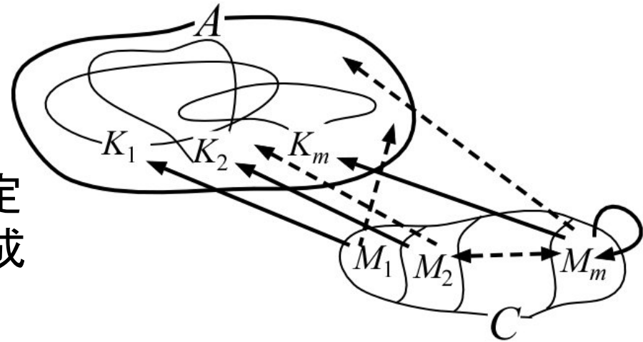
図4 擬集群化可能 な合意形成状況 ステークホルダー(意思決定者)が分割されている。しかし、 政策案に対する意見には重なりが存在し得る。
