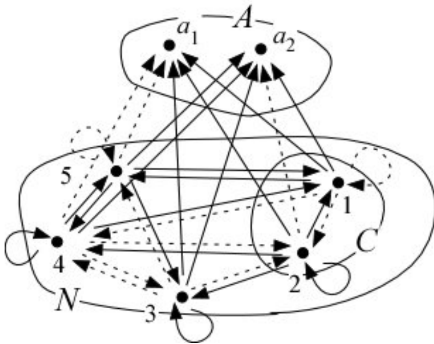
図1 社会的意思決定状況(SDMS)の例.
