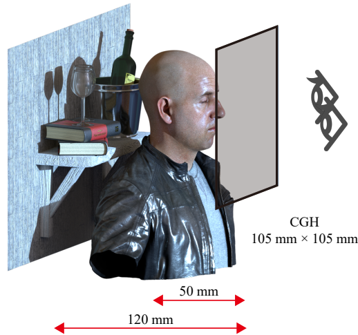
図 6.5 計算する立体像と CGH のセットアップ
