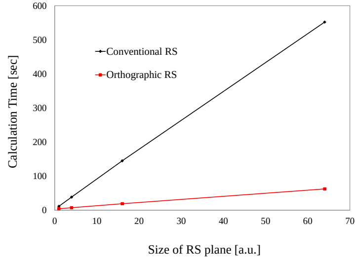
図 3.8 従来手法・提案手法における RS 面サイズと計算時間関係の比較
