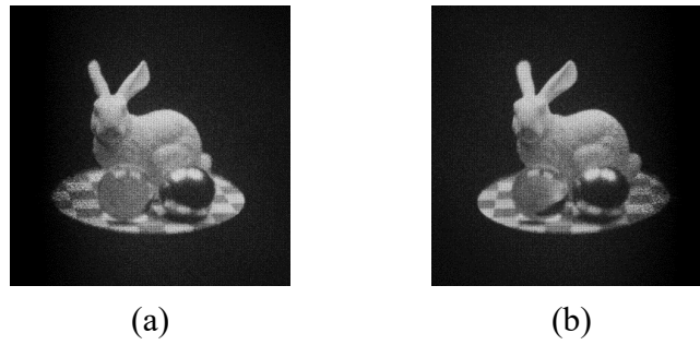
図 4.7 ORS 面を用いた CGH からの (a) 左と (b) 右から観察した立体像再生シミュレーション結果
