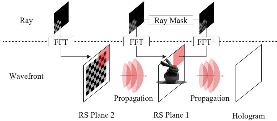
図 5.5 従来の RS 面を用いた相互オクルージョン処理のフロー
