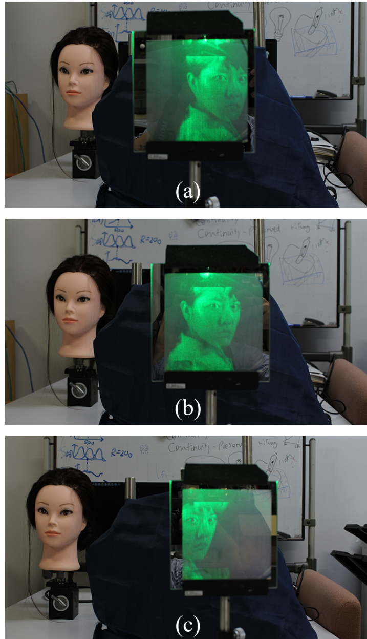
図 4.17 (a) 左 (b) 正面 (c) 右から撮影した実物体を用いた CGH 光学再生像
