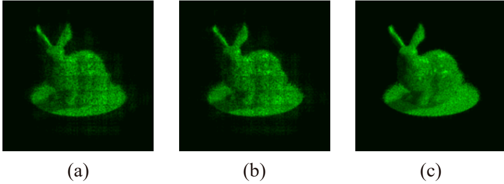
図 7.4 (a) 帯域制限フレネル伝搬, (b) シフト角スペクトル法, (c) 提案手法を用いて生成した CGH の再生シミュレーション結果
