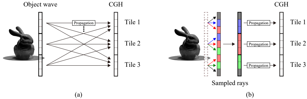
図 4.3 (a) 従来のタイリングを用いた伝搬計算と (b) 提案する光線組み換えによる伝搬計算
