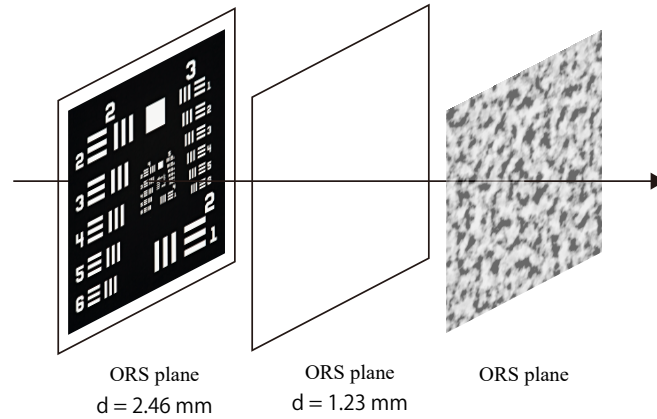
図 3.11 物体面-ORS 面間距離に対する再生像比較における物体と CGH のセットアップ
