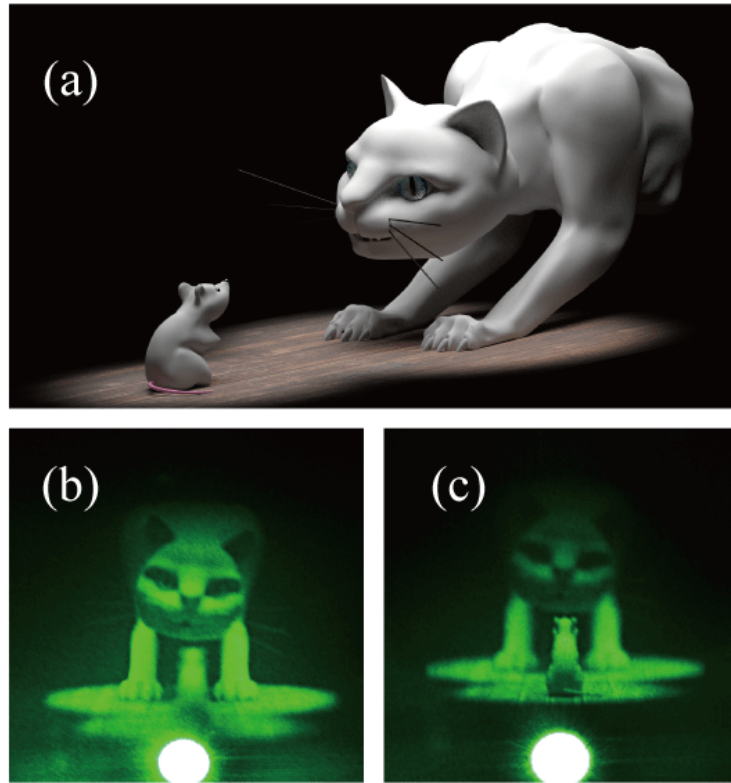
図 5.10 (a) ホログラム生成に用いた 3DCG シーン, (b) ネコにピントを合わせた光学再生像, (c) ネズミにピントを合わせた光学再生像
