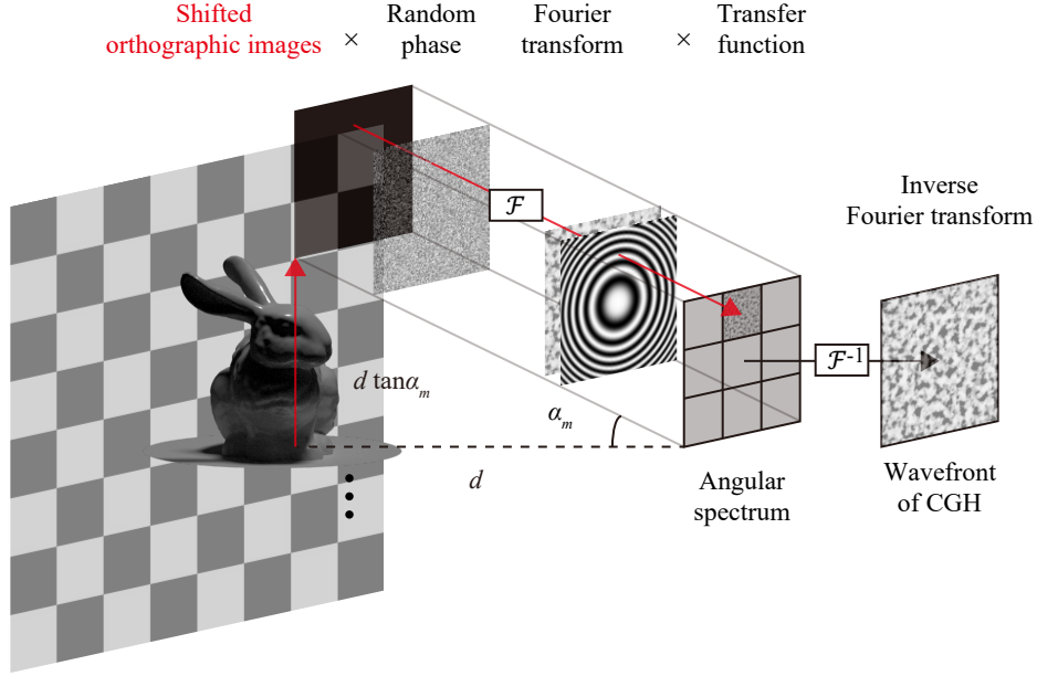
図 4.1 シフト正射影光線を用いた CGH 計算法
