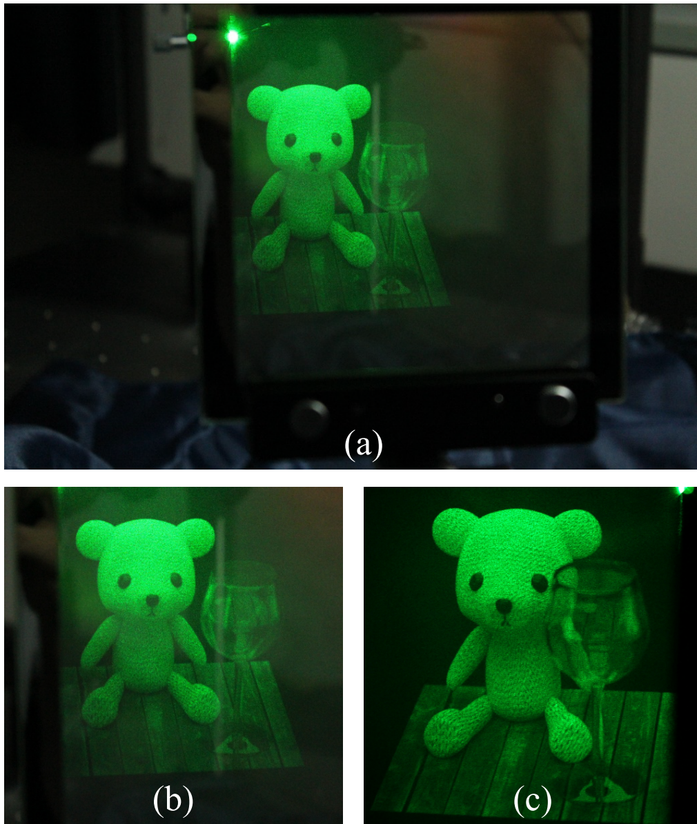
図 4.13 (a) 左 (b) 右 (c) 正面から撮影したクマとワイングラス CGH 光学再生像
