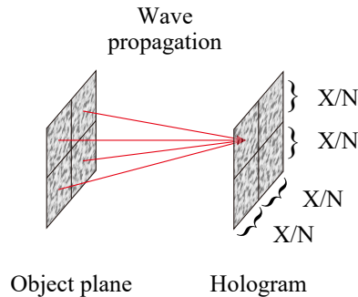
図 4.4 タイリングを用いた CGH 計算の計算量概算
