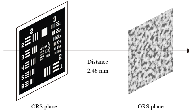
図 3.9 再生像比較における物体と CGH のセットアップ
