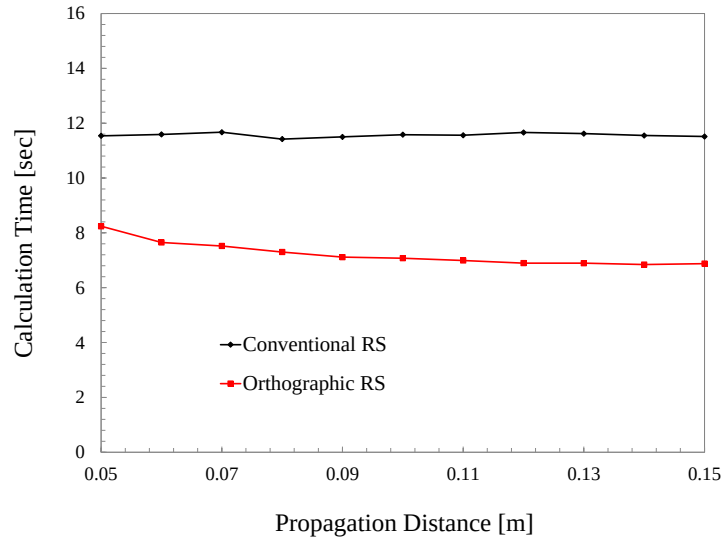
図 3.7 従来手法と提案手法の伝搬距離に対する計算時間の比較
