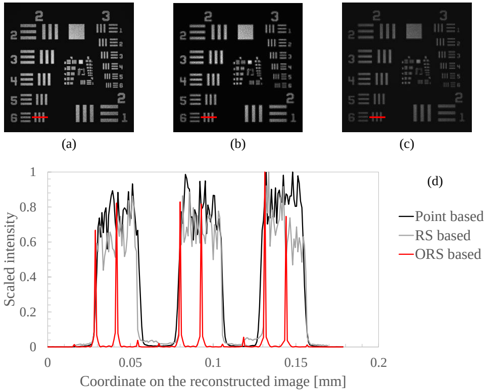
図 3.10 (a) 点光源法, (b) 従来手法, (c) 提案手法における再生像の比較と (d) ラインプロファイル
