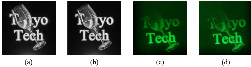
図 3.17 (a) 従来の RS 面, (b) 提案手法再生像のシミュレーション結果, 提案手法によって計算した (c) 左と (d) 右から観察した CGH の光学再生像.
