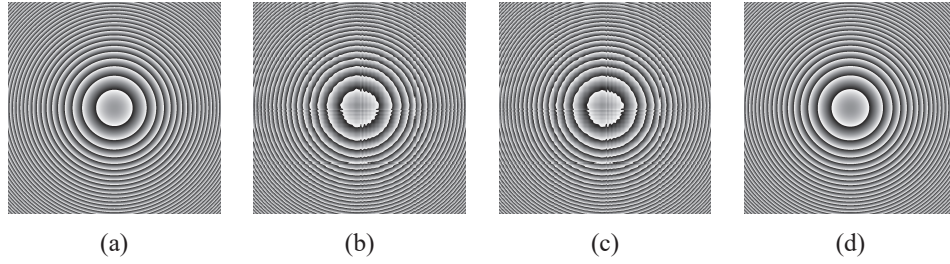
図 7.3 各種伝搬計算法を用いた結果の位相. (a) 解析解, (b) 帯域制限フレネル伝搬, (c) シフト角スペクトル法, (d) 提案手法.
