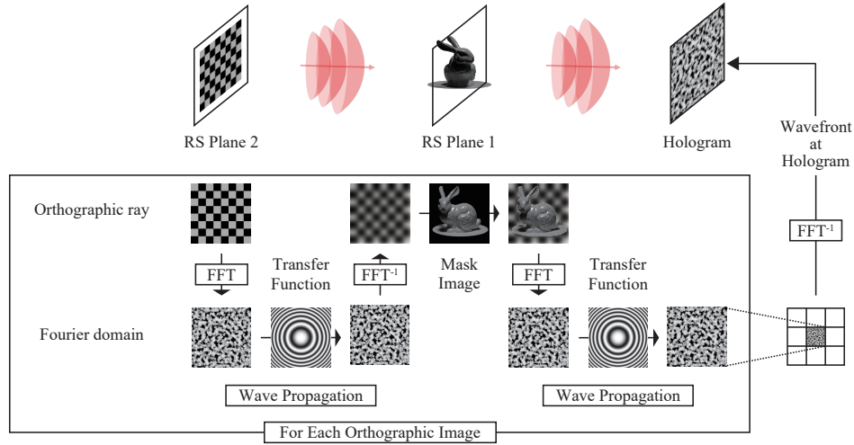
図 5.6 ORS 面を用いた相互オクルージョン処理のフロー
