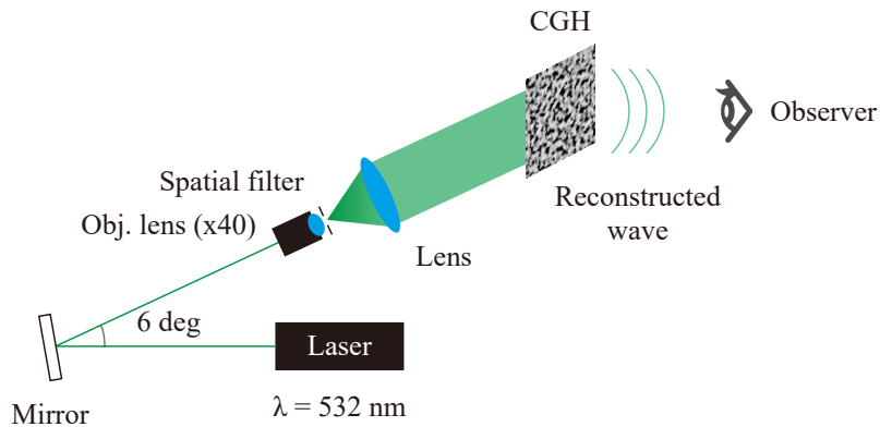
図 3.18 CGH 再生光学系図
