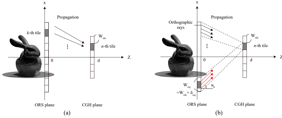
図 4.2 (a) 従来のタイリング計算と比較した (b) 正射影光線-波面変換を用いた大規模 CGH 分割計算のコンセプト
