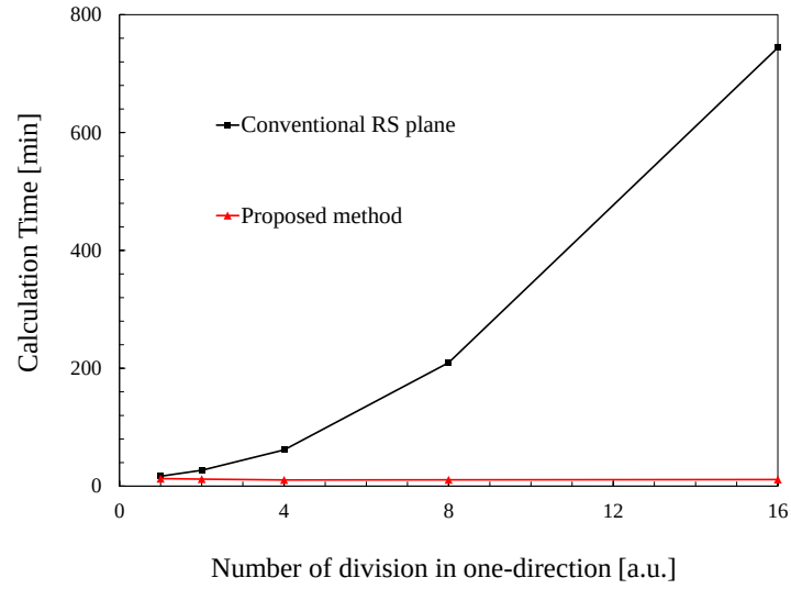
図 4.6 従来の RS 面と ORS 面における分割計算時間の比較結果
