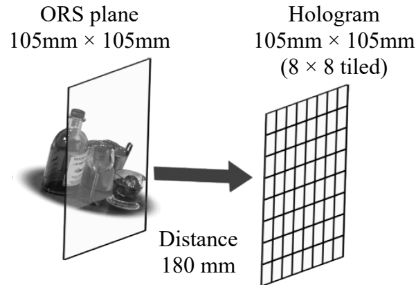
図 4.10 ウィスキー CGH の計算における物体と CGH の位置関係
