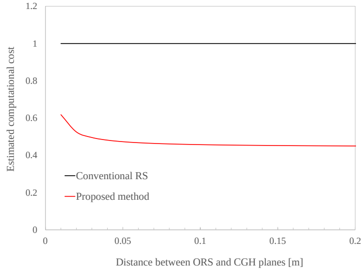
図 3.5 伝搬距離に対する従来手法と提案手法における計算量の推定
