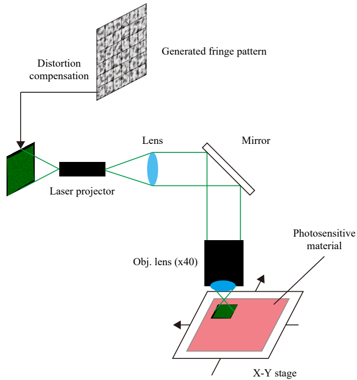
図 3.13 レーザープロジェクタと対物レンズを用いた CGH プリンタの光学系図
