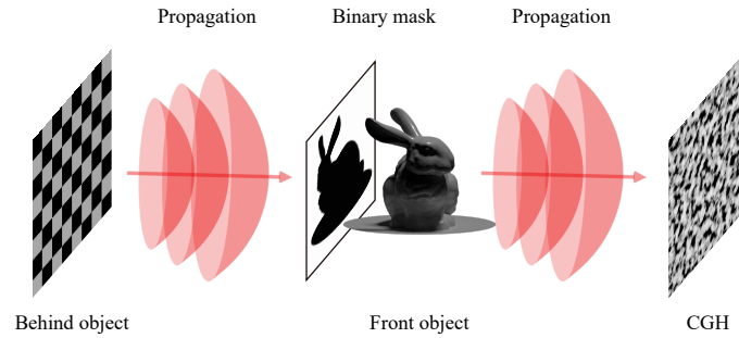
図 5.2 シルエット法を用いた相互オクルージョン処理
