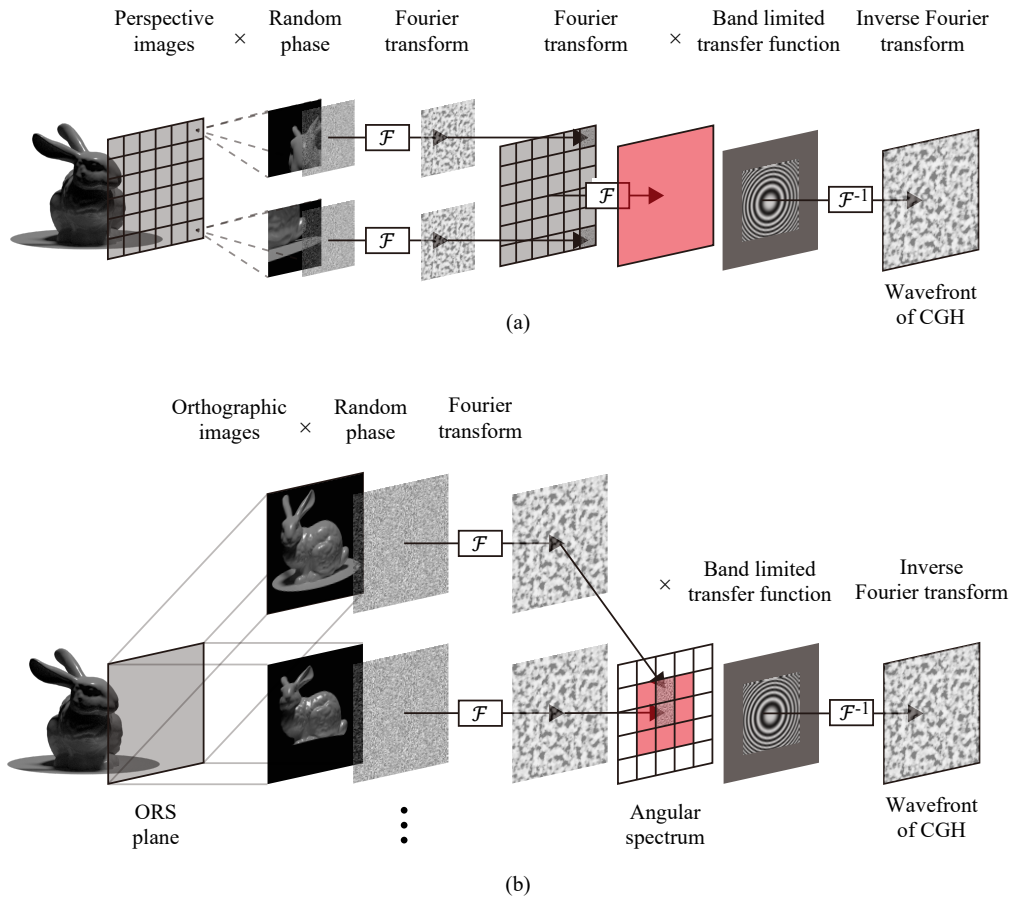
図 3.3 (a) 従来の RS 面を用いた CGH 計算法と (b) 正射影光線-波面変換を用いた CGH 計算法の比較
