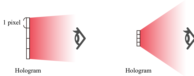
図 2.2 ディスプレイサイズとピクセルピッチの関係
