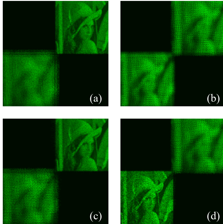
図 6.4 再生シミュレーション結果．通常の ORS 面を用いた CGH から再生し (a) 手前 (b) 奥にピントを合わせた像と，深度可変法を用いた CGH から再生し (c) 手前 (d) 奥にピントを合わせた像．
