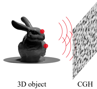
図 2.3 点光源法に基づく CGH 計算法の概念図
