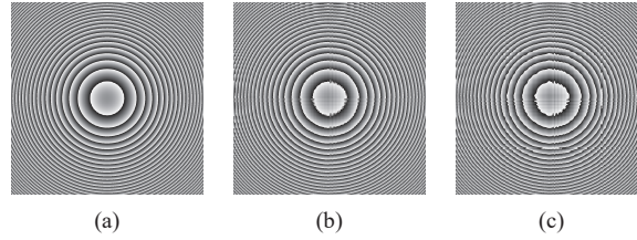
図 7.1 帯域制限フレネル伝搬によって計算された位相. (a) タイリングなし, (b) 2 \times 2 タイリング, (c) 4 \times 4 タイリング.
