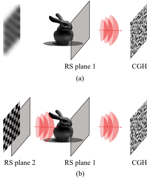
図 5.4 (a) 単一の RS 面による深度の限界と (b) 複数 ORS 面の設置による広深度表現
