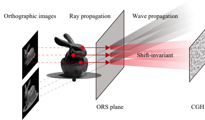
図 3.2 正射影光線-波面変換を用いた CGH 計算法の物理的イメージ
