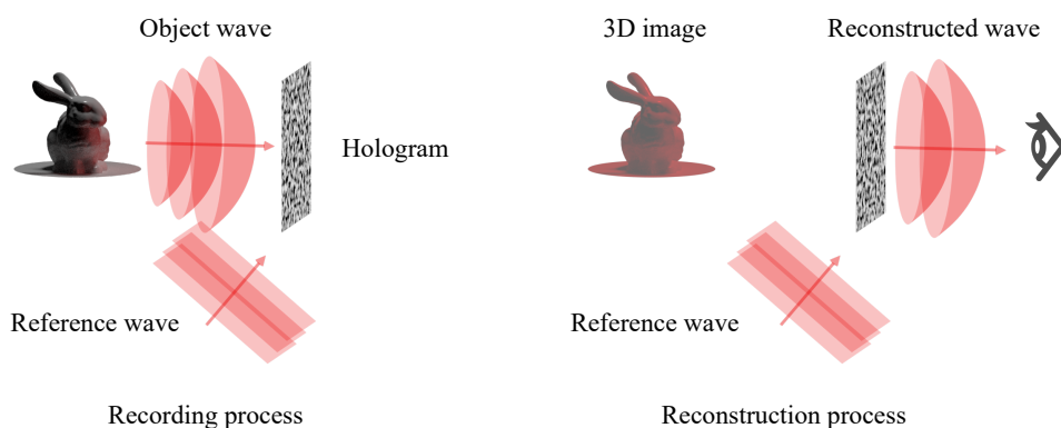
図 2.1 ホログラムの記録と再生の概念図
