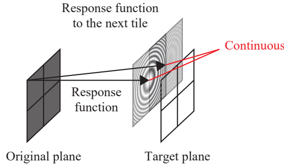
図 7.2 アーティファクトノイズを生じない分割伝搬計算の原理
