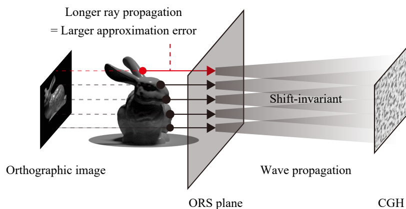
図 6.1 正射影光線-波面変換法における幾何光学近似に伴う精度低下の原因
