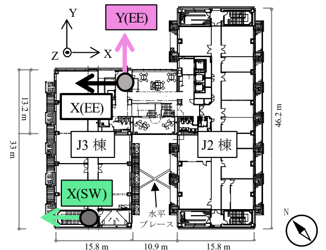
図3 J3 棟20階加速度計設置位置
