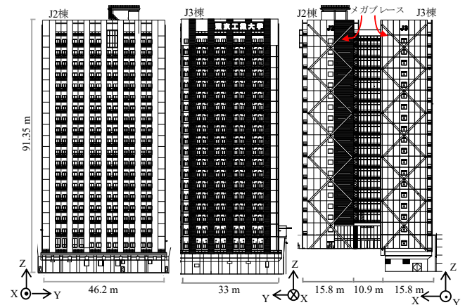
図2 J2-3 棟立面図
