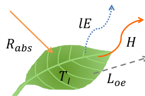
図 2-1 葉の熱収支
