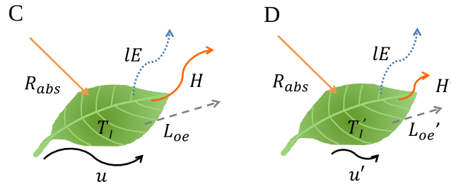
図 2-5 放射吸収量の変化が顕著な 2 時刻の葉の熱収支
