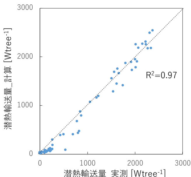
図 3-7 潜熱輸送量の熱収支モデルによる計算結果と実測結果の関係
