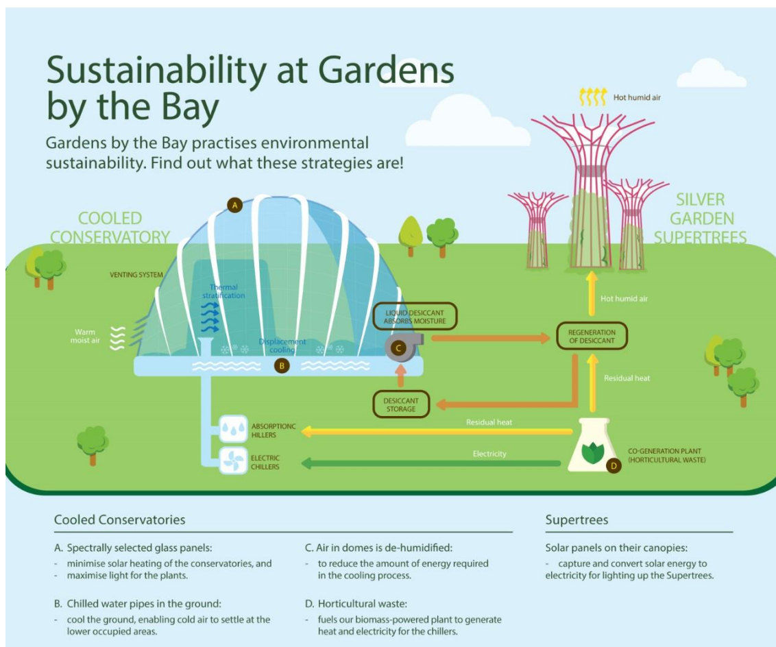
図-15 ガーデン・バイ・ザ・ベイ コージェネレーション設備概略図
