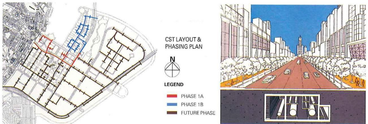
図-18 マリーナ・ベイエリア内の地中配管図及びイメージ
