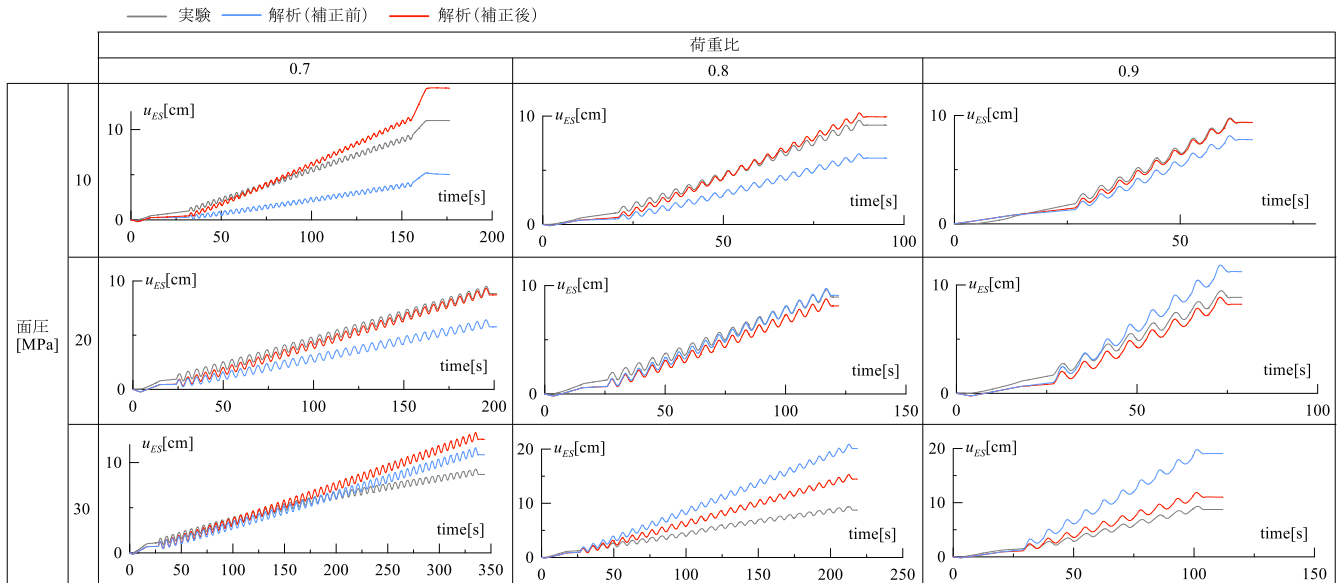
(b) 総厚 8 mm
